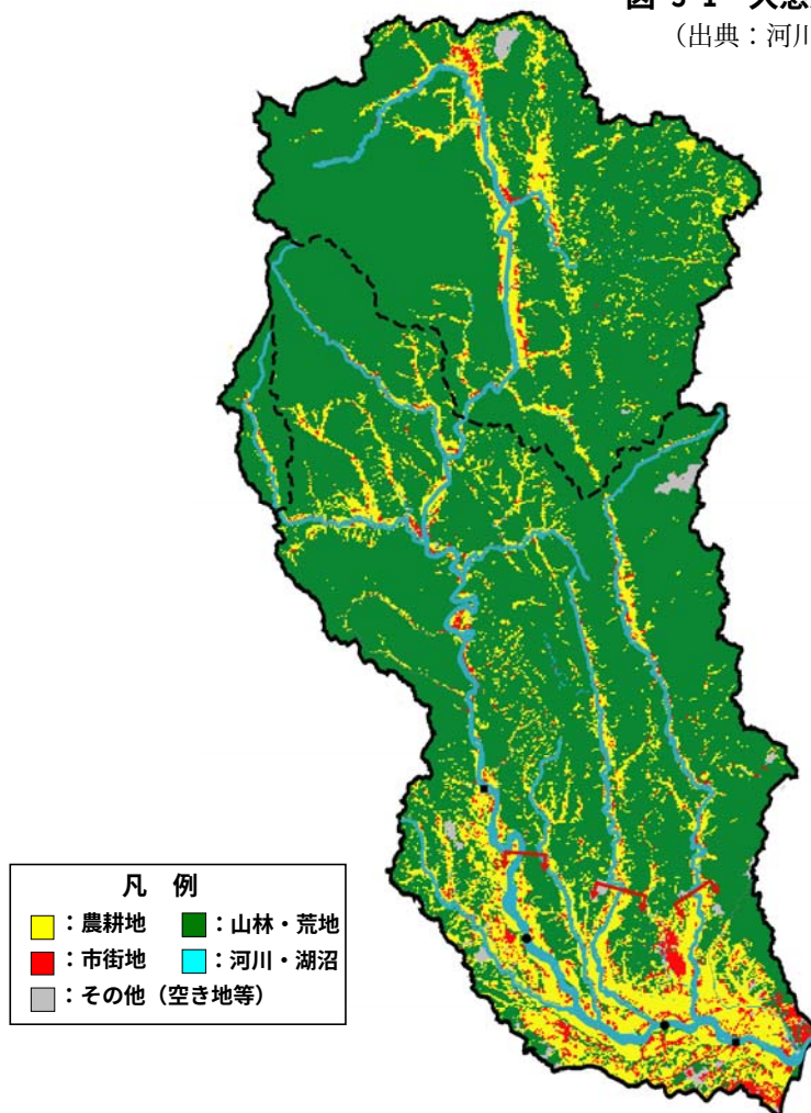
図 3-2 久慈川流域の土地利用状況図（平成 9 年）
