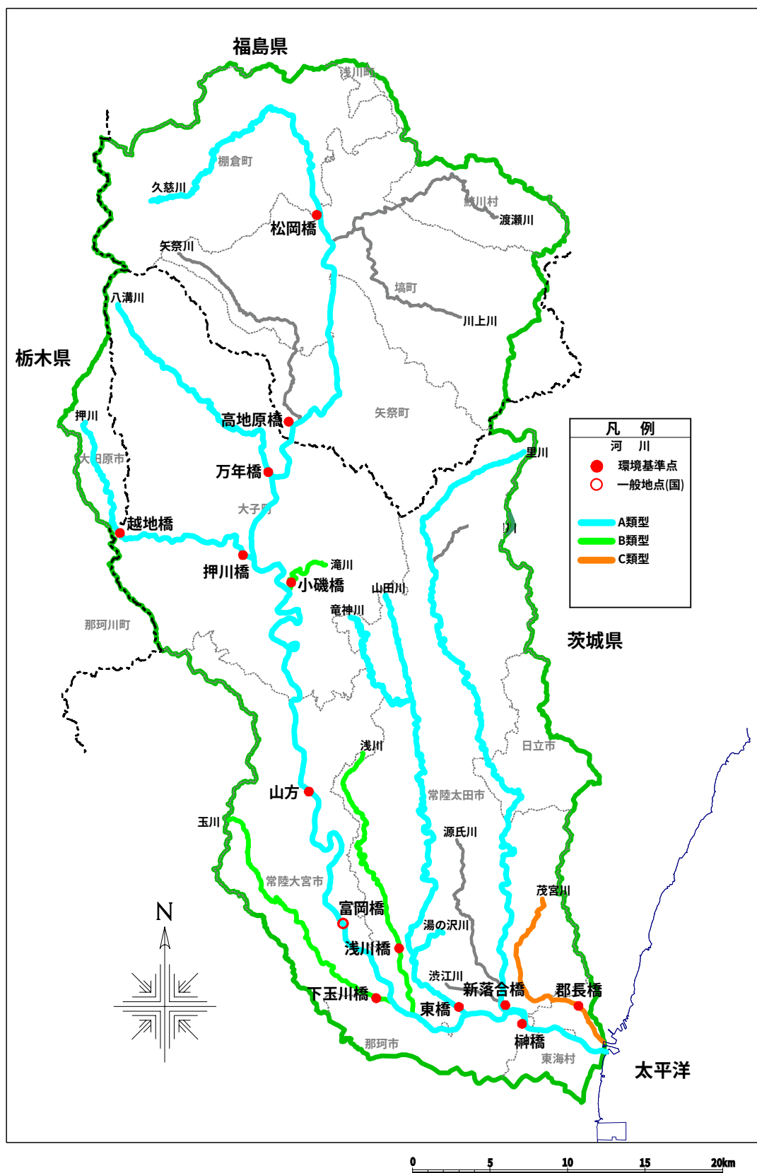
図 6-2 久慈川流域の環境基準類型指定図
