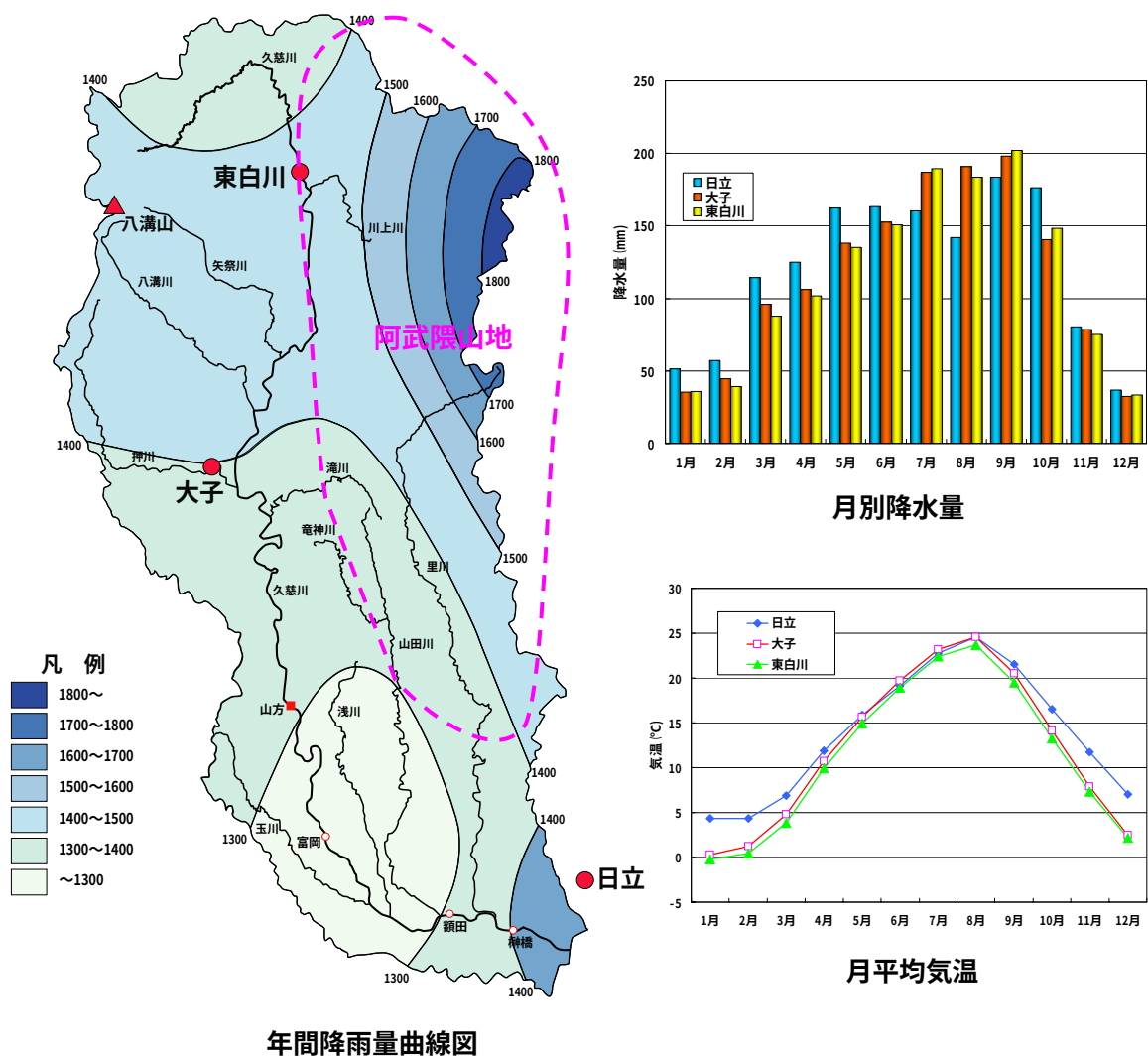
図 1-4 久慈川流域の気象（昭和 52 年～平成 18 年 30 カ年平均）
