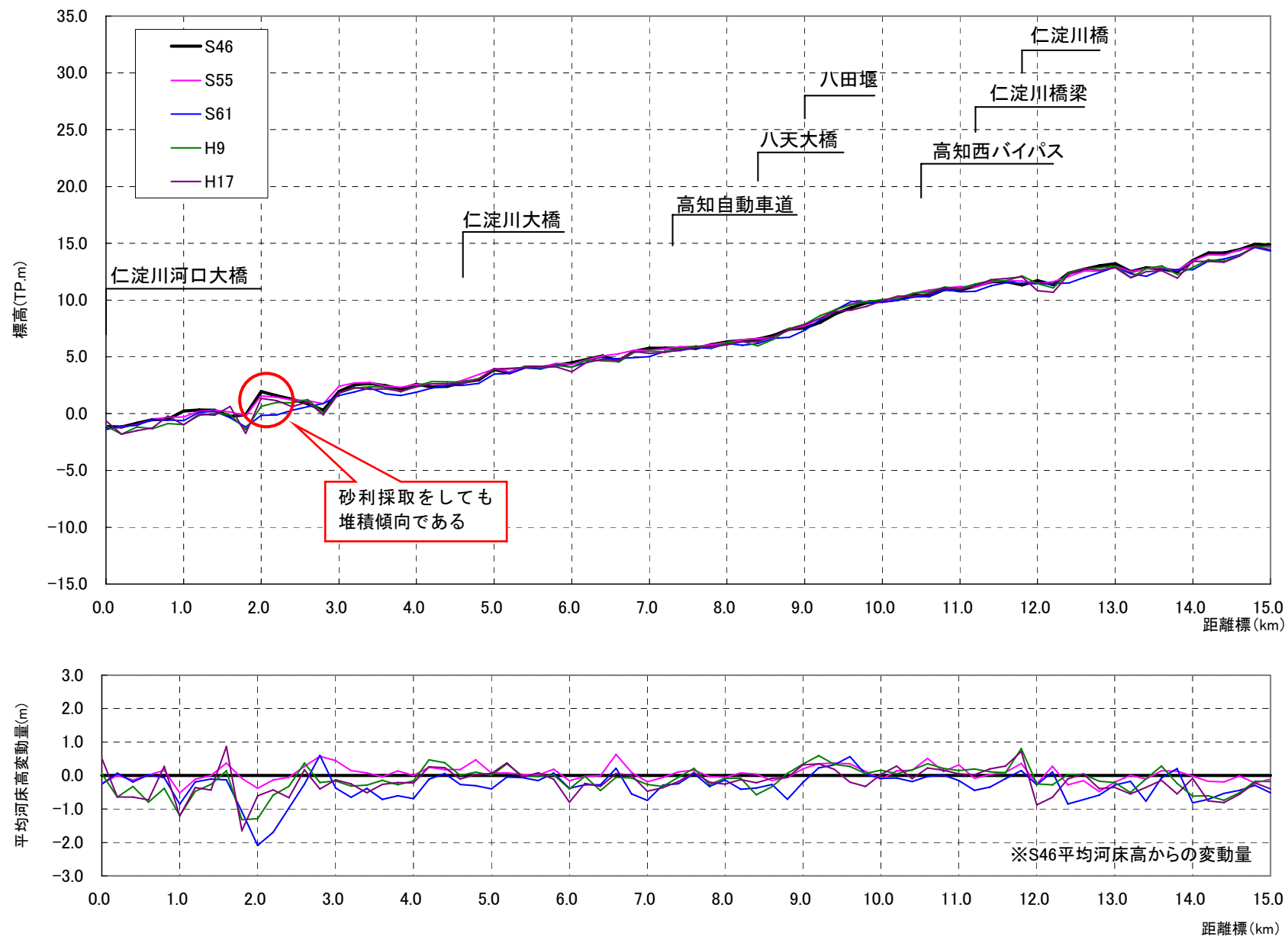
図 2 - 3 仁淀川平均河床高縦断図 (上段)、昭和46年を基準とした平均河床高変動量 (下段)
