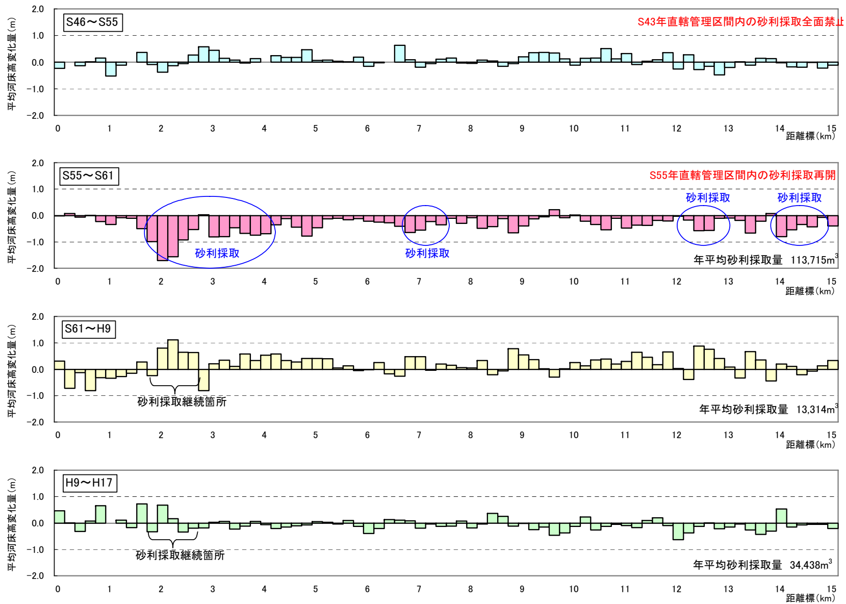
図 2 - 2 年平均河床変動高
