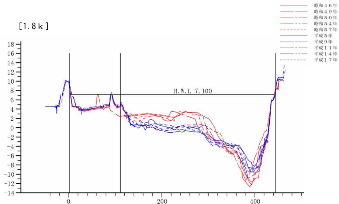
図2-4 (1) 仁淀川1.8k横断図
