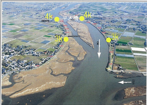
② 緑川浜戸川合流点付近 (3k~4k付近)
