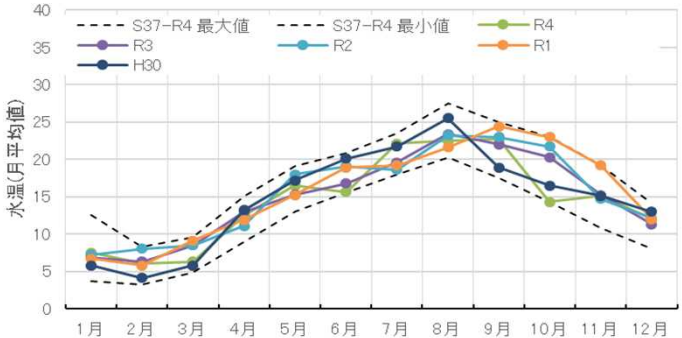
水温(鹿島橋)の経月変化
