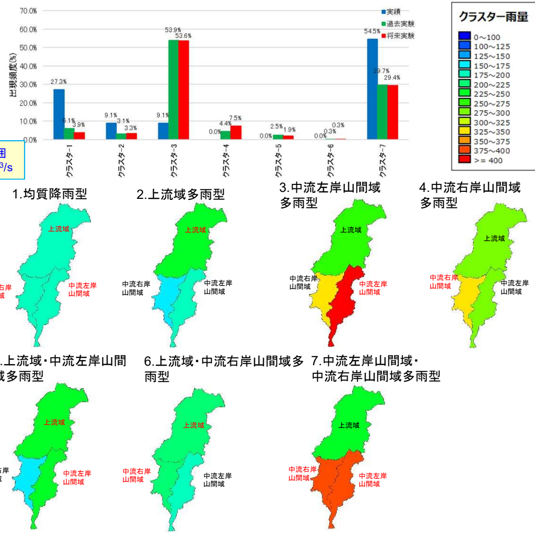
降雨寄与率の分析による主要洪水群に不足する地域分布の降雨パターンの確認
