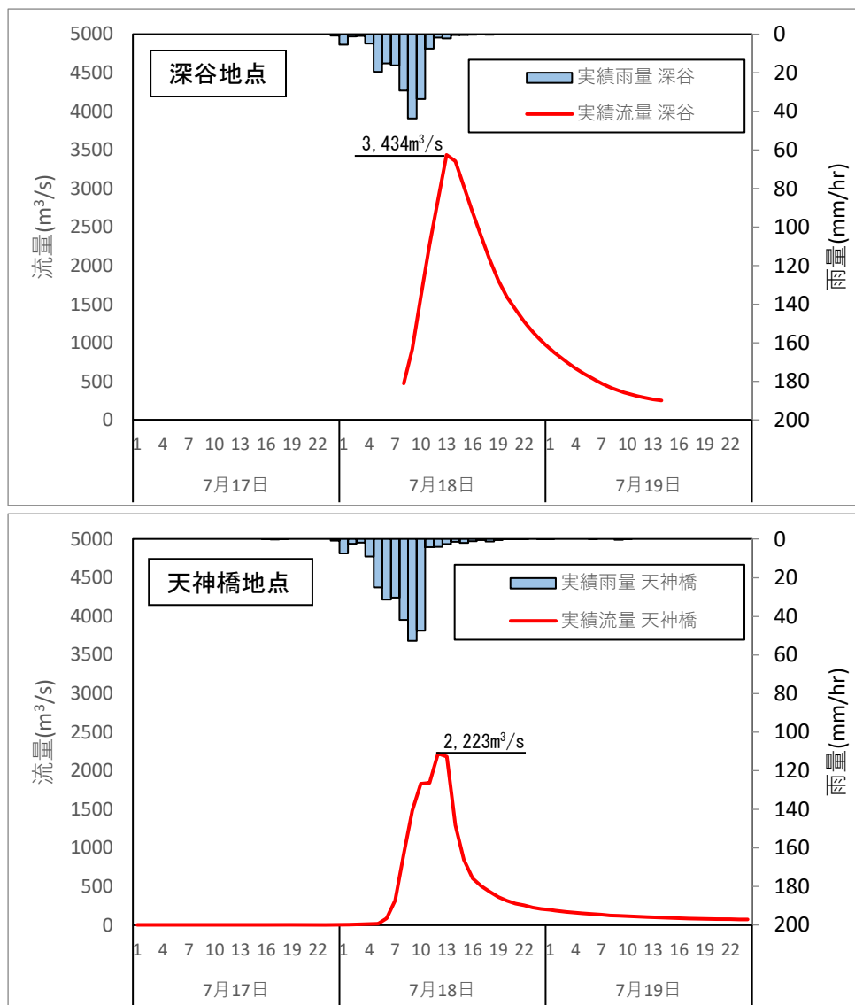
図 1.67 平成 16 年 7 月洪水のハイドログラフ（実績流量）
