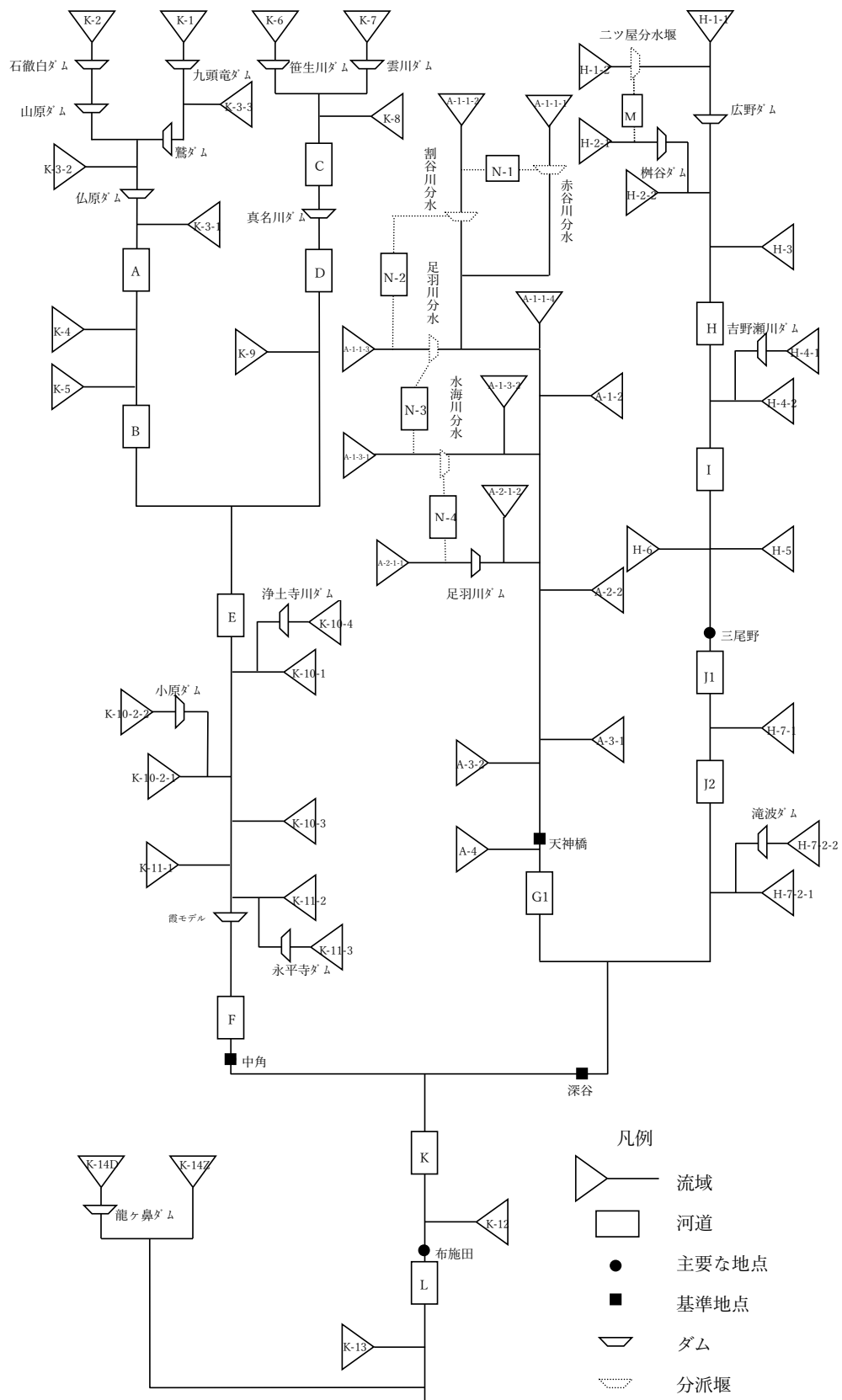
図 1.8 流出モデル模式図
