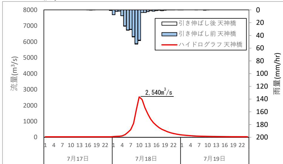
図 1.55 (3) 基本高水ハイドロ (基準地点：天神橋地点)
