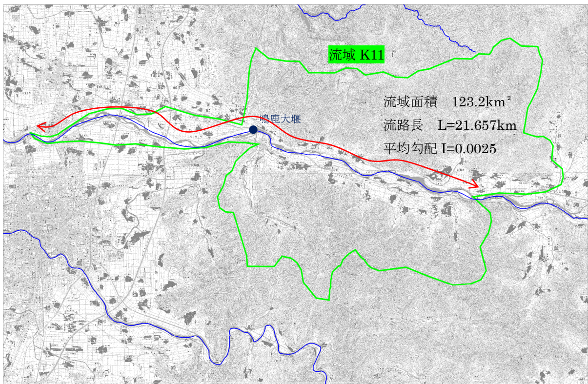
图 1.17 (11) 流路延長 (流域番号 K11)
