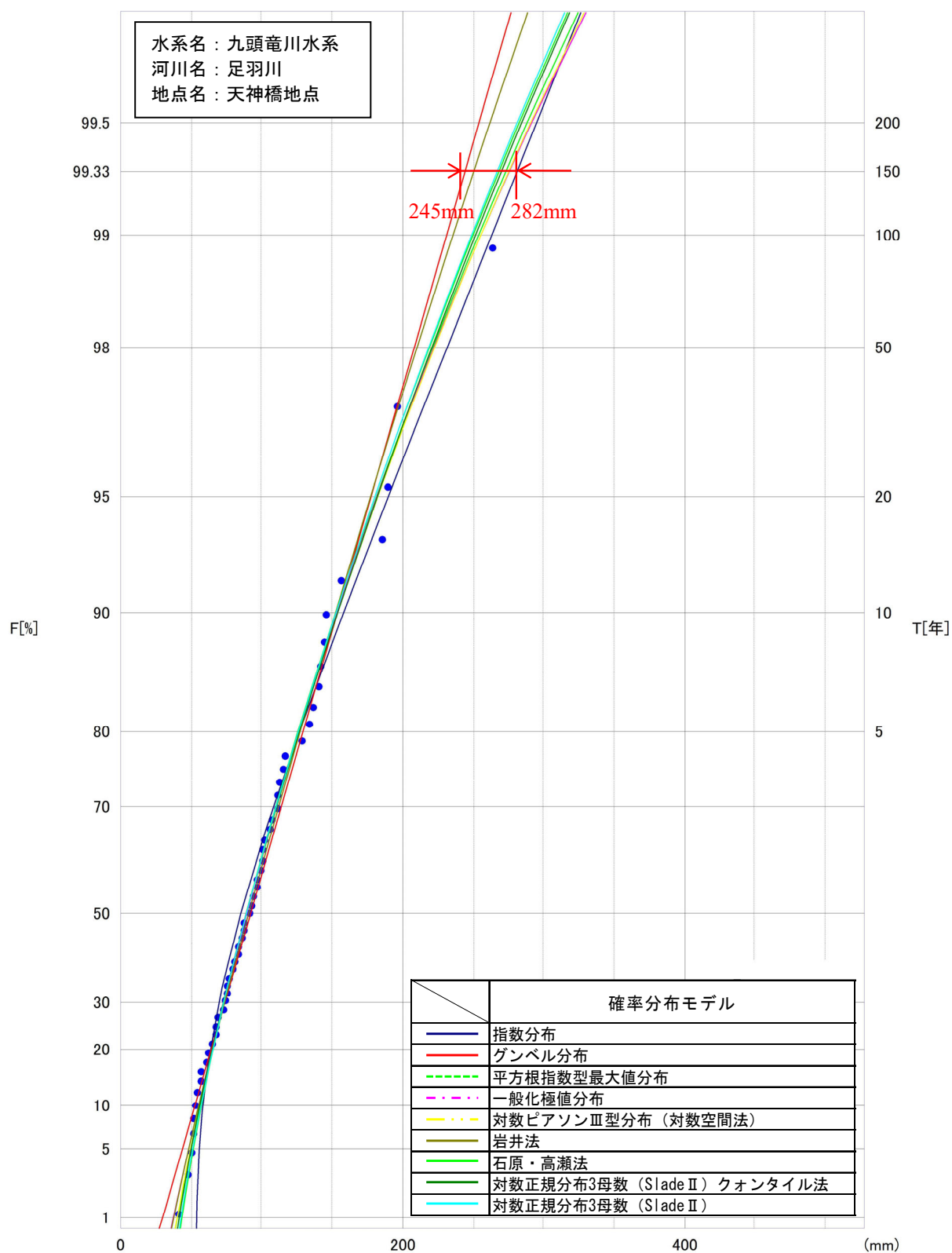
図 1.47 天神橋地点における雨量確率計算結果
