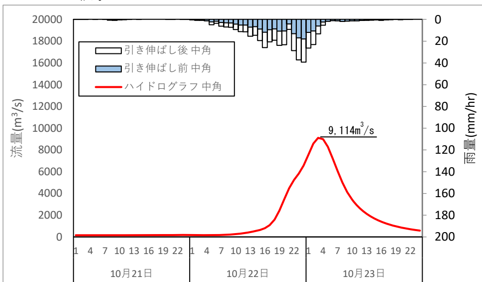
図 1.53 (2) 基本高水ハイドロ (基準地点：中角地点)
