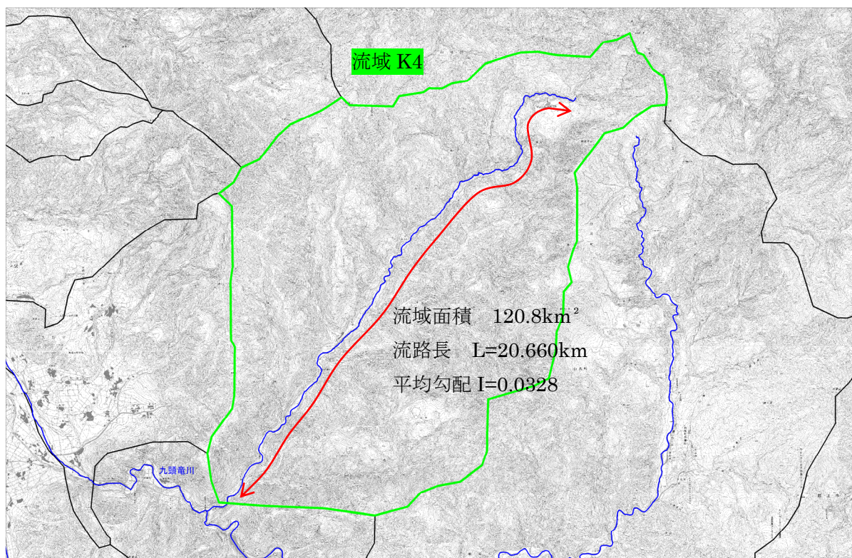
图 1.17 (4) 流路延長 (流域番号 K4)
