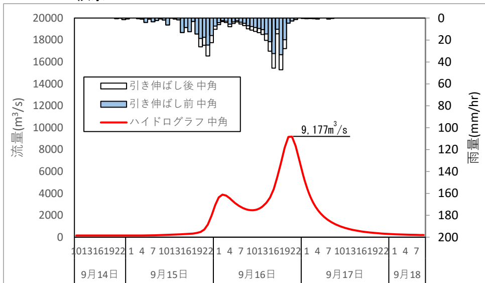
図 1.53 (1) 基本高水ハイドロ (基準地点：中角地点)
