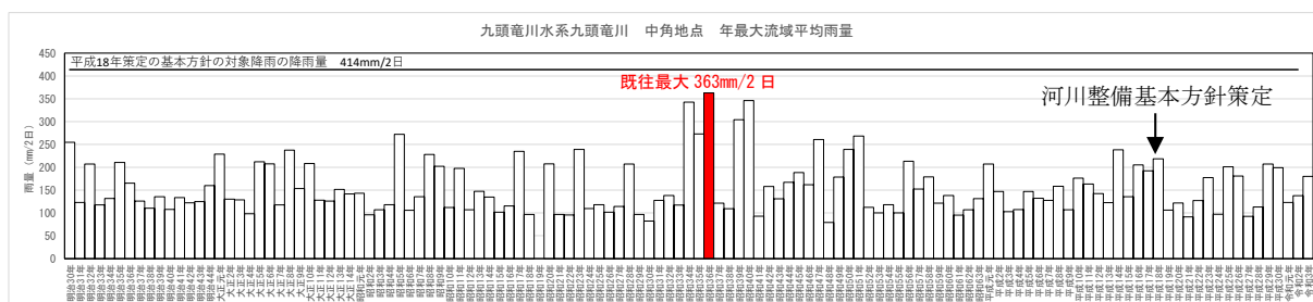
図 1.2 年最大 2 日雨量（基準地点中角上流域平均雨量）
