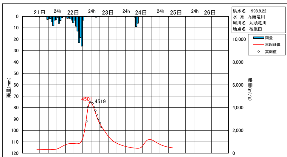
図 1.30 H10.9.22 洪水ハイドロの再現計算結果 (1/2)
