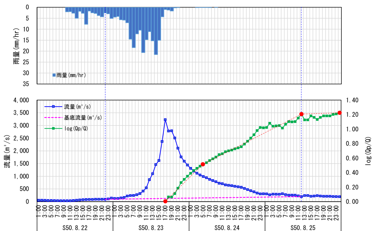
图 1.11 (1) 流出成分分離結果 (中角 S50.8.23)
