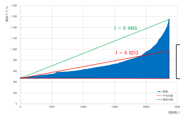
図 1.14 流域平均勾配算出例（流域番号 K2）
