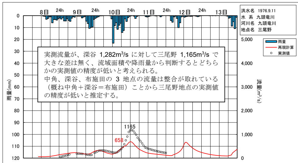
図 1.29 S51.9.11 洪水ハイドロの再現計算結果 (2/2)
