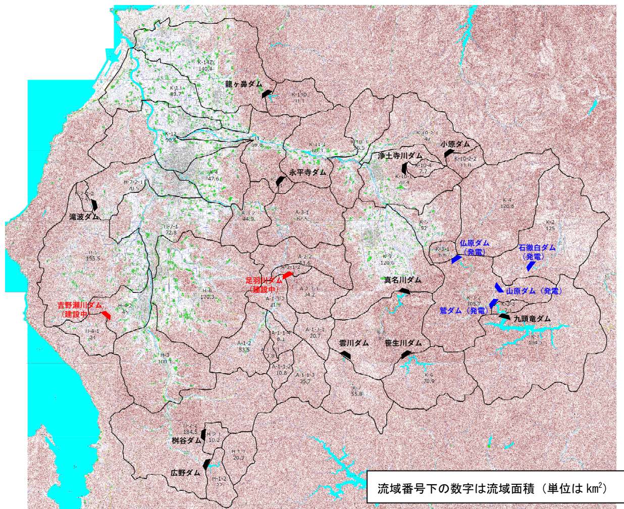
図 1.7 流域分割図
