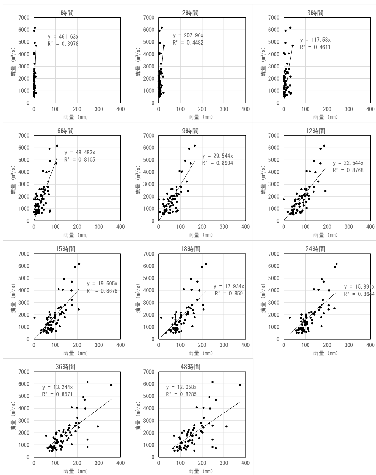
図 1.39 ピーク流量と雨量の相関関係（中角地点）
