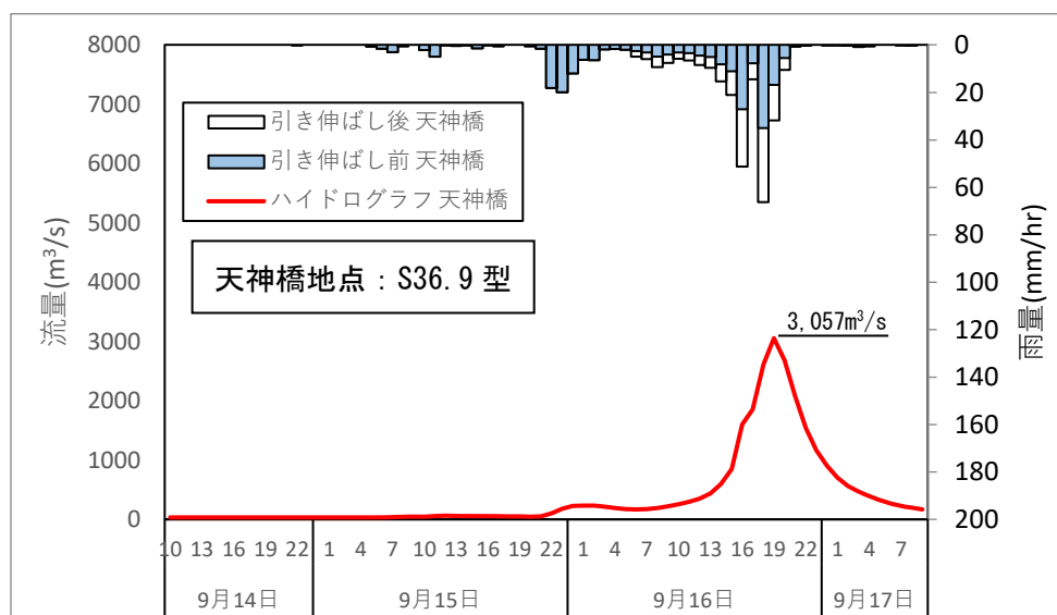
図 1.71 基本高水のピーク流量決定のハイドログラフ
