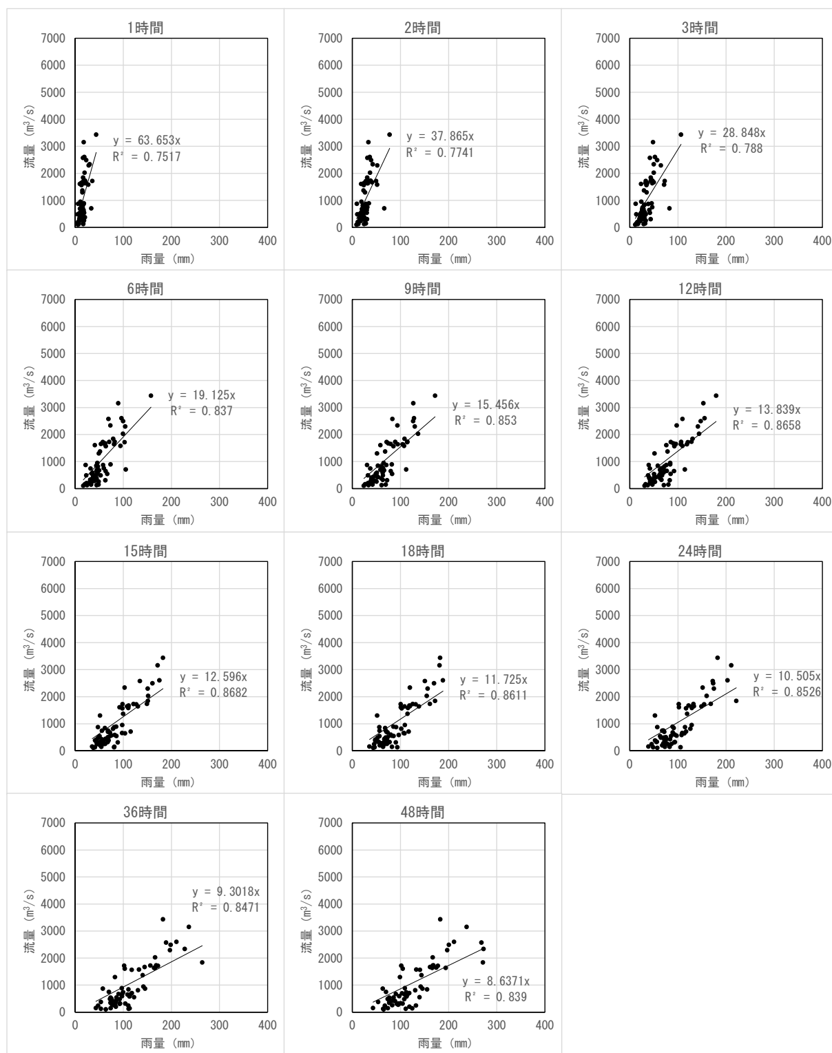
図 1.40 ピーク流量と雨量の相関関係（深谷地点）
