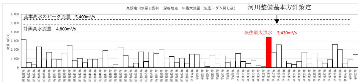
図 1.3 年最大流量（基準地点深谷）
