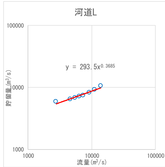
図 1.21 (3) S-Q 関係図 (計画河道)
