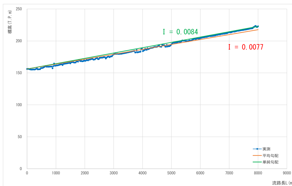
图 1.18 (5) 流域流路勾配 (流域番号 K5)
