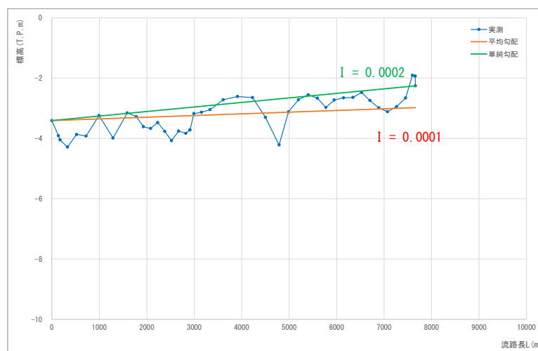
図 1.18 (13) 流域流路勾配 (流域番号 K13)
