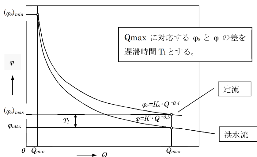
図 1.22 定流の貯留関数 \varphi_s と洪水流の貯留関数 \varphi の関係
