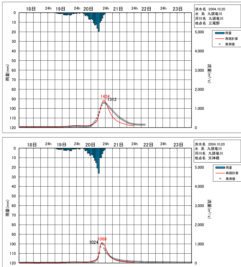
図 1.35 H16. 10. 20 洪水ハイドロの再現計算結果 (2/2)
