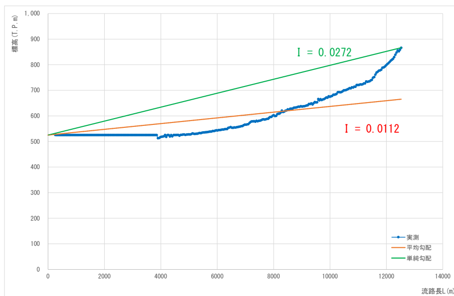
図 1.18 (6) 流域流路勾配 (流域番号 K6)
