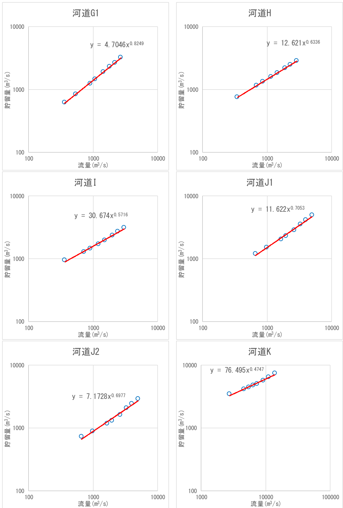
図 1.21 (2) S-Q 関係図 (計画河道)
