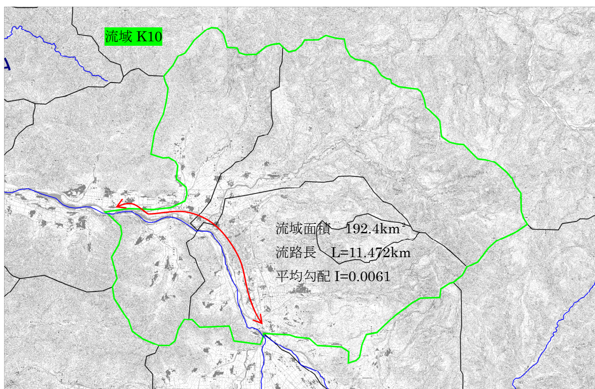
図 1.17 (10) 流路延長 (流域番号 K10)
