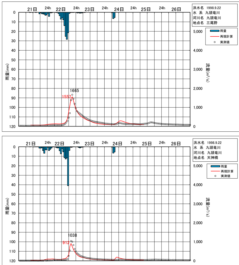
図 1.31 H10. 9. 22 洪水ハイドロの再現計算結果 (2/2)
