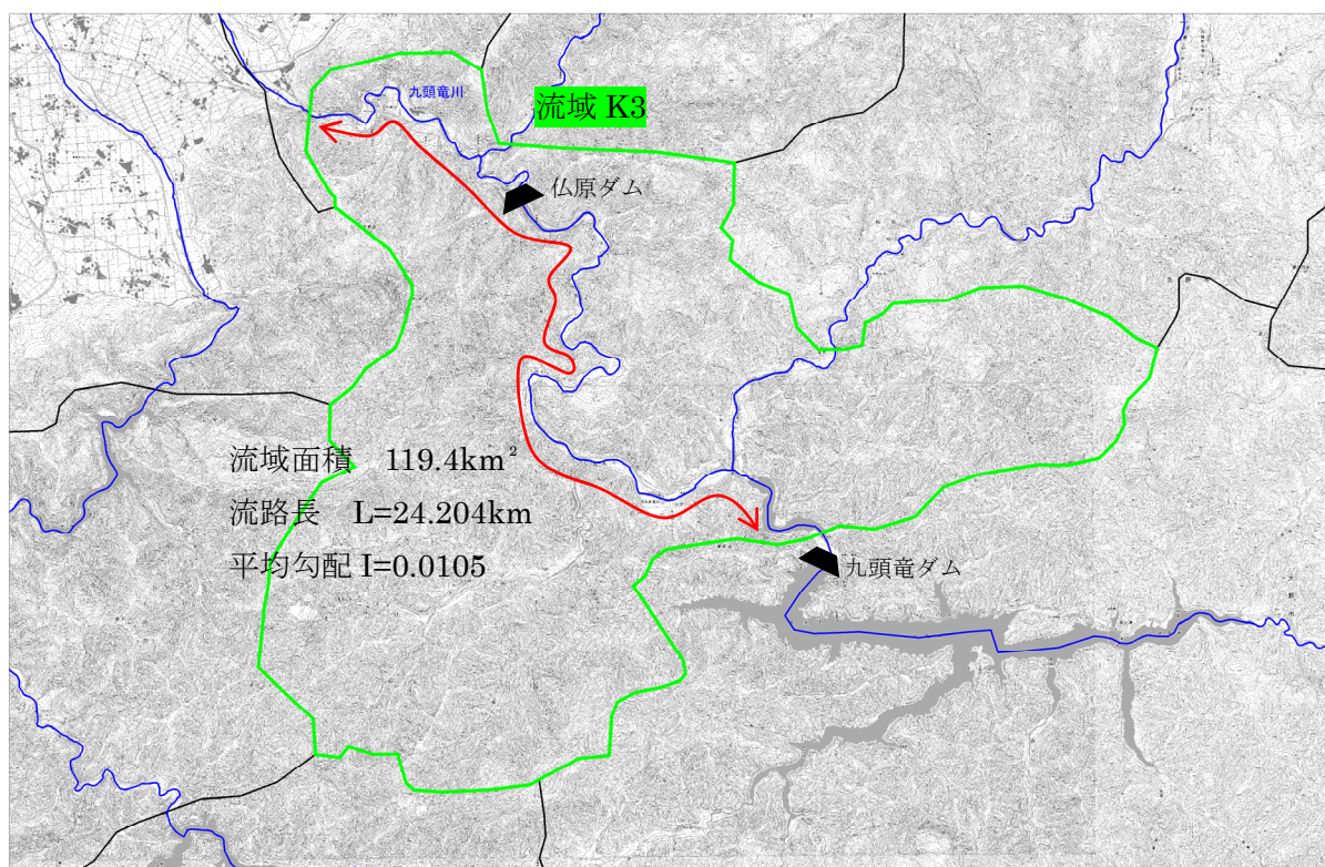
図 1.17 (3) 流路延長 (流域番号 K3)
