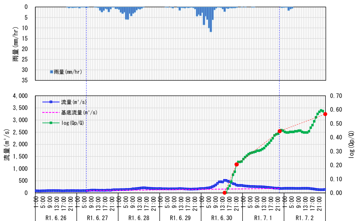
図 1.11 (13) 流出成分分離結果 (中角 R1. 6. 30)
