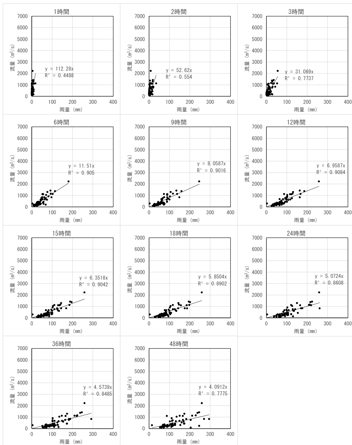
図 1.43 ピーク流量と雨量の相関関係（天神橋地点）
