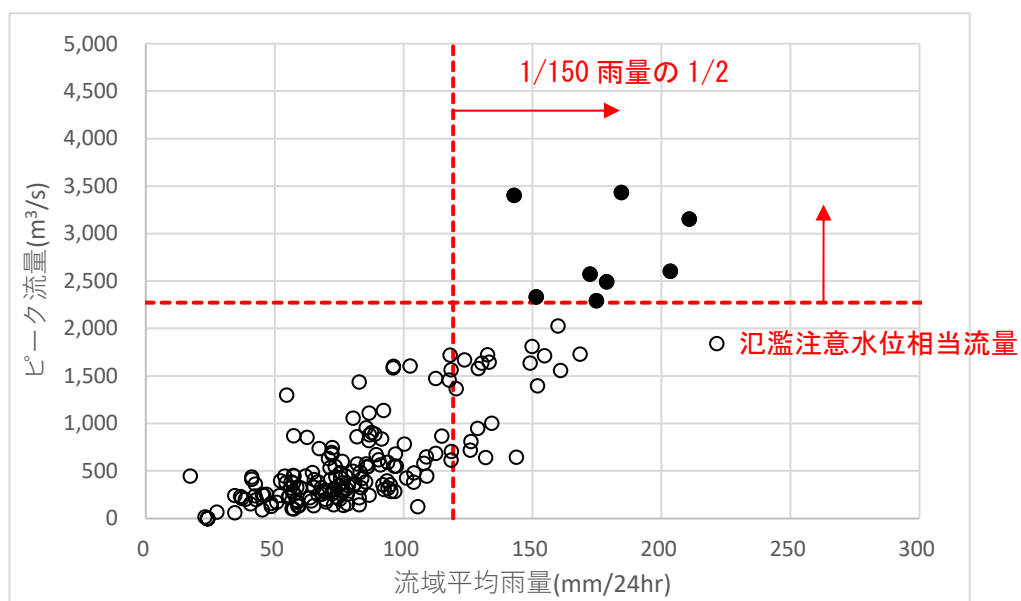
図 1.49 対象洪水の選定結果（基準地点：深谷地点）
