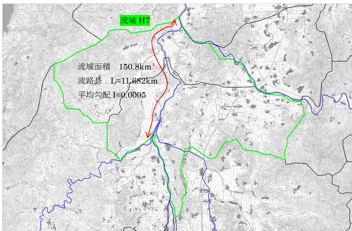
图 1.17 (26) 流路延長 (流域番号 H7)
