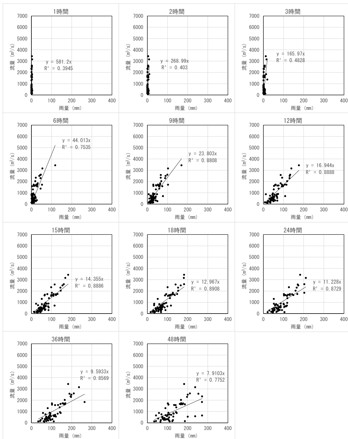
図 1.41 ピーク流量と雨量の相関関係（深谷地点）
