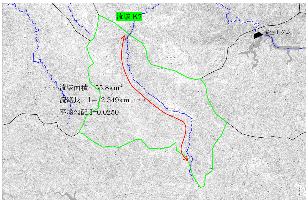
図 1.17 (7) 流路延長 (流域番号 K7)
