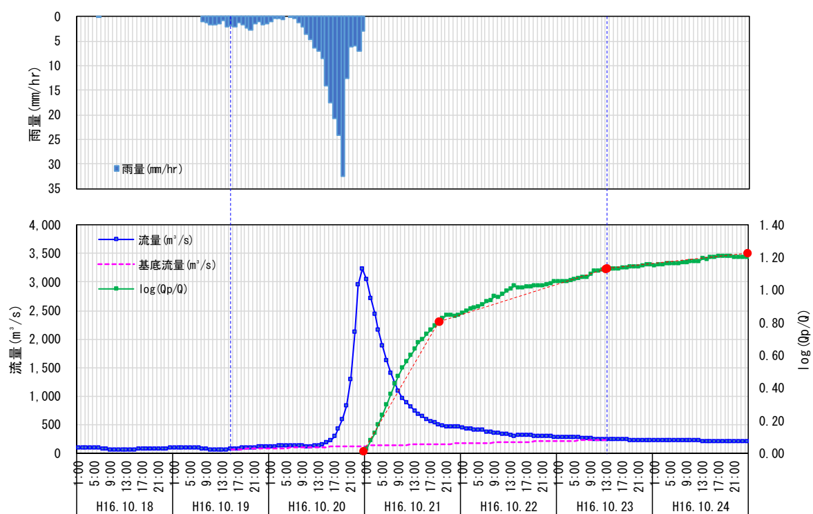
图 1.11 (4) 流出成分分離結果 (中角 H16.10.20)
