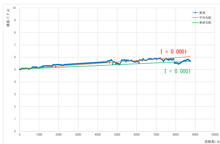
図 1.18 (12) 流域流路勾配 (流域番号 K12)
