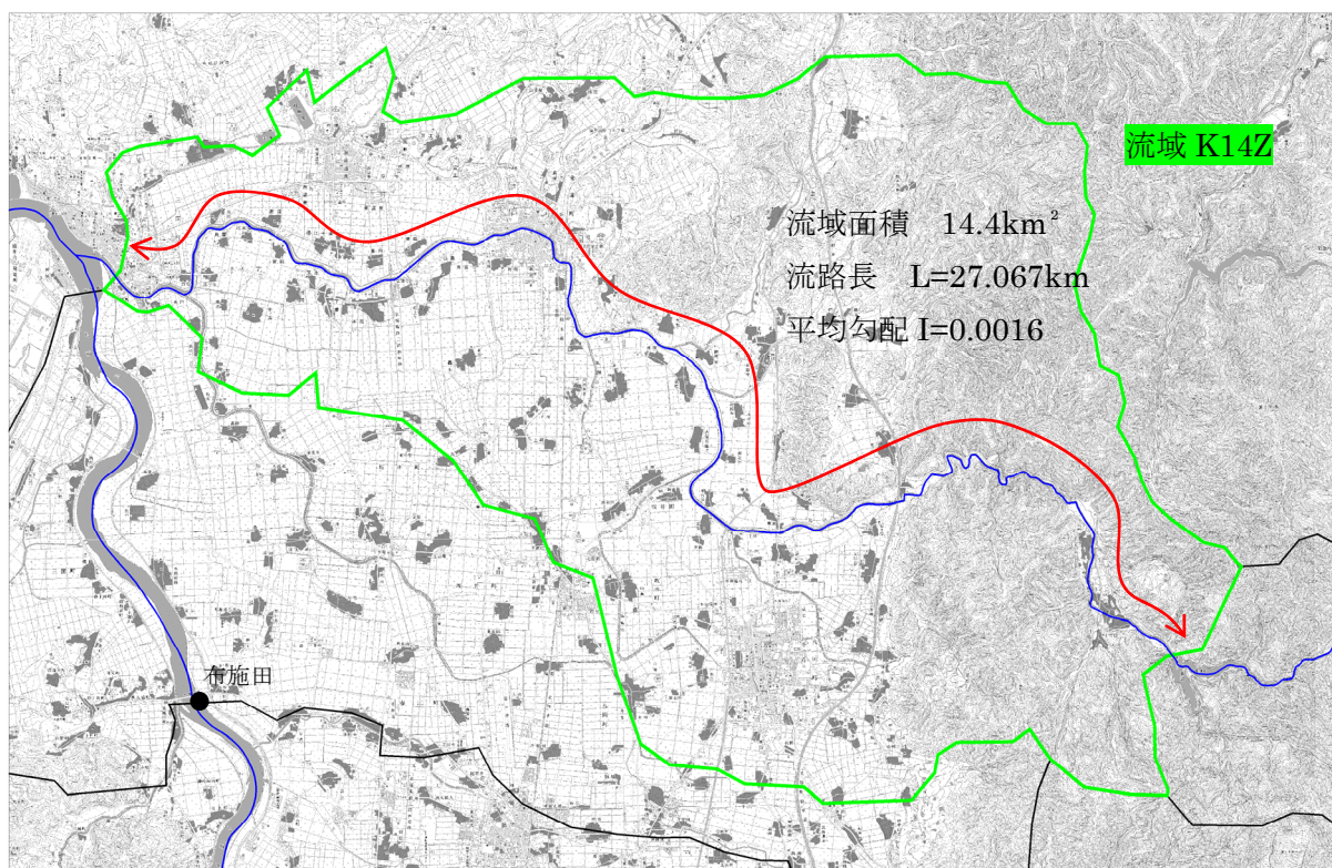
图 1.17 (15) 流路延長 (流域番号 K14Z)
