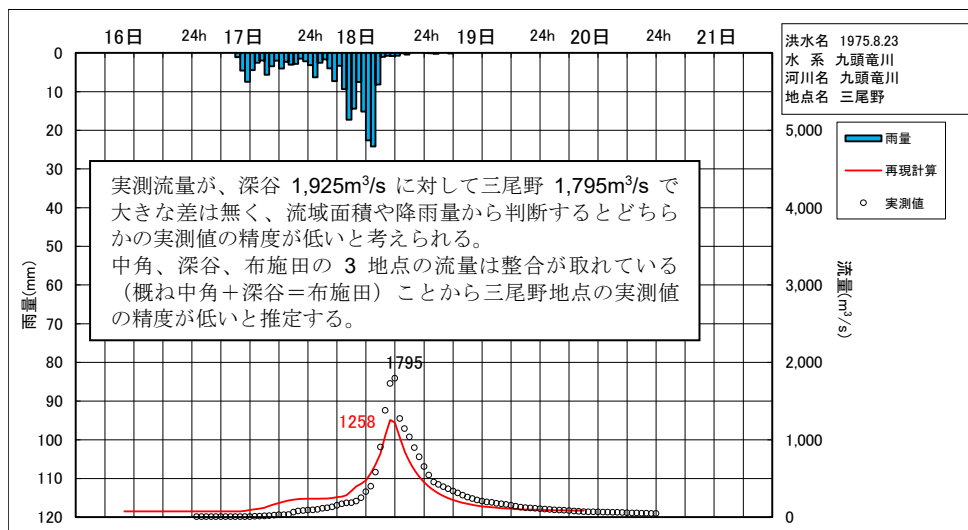
図 1.27 S50. 8. 23 洪水ハイドロの再現計算結果 (2/2)
