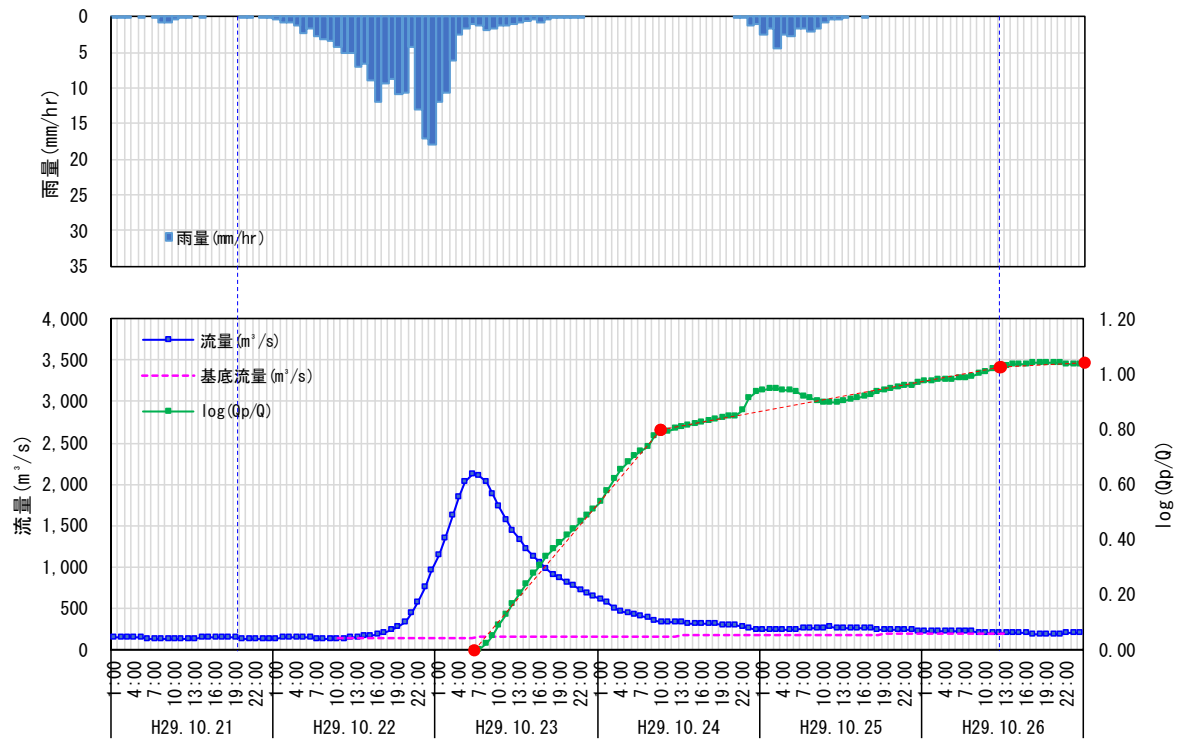
图 1.11 (11) 流出成分分離結果 (中角 H29.10.22)
