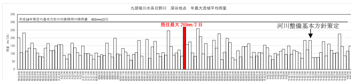
図 1.4 年最大2日雨量（基準地点深谷上流域平均雨量）
