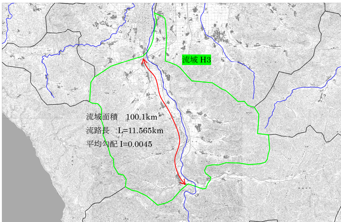
图 1.17 (22) 流路延長 (流域番号 H3)
