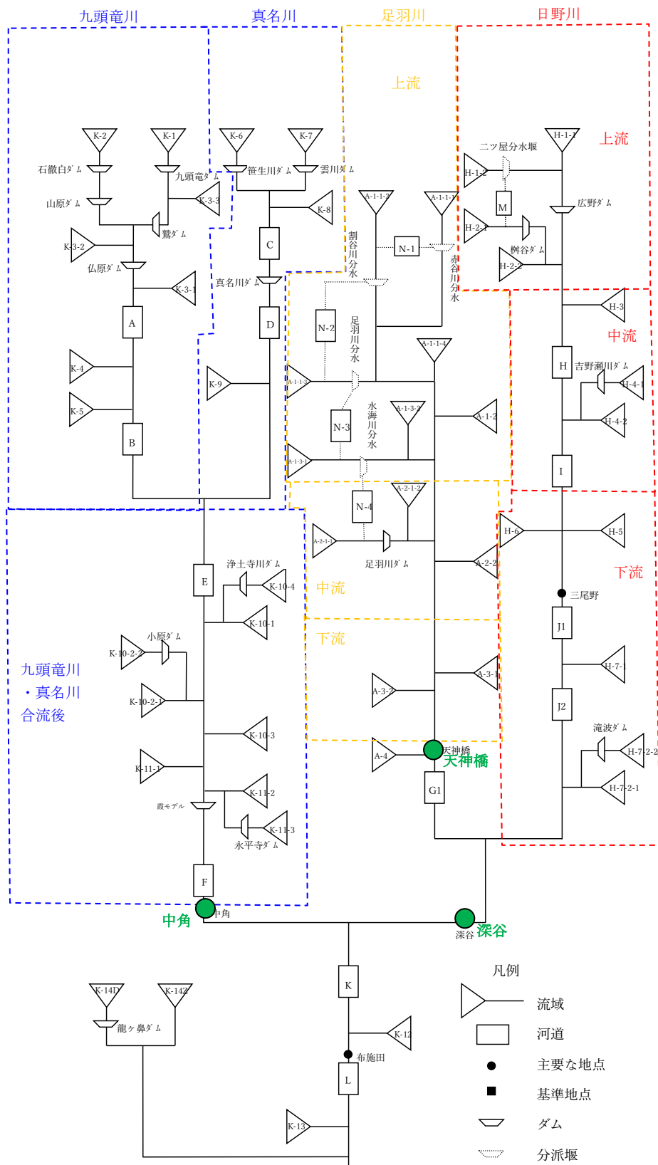
図 1.52 地域分布の検討地区（モデル図）
