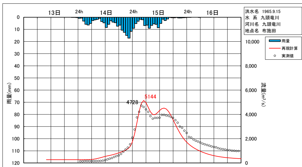
図 1.25 S40. 9. 15 洪水ハイドロの再現計算結果
