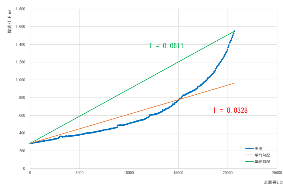
图 1.18 (4) 流域流路勾配 (流域番号 K4)
