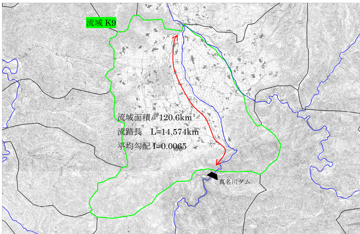
図 1.17 (9) 流路延長 (流域番号 K9)
