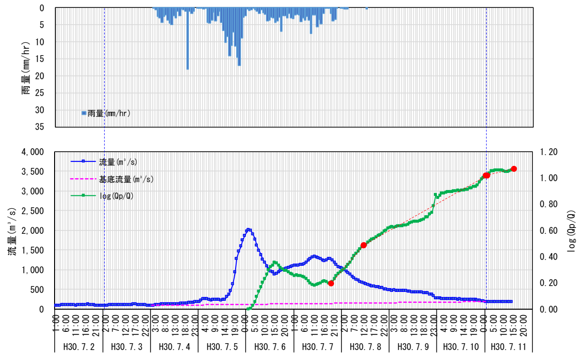
图 1.11 (12) 流出成分分離結果 (中角 H30.7.6)
