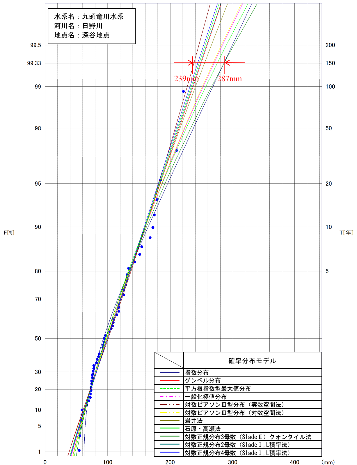
図 1.46 深谷地点における雨量確率計算結果
