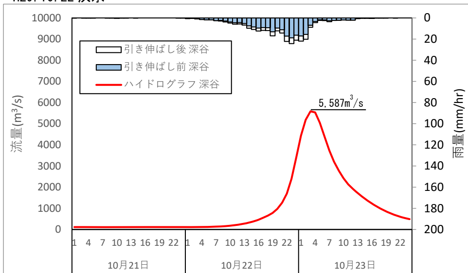
図 1.54 (2) 基本高水ハイドロ (基準地点 : 深谷地点)
