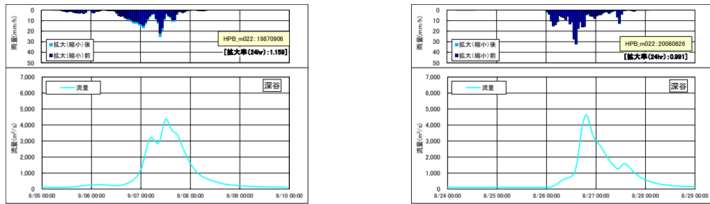
図 1.59 (3) 抽出した予測降雨波形群によるハイドログラフ (基準地点: 深谷地点)
