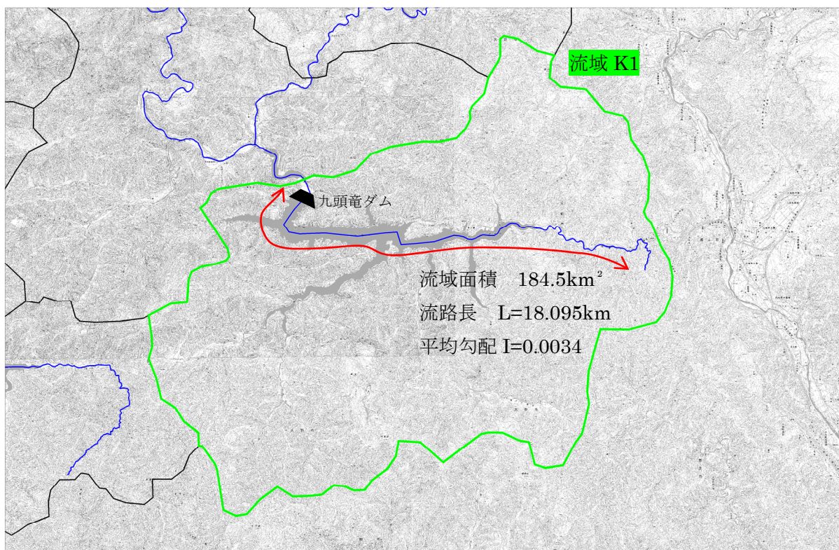
図 1.17 (1) 流路延長 (流域番号 K1)
