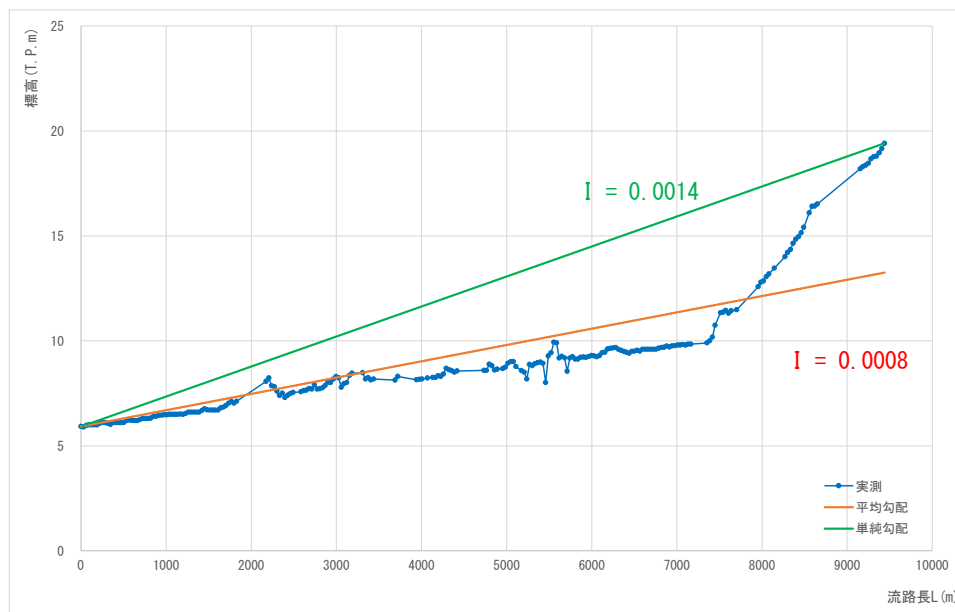
图 1.18 (19) 流域流路勾配 (流域番号 A4)
