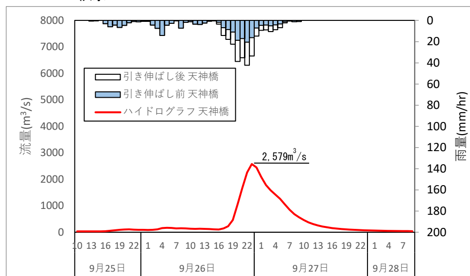
図 1.55 (1) 基本高水ハイドロ (基準地点：天神橋地点)
