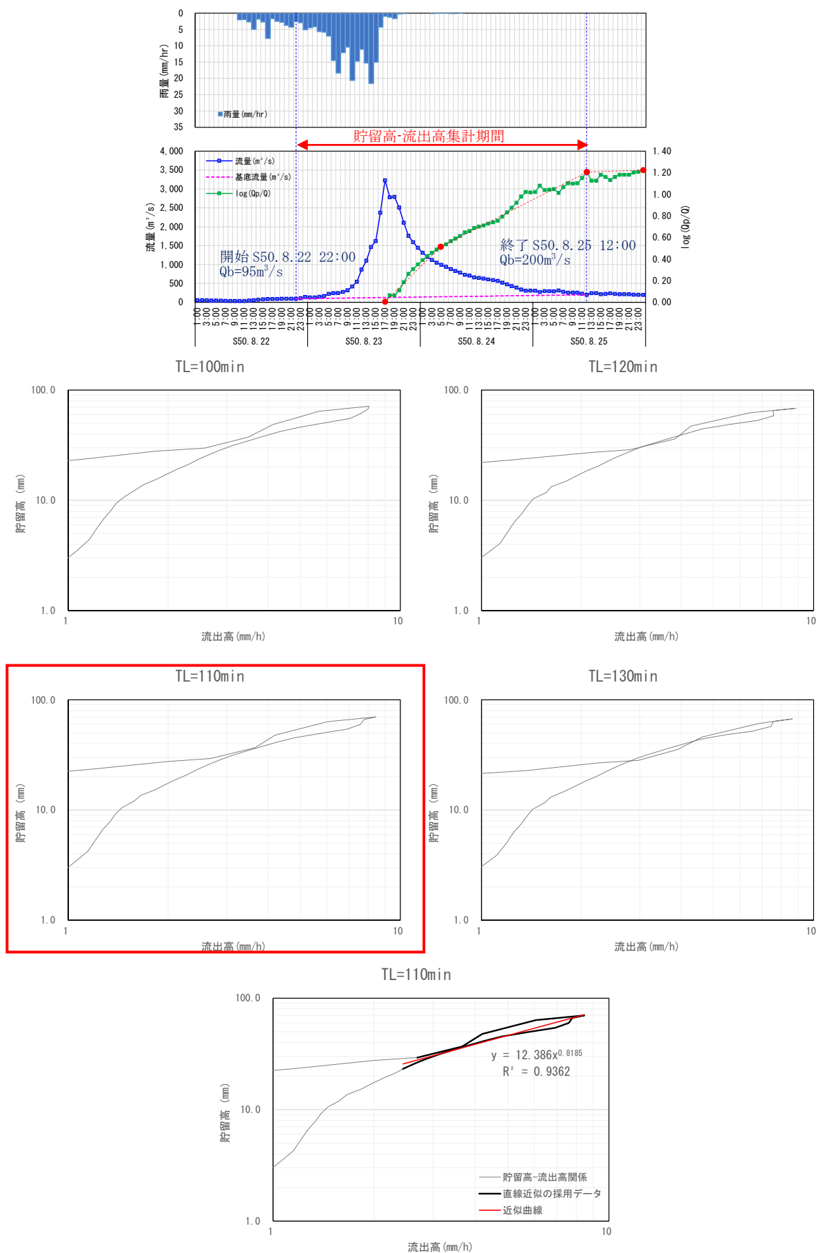
図 1.13 貯留高-流出高関係図 (中角地点 S50.8.23 洪水)
