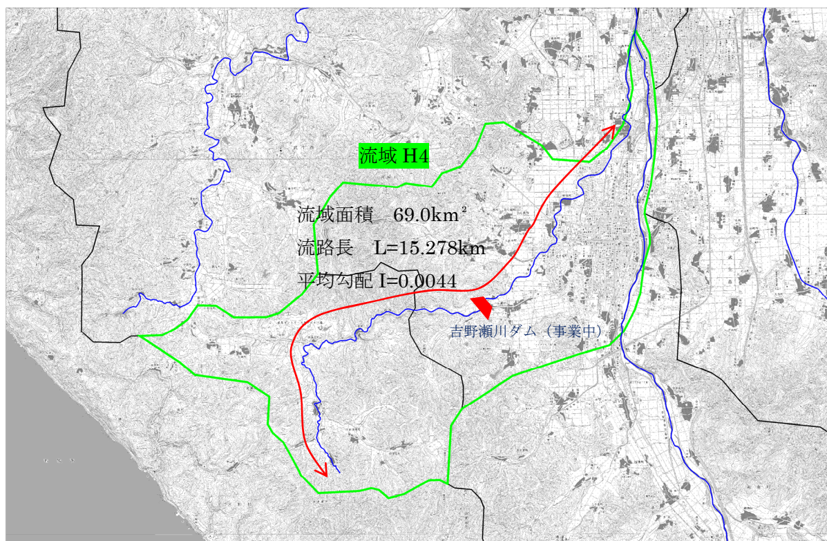
図 1.17 (24) 流路延長（流域番号 H4）
