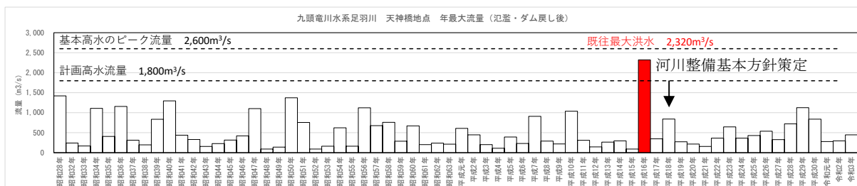
図 1.5 年最大流量（基準地点天神橋）
