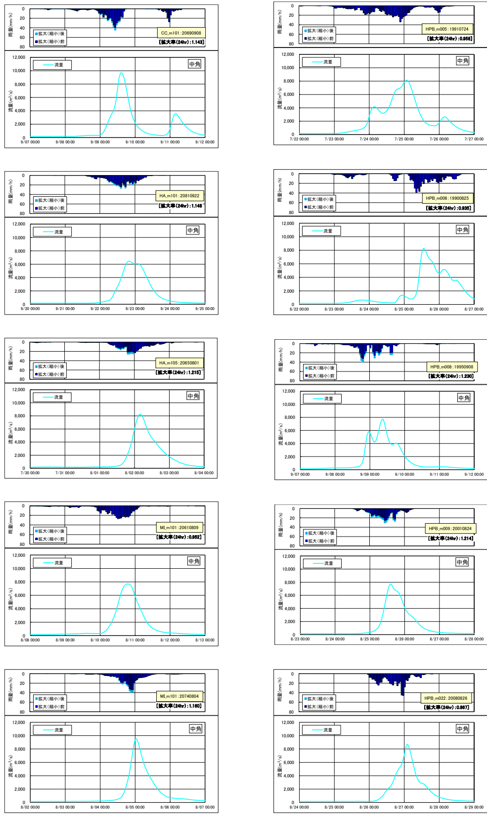
図 1.57 抽出した予測降雨波形群によるハイドログラフ（基準地点：中角地点）
