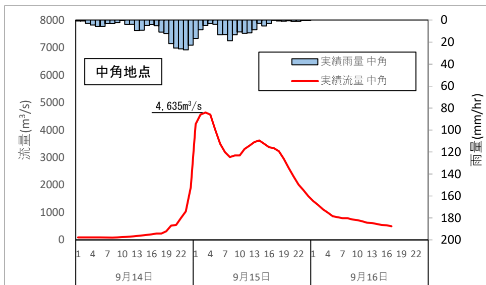
図 1.66 昭和 40 年 9 月洪水のハイドログラフ（実績流量）
