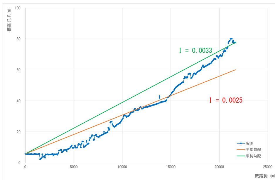
图 1.18 (11) 流域流路勾配 (流域番号 K11)
