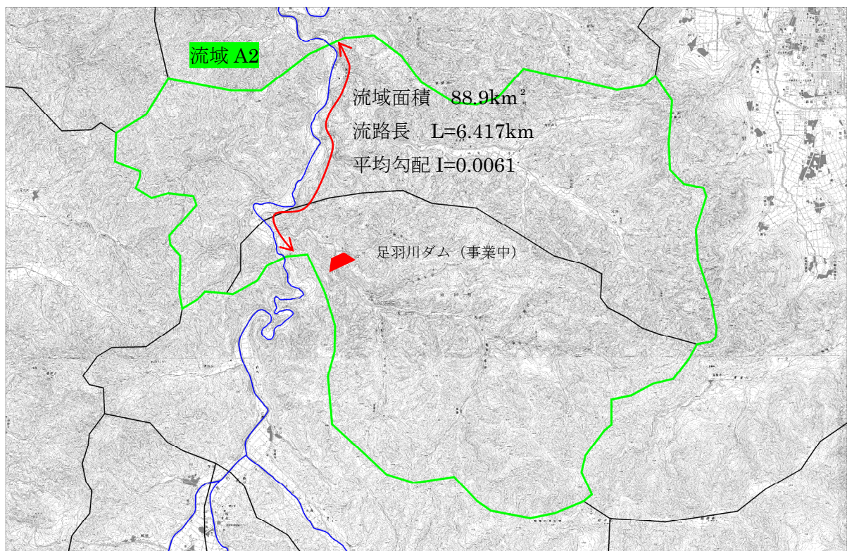
図 1.17 (17) 流路延長（流域番号 A2）
