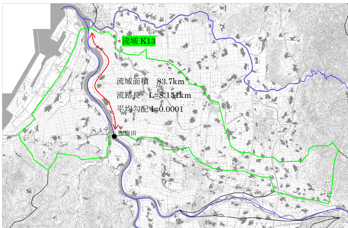
図 1.17 (13) 流路延長 (流域番号 K13)
