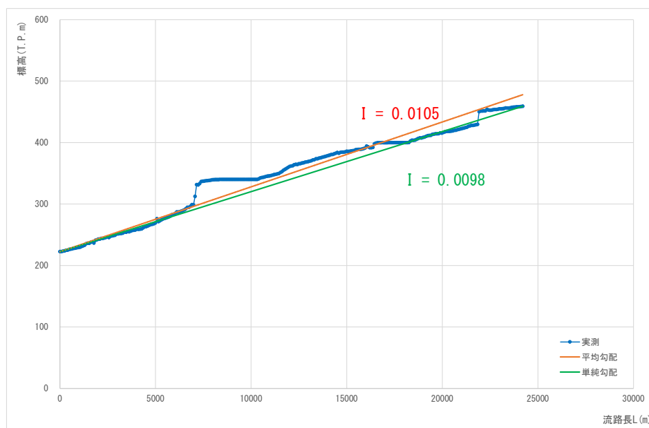
図 1.18 (3) 流域流路勾配 (流域番号 K3)
