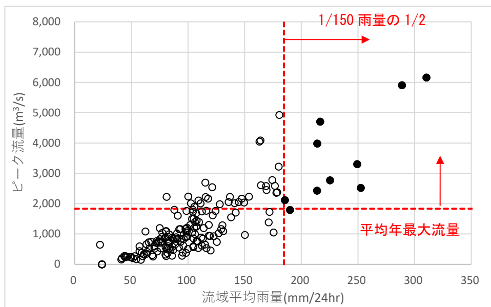
図 1.48 対象洪水の選定結果（基準地点：中角地点）
