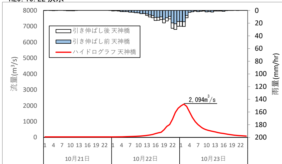
図 1.55 (4) 基本高水ハイドロ (基準地点：天神橋地点)
