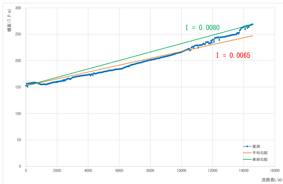
図 1.18 (9) 流域流路勾配 (流域番号 K9)
