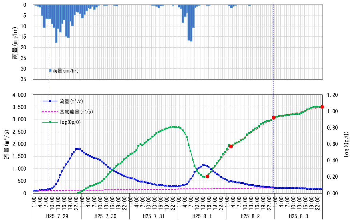
图 1.11 (7) 流出成分分離結果 (中角 H25.7.29 )
