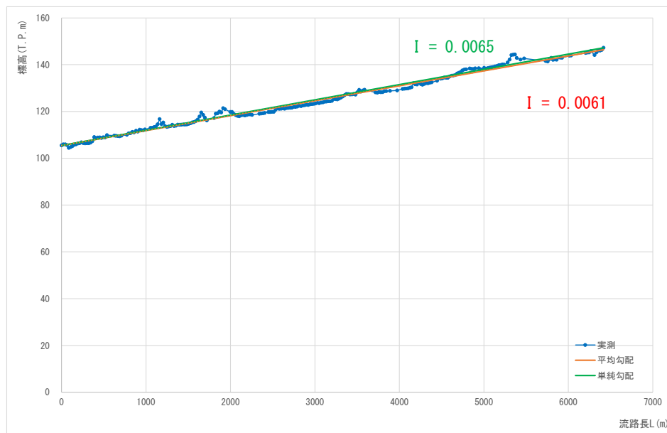
図 1.18 (17) 流域流路勾配（流域番号 A2）
