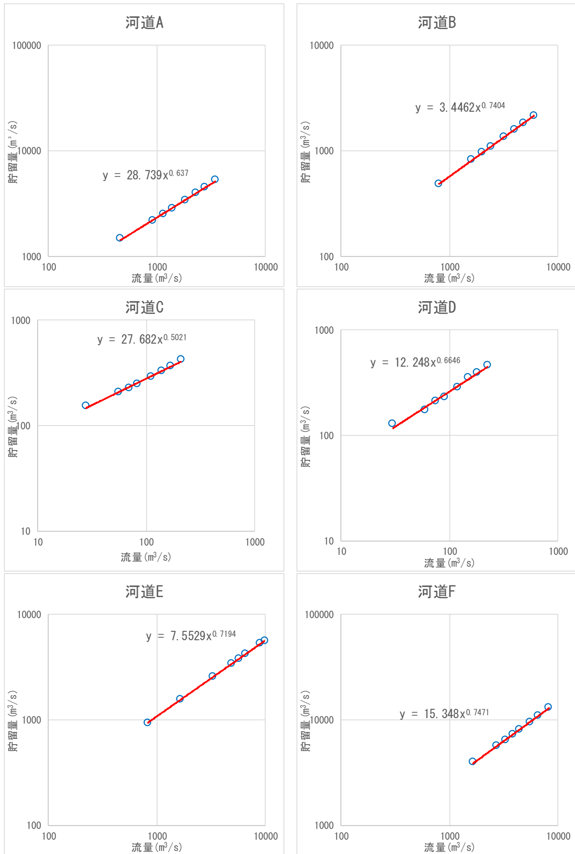
図 1.21 (1) S-Q 関係図 (計画河道)
