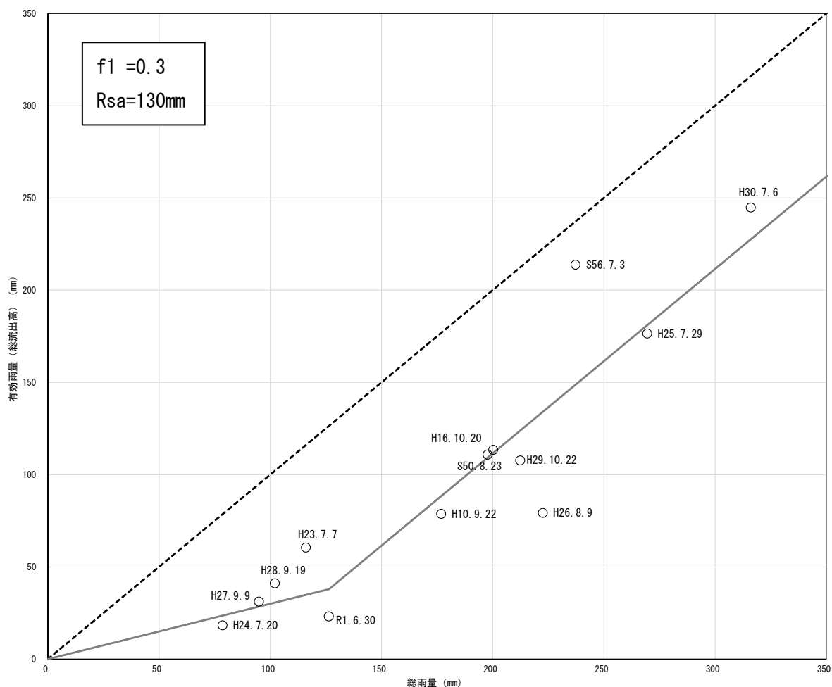
図 1.12 総雨量-総流出高の関係
