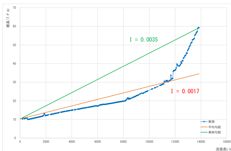
图 1.18 (25) 流域流路勾配 (流域番号 H6)
