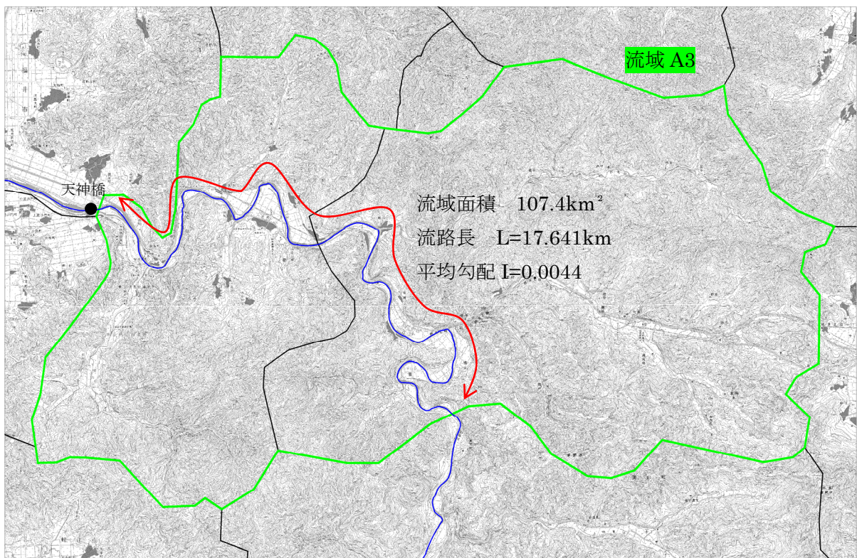
图 1.17 (18) 流路延長 (流域番号 A3)
