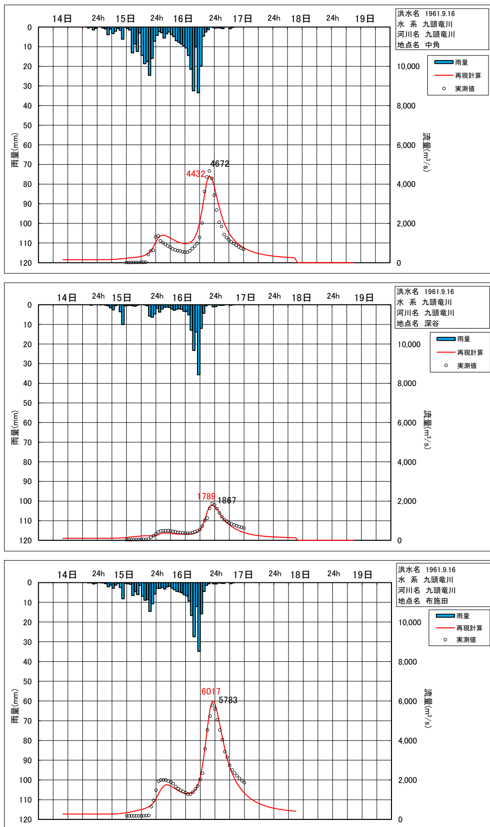
図 1.24 S36.9.16 洪水ハイドロの再現計算結果
