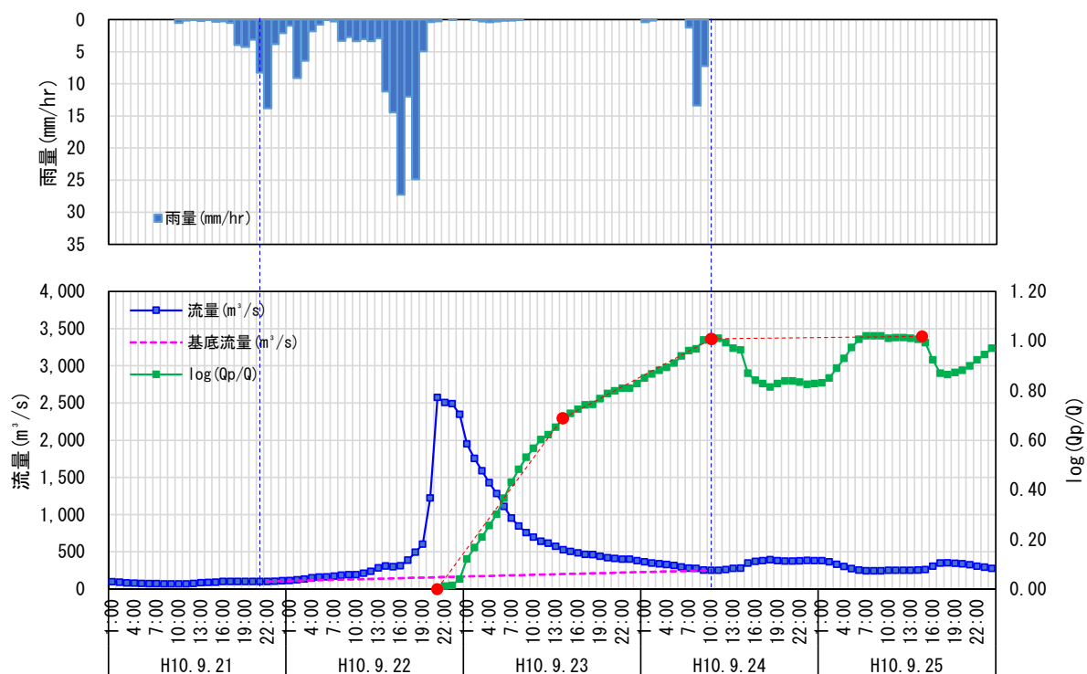
图 1.11 (3) 流出成分分離結果 (中角 H10.9.22)
