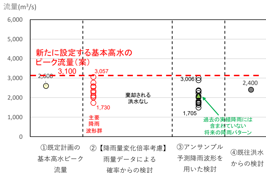
図 1.69 基本高水の設定に関する総合判断（基準地点：深谷地点）
