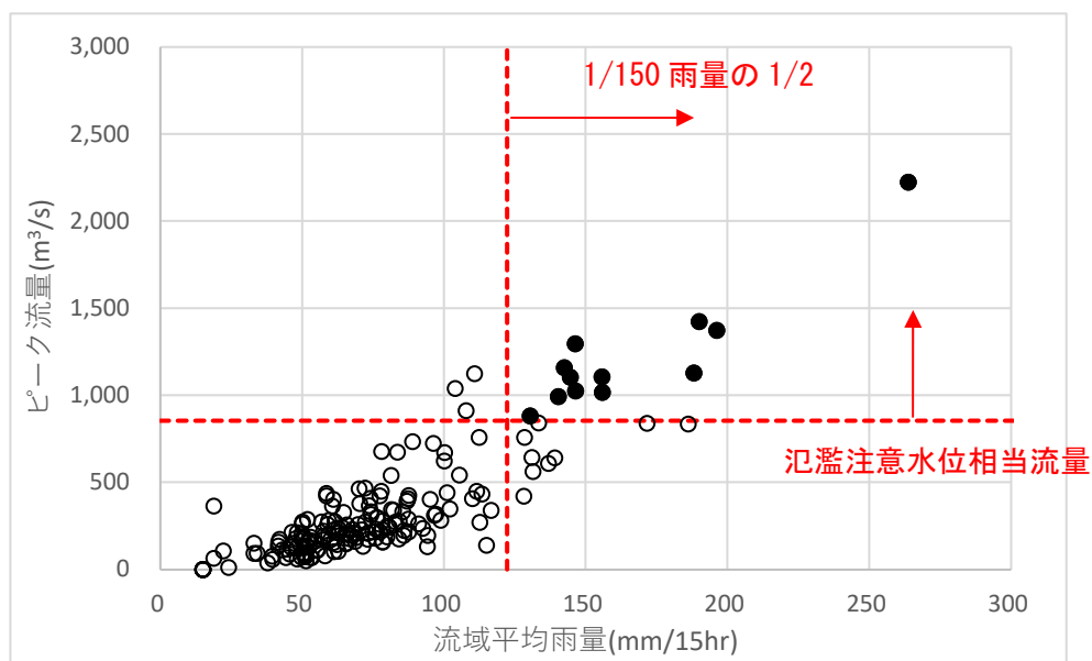
図 1.50 対象洪水の選定結果（基準地点：天神橋地点）
