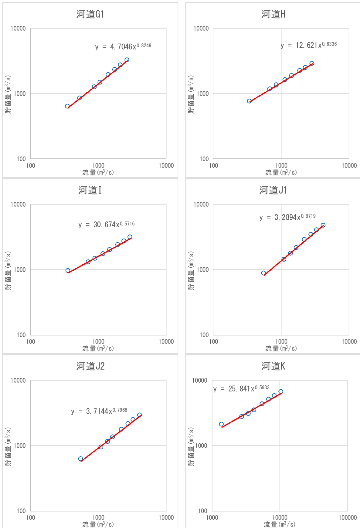
図 1.20 (2) S-Q 関係図 (現況河道)
