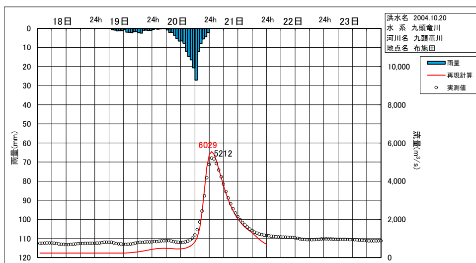
図 1.34 H16. 10. 20 洪水ハイドロの再現計算結果 (1/2)
