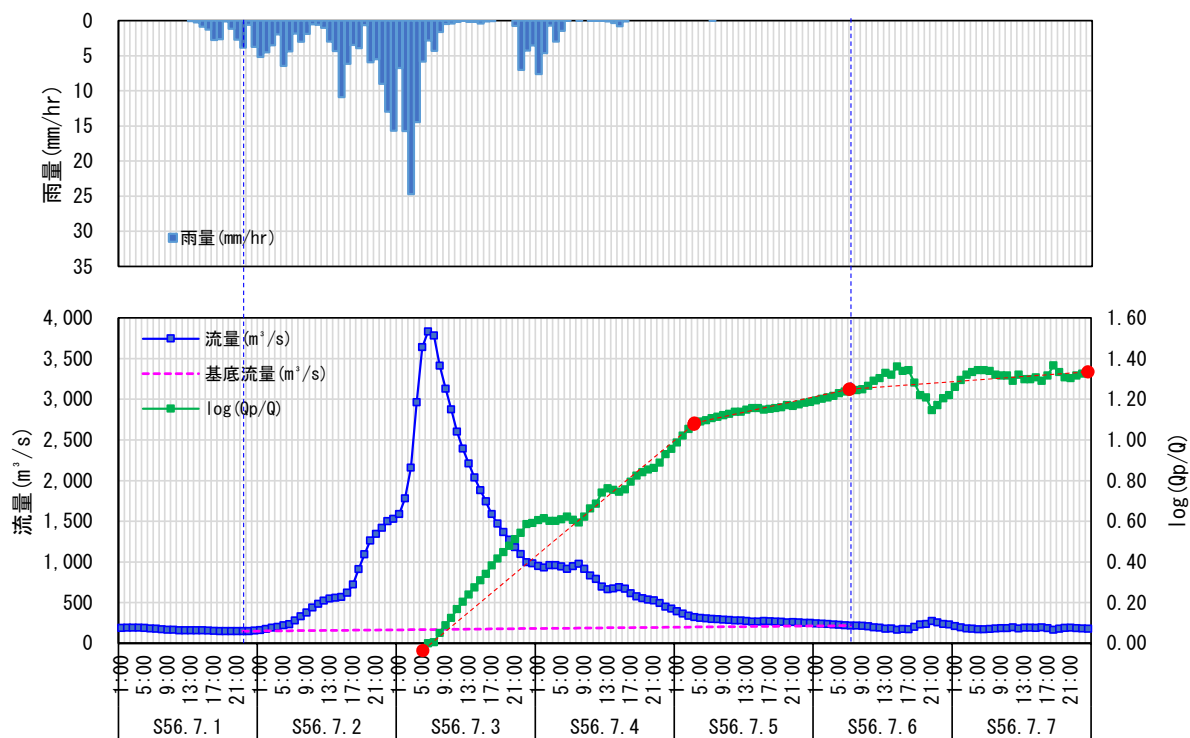
图 1.11 (2) 流出成分分離結果 (中角 S56.7.3)
