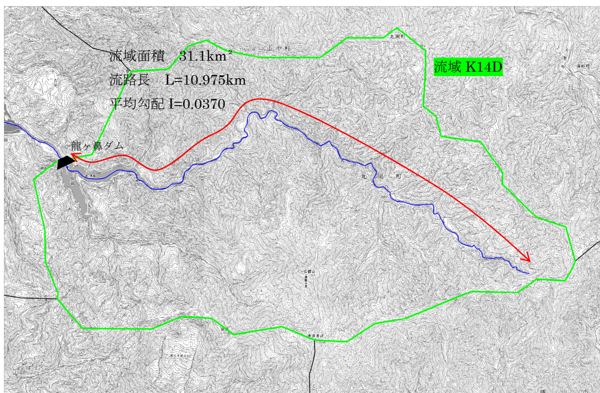
図 1.17 (14) 流路延長 (流域番号 K14D)
