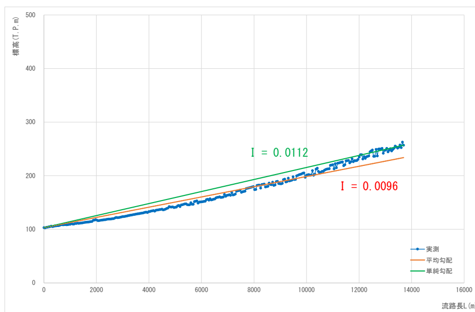
図 1.18 (21) 流域流路勾配 (流域番号 H2)
