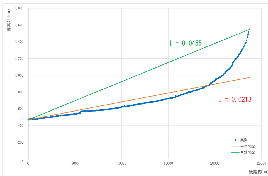
図 1.18 (2) 流域流路勾配 (流域番号 K2)
