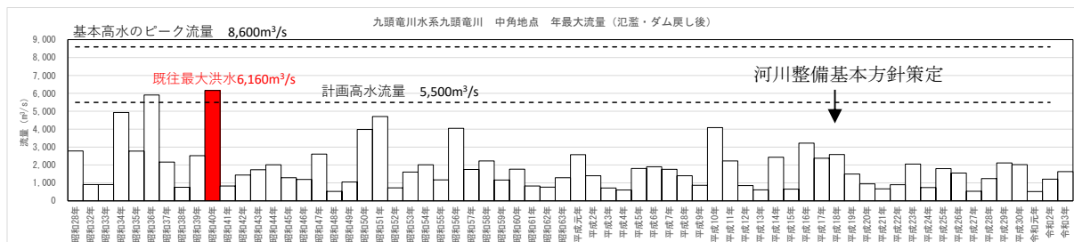
図 1.1 年最大流量（基準地点中角）
