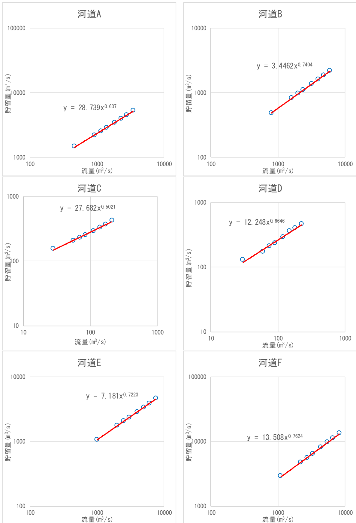
図 1.20 (1) S-Q 関係図 (現況河道)
