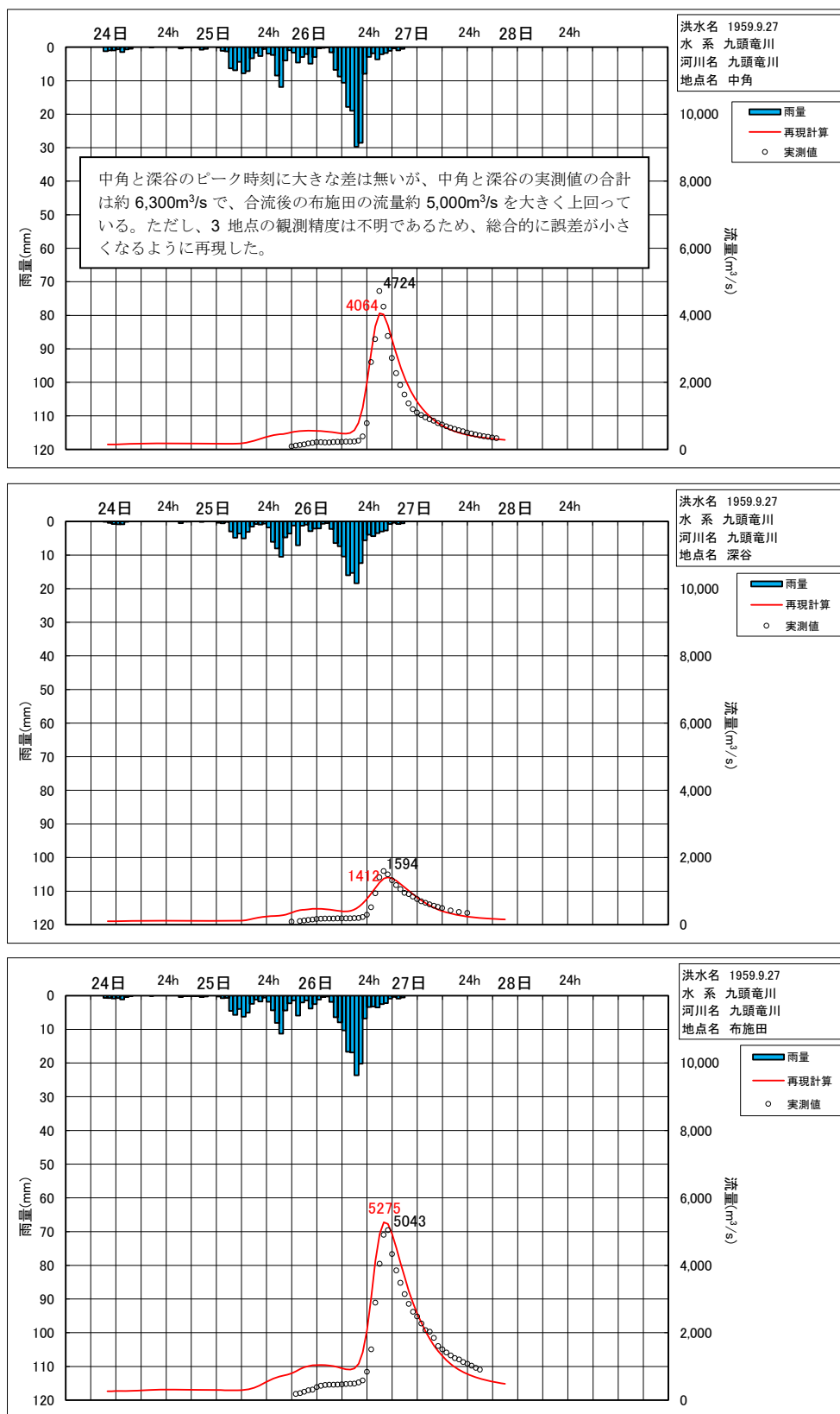
図 1.23 S34. 9. 27 洪水ハイドロの再現計算結果
