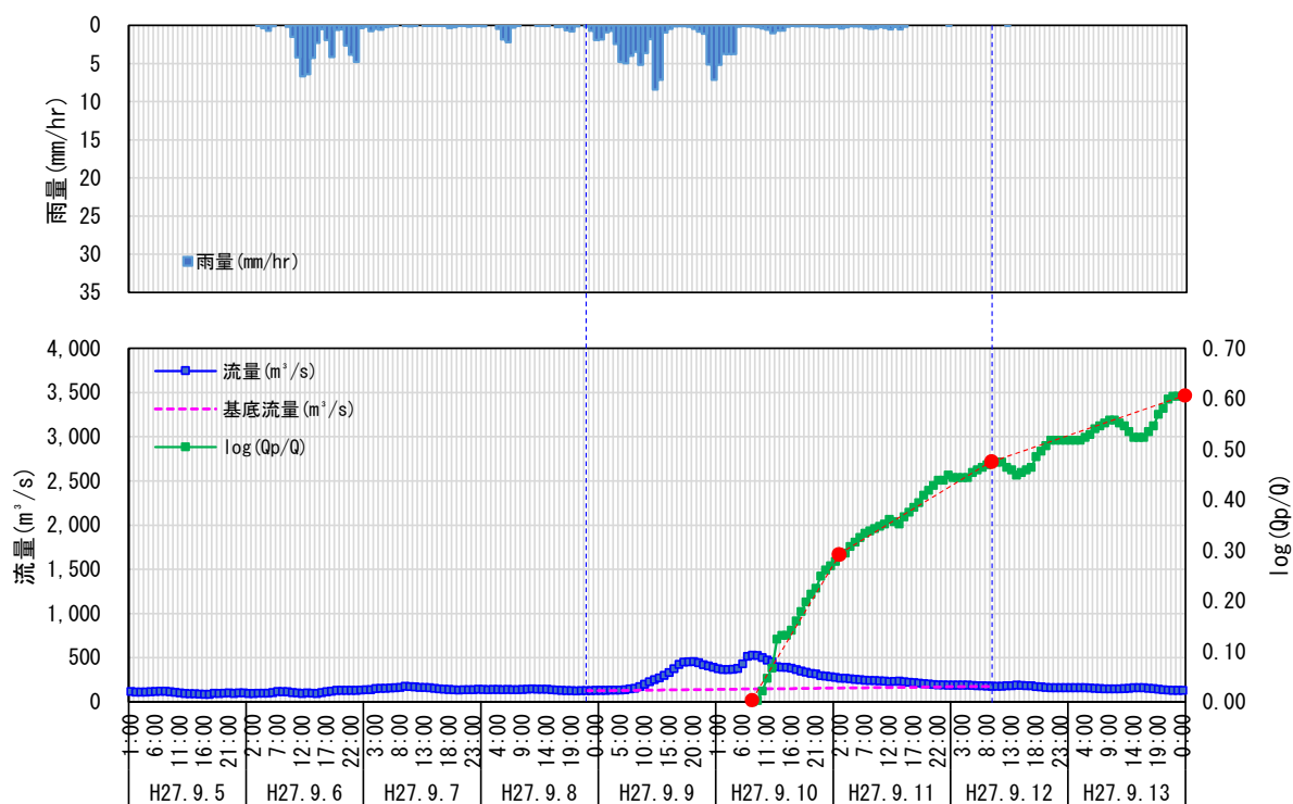
图 1.11 (9) 流出成分分離結果 (中角 H27.9.9)
