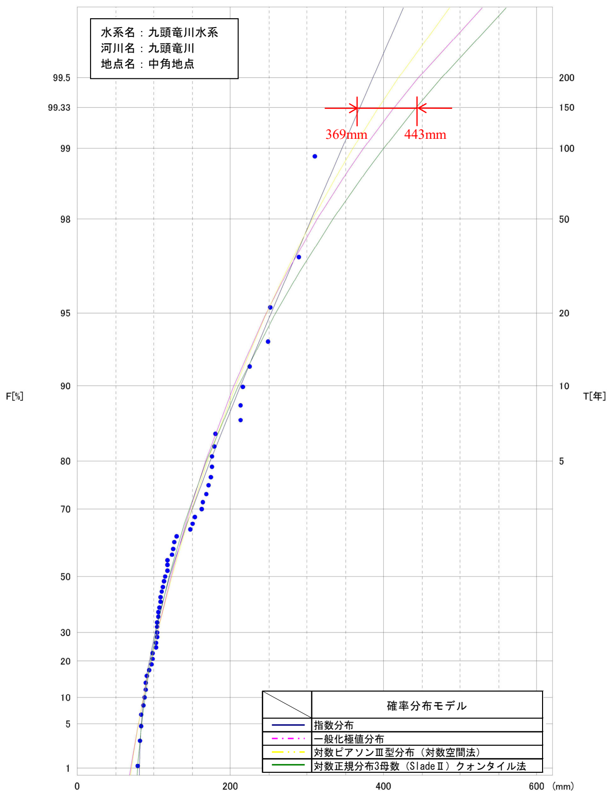
図 1.45 中角地点における雨量確率計算結果
