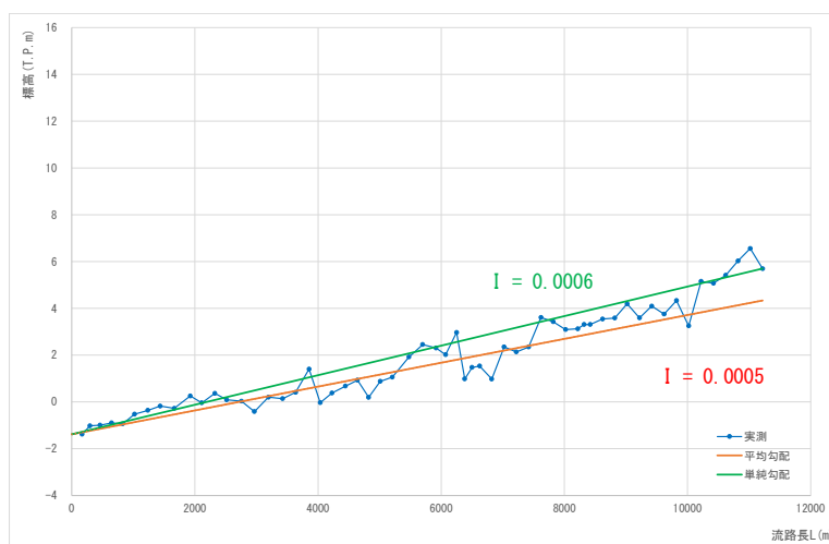
图 1.18 (26) 流域流路勾配 (流域番号 H7)
