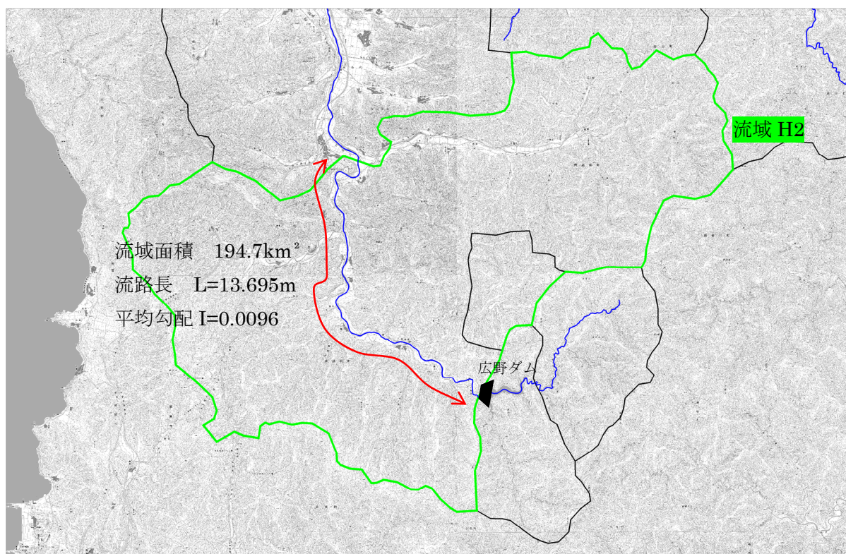
図 1.17 (21) 流路延長 (流域番号 H2)
