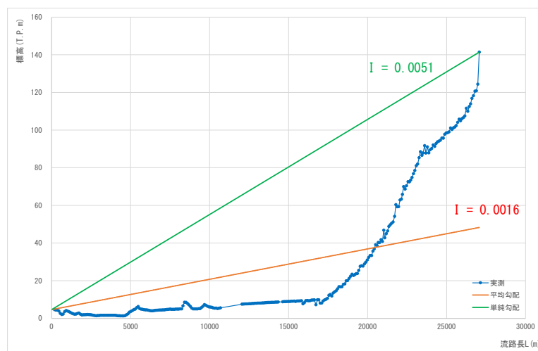
图 1.18 (15) 流域流路勾配 (流域番号 K14Z)
