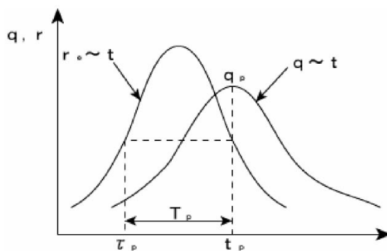
図 1.36 Kinematic Wave 法に基づく洪水到達時間の設定
