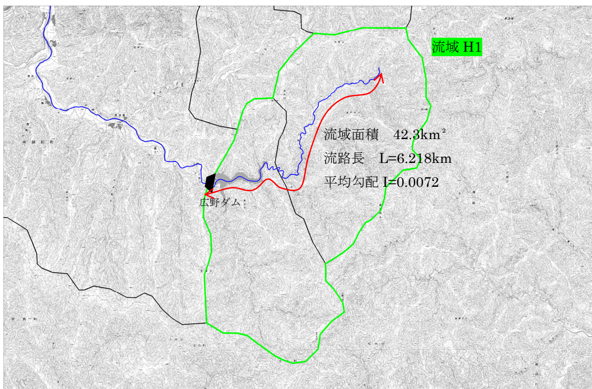
図 1.17 (20) 流路延長 (流域番号 H1)
