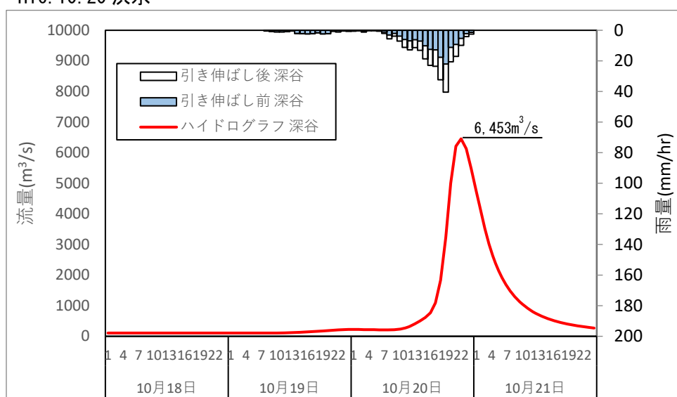
図 1.54 (1) 基本高水ハイドロ (基準地点：深谷地点)
