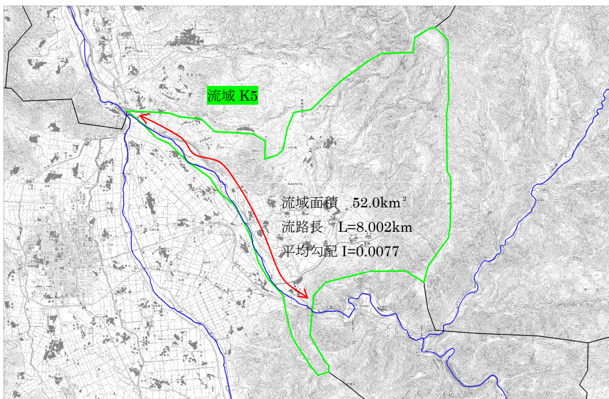
图 1.17 (5) 流路延長 (流域番号 K5)
