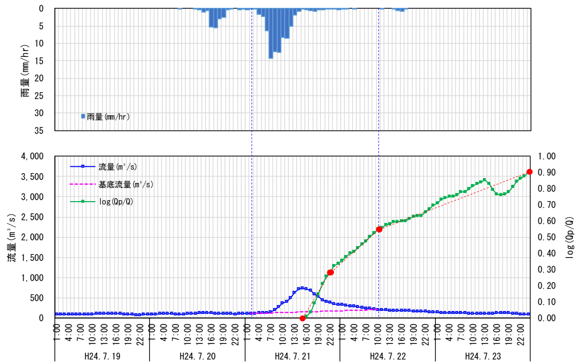
图 1.11 (6) 流出成分分離結果 (中角 H24.7.20)
