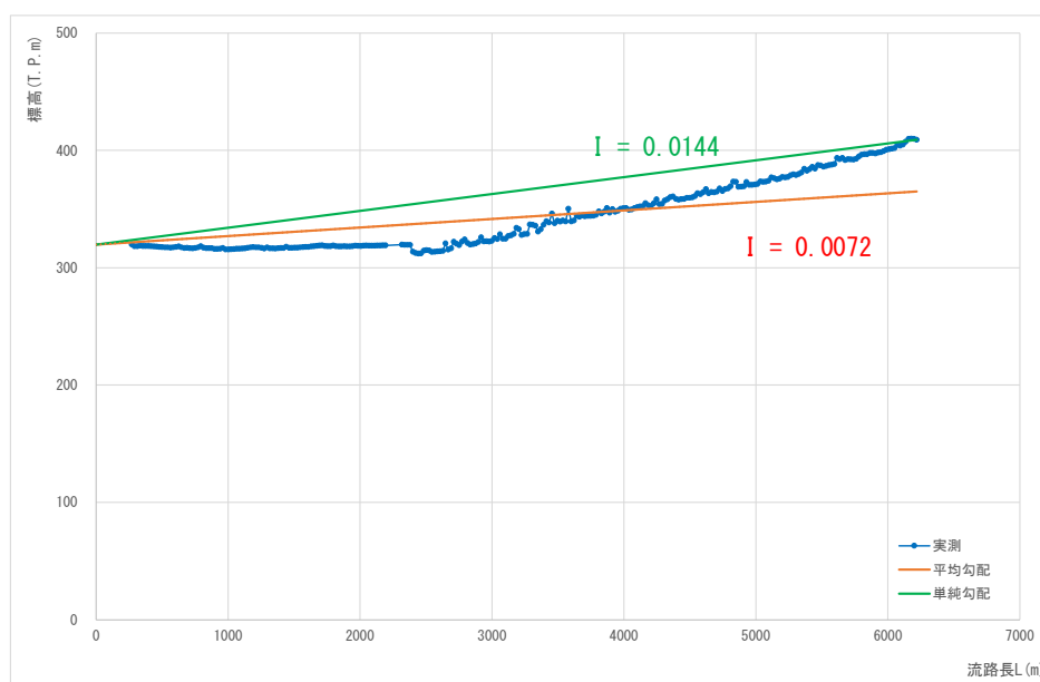
図 1.18 (20) 流域流路勾配 (流域番号 H1)
