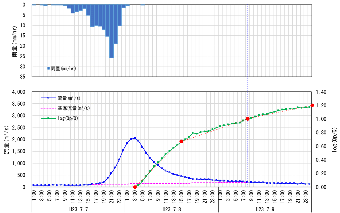
图 1.11 (5) 流出成分分離結果 (中角 H23.7.7)
