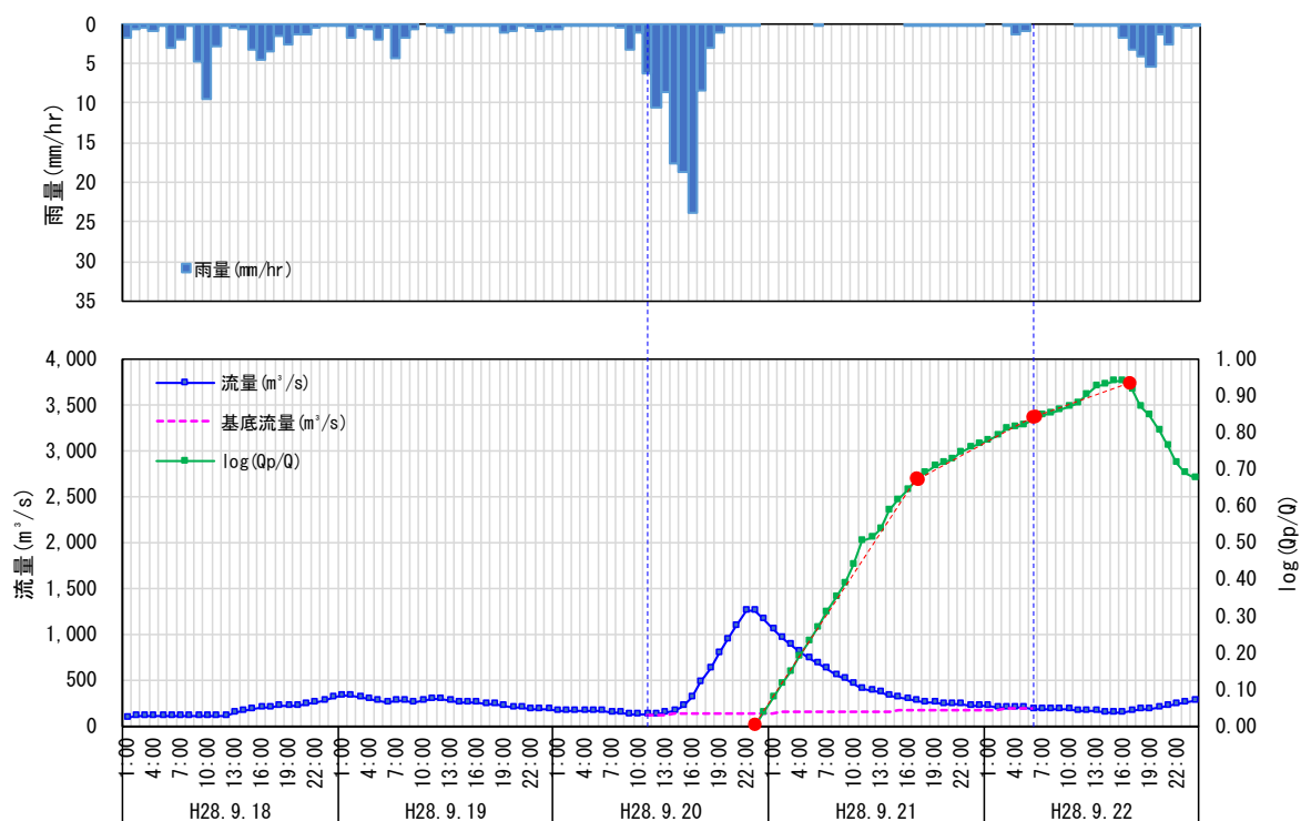
图 1.11 (10) 流出成分分離結果 (中角 H28.9.19)
