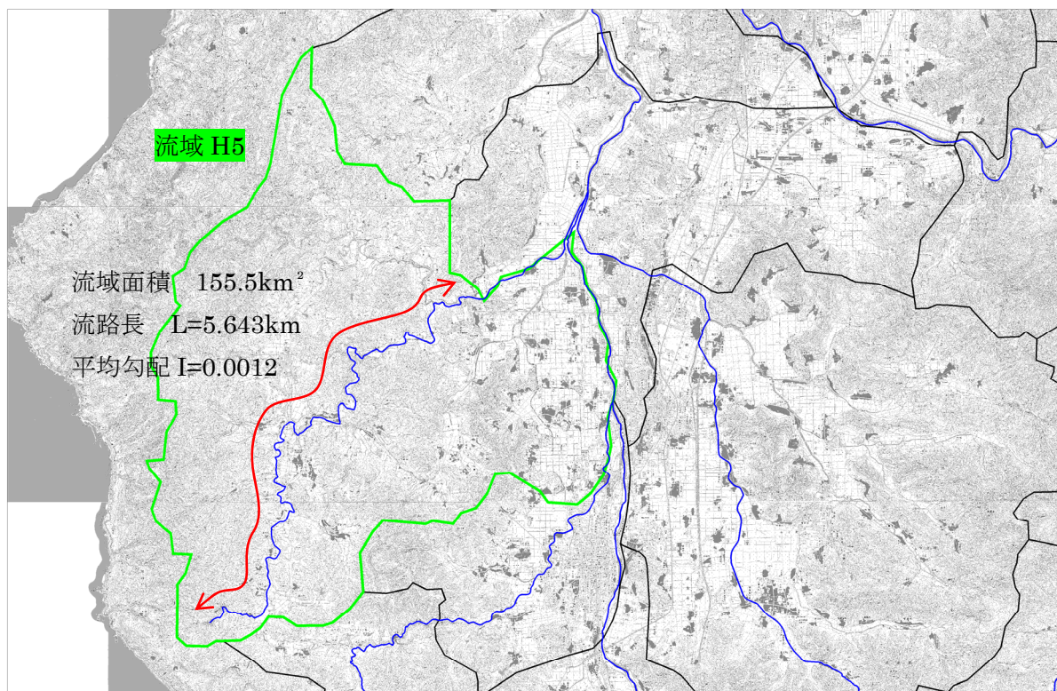
图 1.17 (24) 流路延長 (流域番号 H5)
