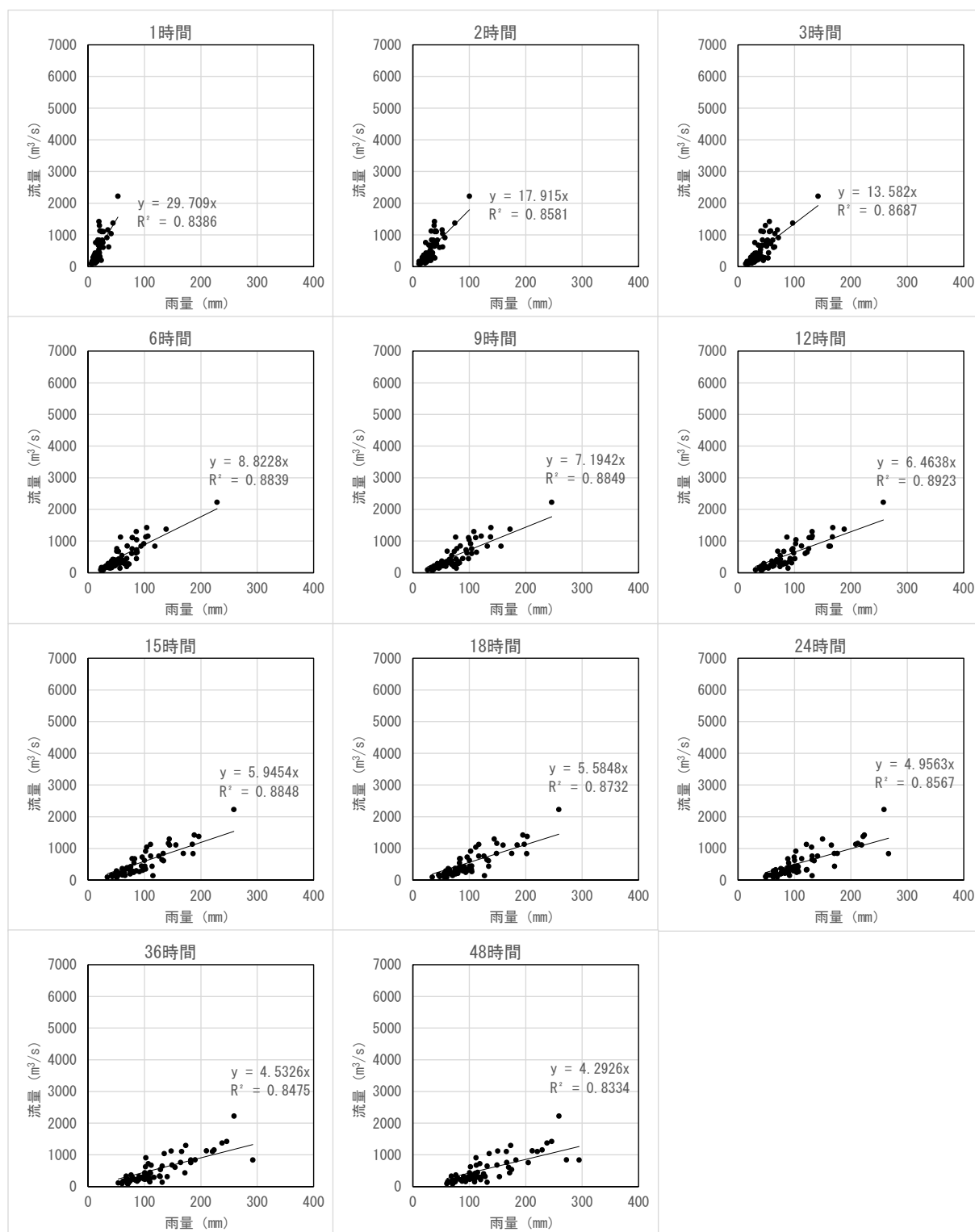
図 1.42 ピーク流量と雨量の相関関係（天神橋地点）
