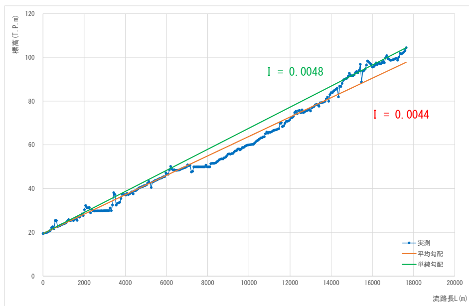
图 1.18 (18) 流域流路勾配 (流域番号 A3)
