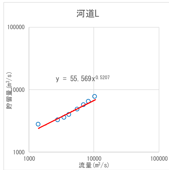
図 1.20 (3) S-Q 関係図 (現況河道)
