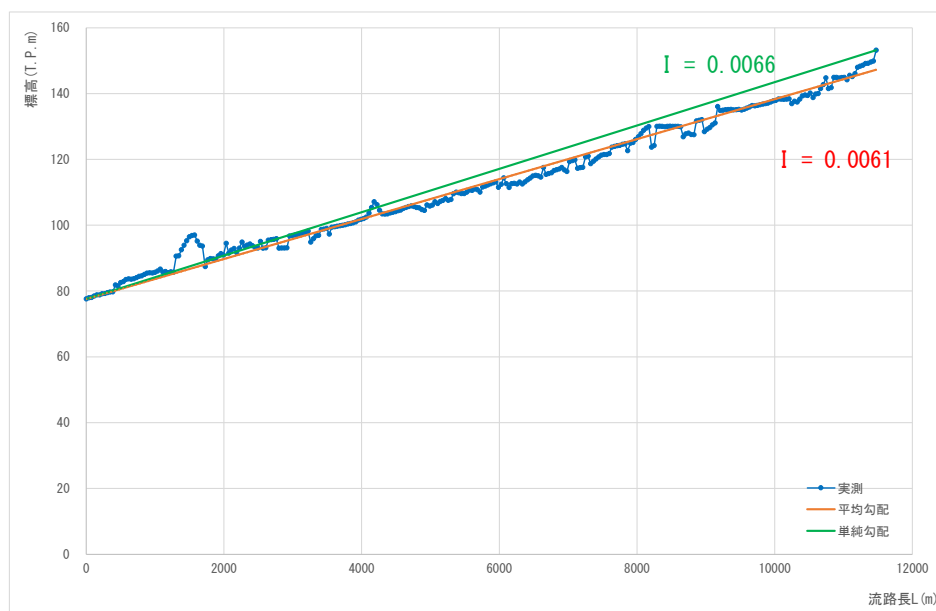
図 1.18 (10) 流域流路勾配 (流域番号 K10)
