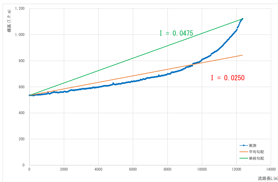
図 1.18 (7) 流域流路勾配 (流域番号 K7)
