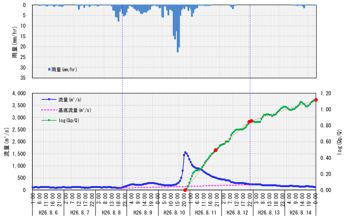
图 1.11 (8) 流出成分分離結果 (中角 H26.8.9)
