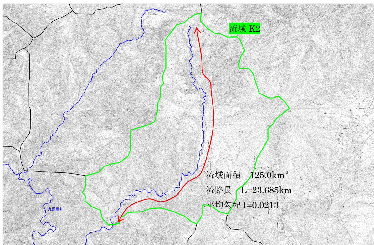
図 1.17 (2) 流路延長 (流域番号 K2)
