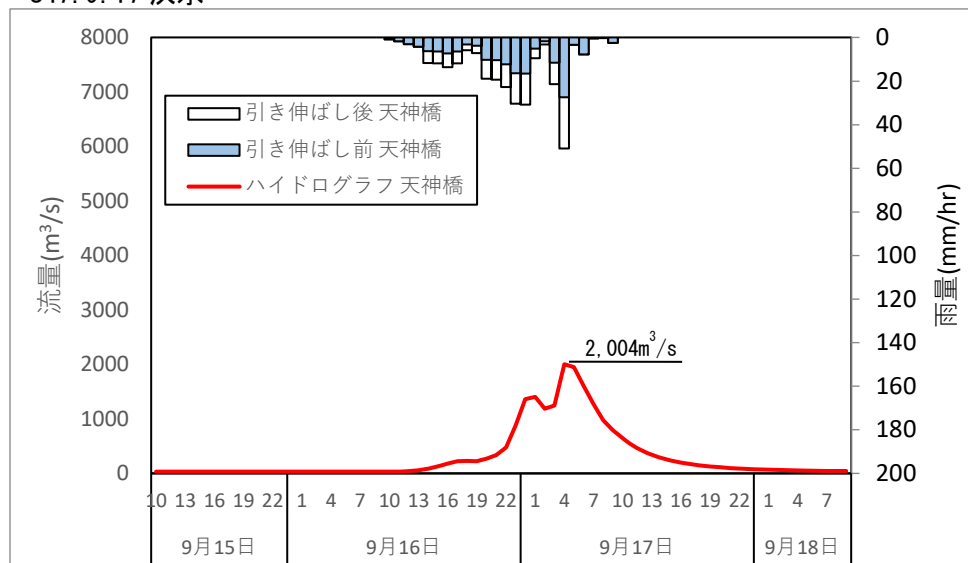
図 1.55 (2) 基本高水ハイドロ (基準地点：天神橋地点)
