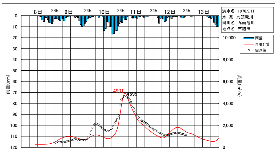
図 1.28 S51.9.11 洪水ハイドロの再現計算結果 (1/2)
