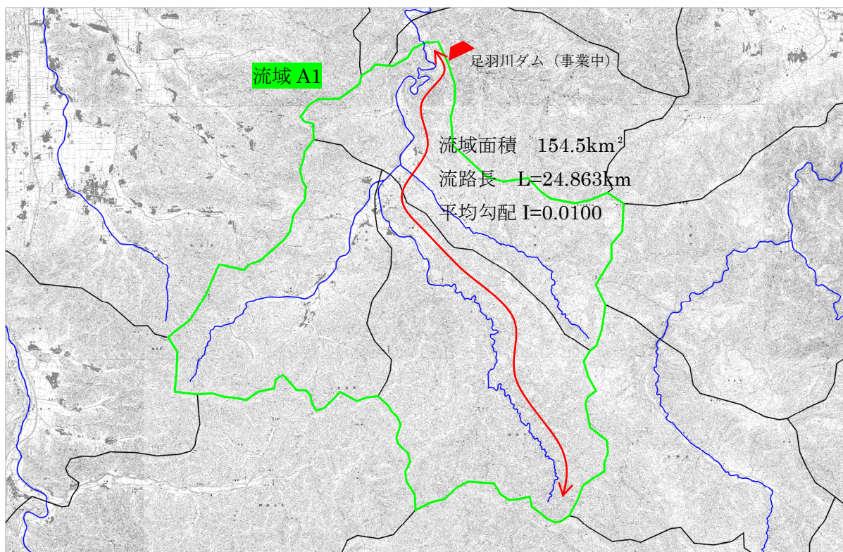
図 1.17 (16) 流路延長 (流域番号 A1)
