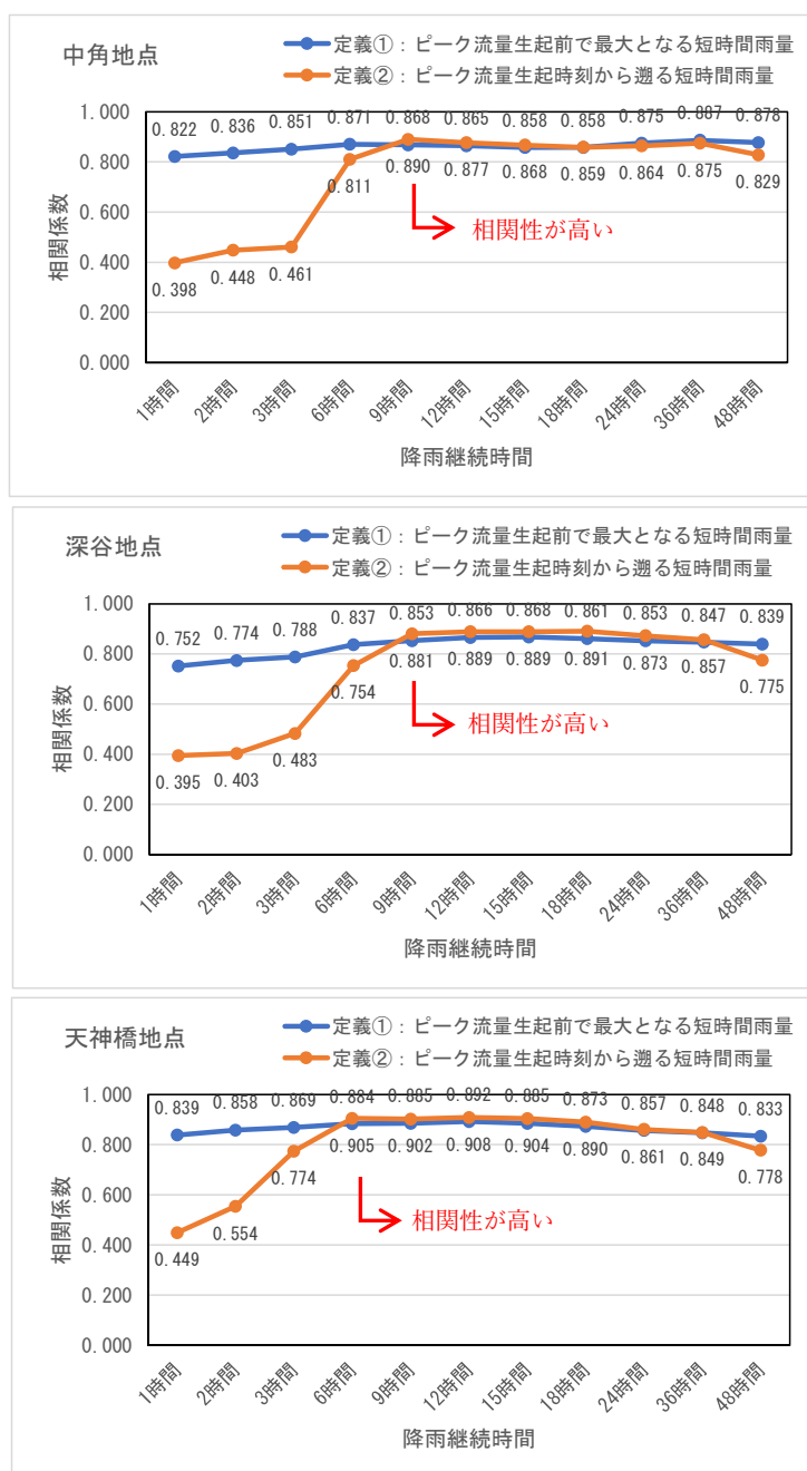
図 1.37 ピーク流量と降雨継続時間の相関図
