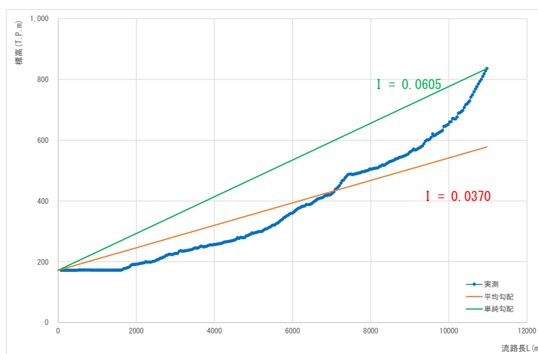
图 1.18 (14) 流域流路勾配 (流域番号 K14D)
