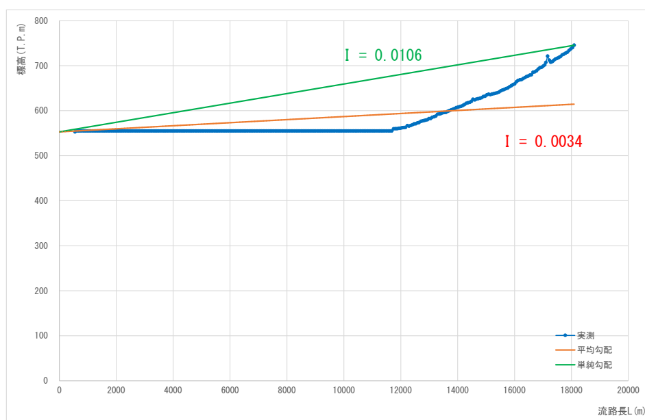
図 1.18 (1) 流域流路勾配 (流域番号 K1)
