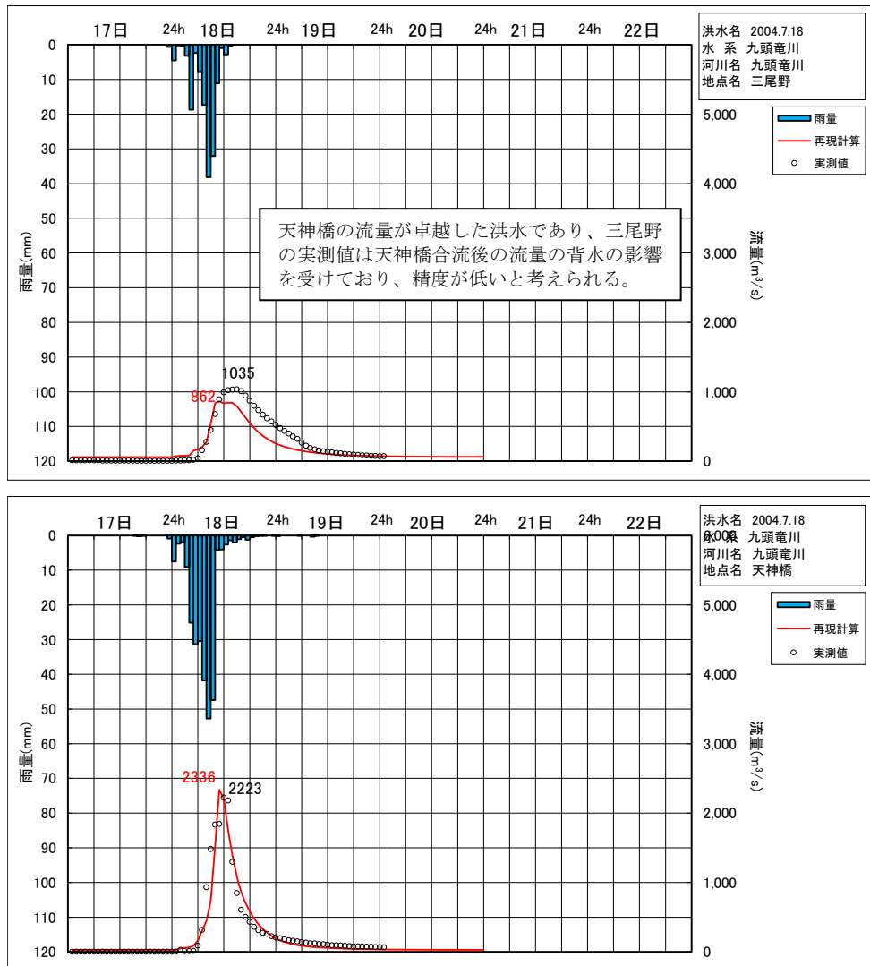
図 1.33 H16.7.17 洪水ハイドロの再現計算結果 (2/2)
