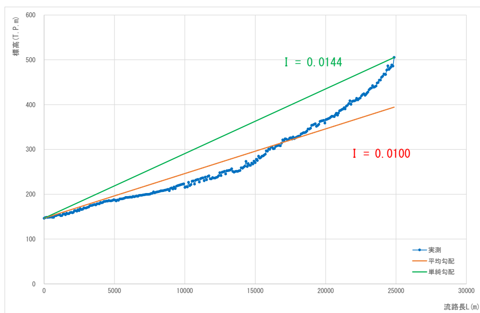
図 1.18 (16) 流域流路勾配 (流域番号 A1)
