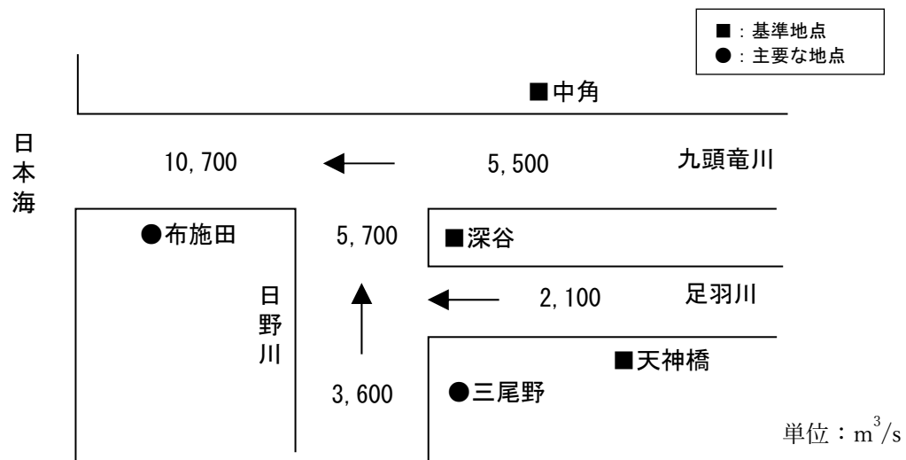
図 3.1 計画高水流量配分図
