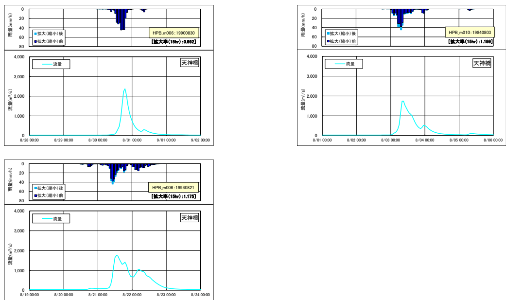
図 1.61 (2) 抽出した予測降雨波形群によるハイドログラフ（基準地点：天神橋地点）
