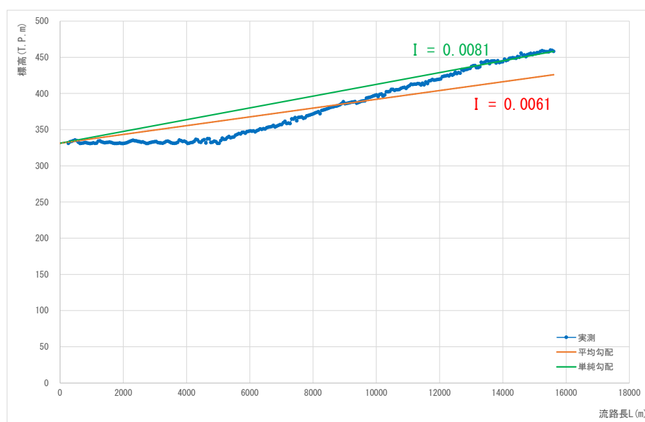
図 1.18 (8) 流域流路勾配 (流域番号 K8)
