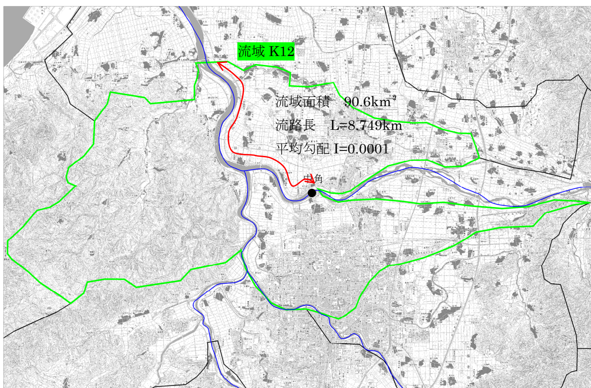
図 1.17 (12) 流路延長 (流域番号 K12)
