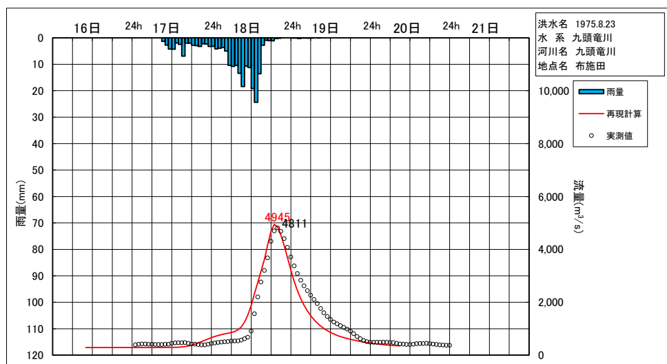
図 1.26 S50.8.23 洪水ハイドロの再現計算結果 (1/2)
