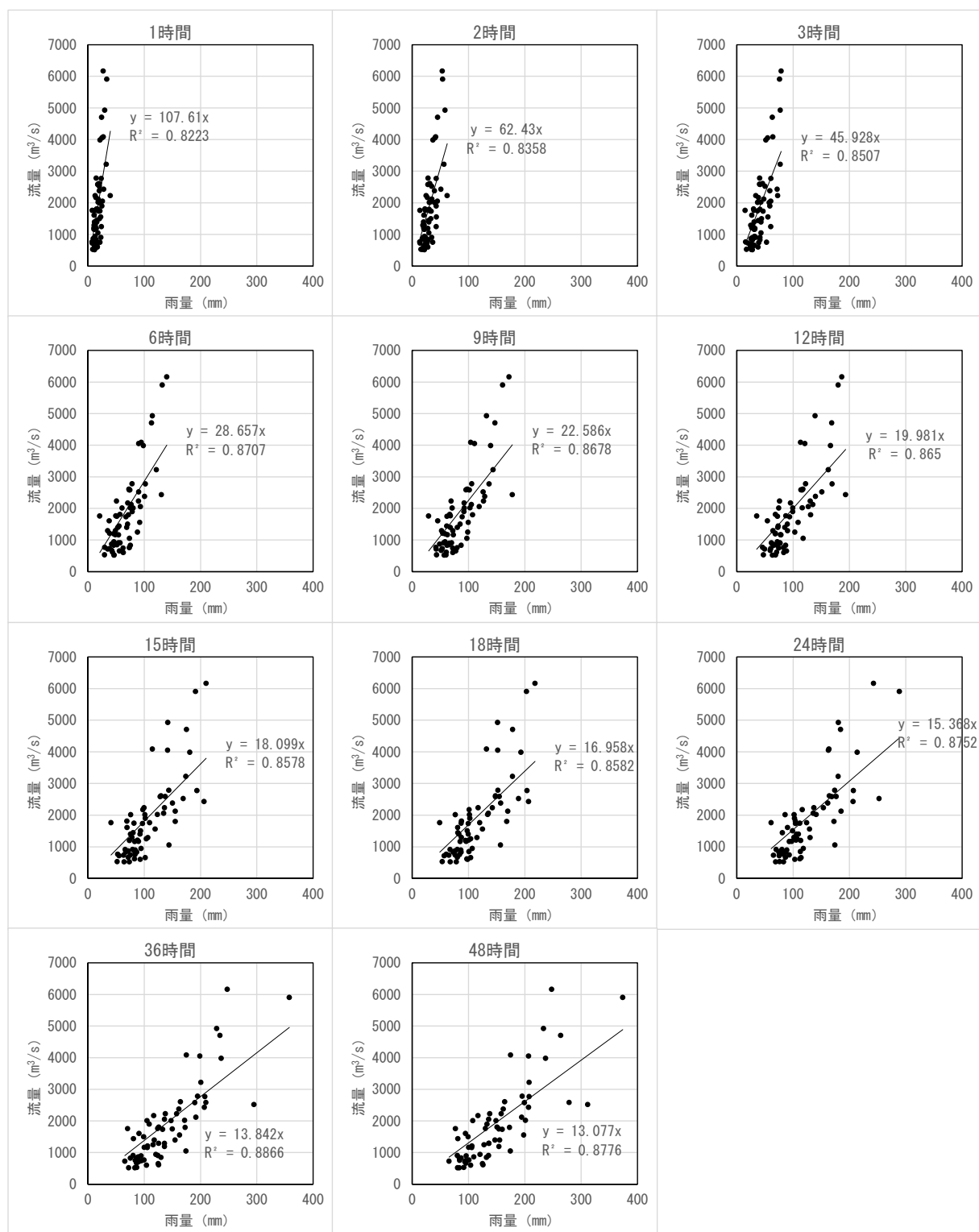
図 1.38 ピーク流量と雨量の相関関係（中角地点）
