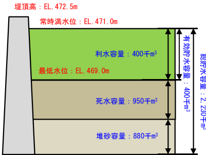
双珠別ダム容量配分図
