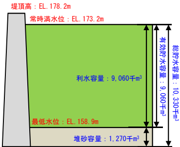
穂別ダム容量配分図
