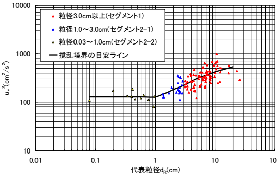
攪乱境界の摩擦速度の2乗 ( u_*^2 ) 調査結果
