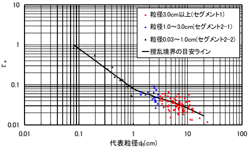
攪乱境界の無次元掃流力 ( \tau_* ) 調査結果
