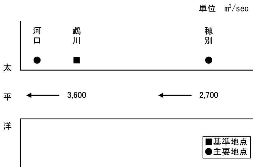
図 4-1 鷓川水系河川整備基本方針における計画高水流量配分図
