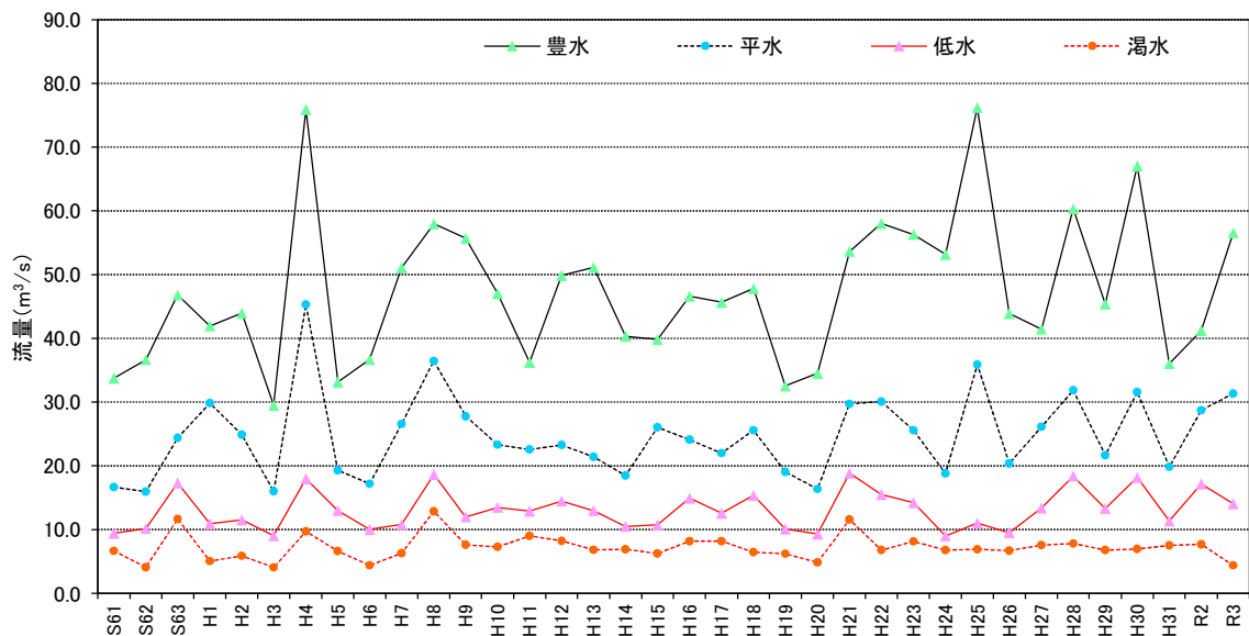
図 6-1 鷓川地点流況経年変化図
