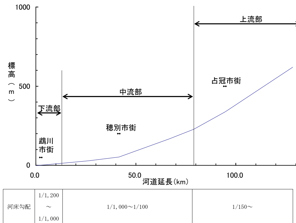
図 8-1 鷓川河床高縦断面図
