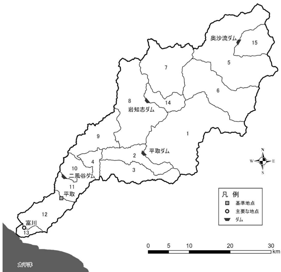
図 1-3 流域分割図
