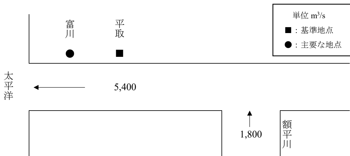
図 3-1 沙流川計画高水流量図
