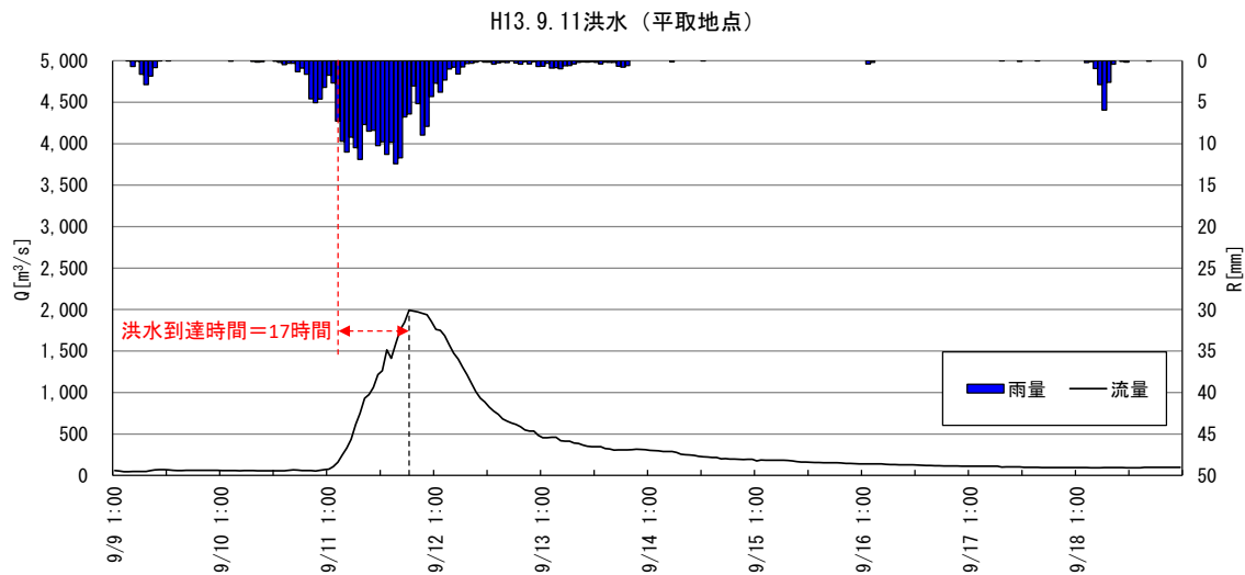
図 1-16(5) Kinematic Wave 法による洪水到達時間（平成 13 年 9 月洪水）
