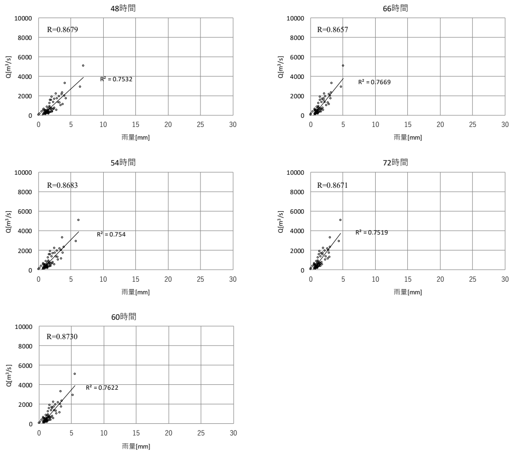
図 1-19 (2) ピーク流量と流域平均時間雨量の相関図【定義②】
