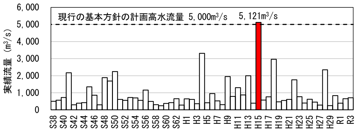
図 1-2 年最大流量 (基準地点平取)
