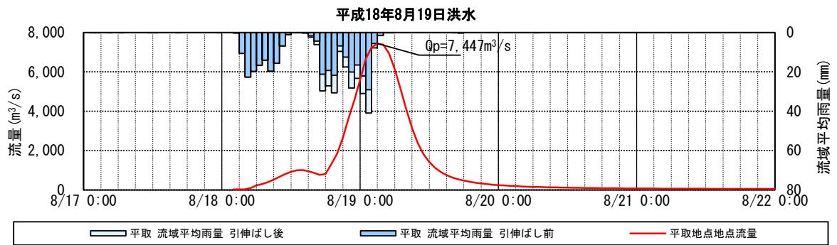
図 1-24(5) 基本高水ハイドログラフ (基準地点平取)
