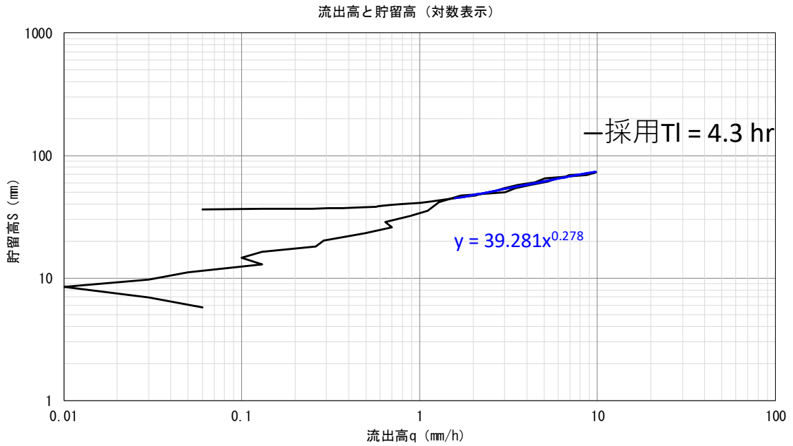
図 1-8(5) 貯留高-流出高関係図 (幌毛志橋地点:平成 28 年 8 月 31 日洪水)
