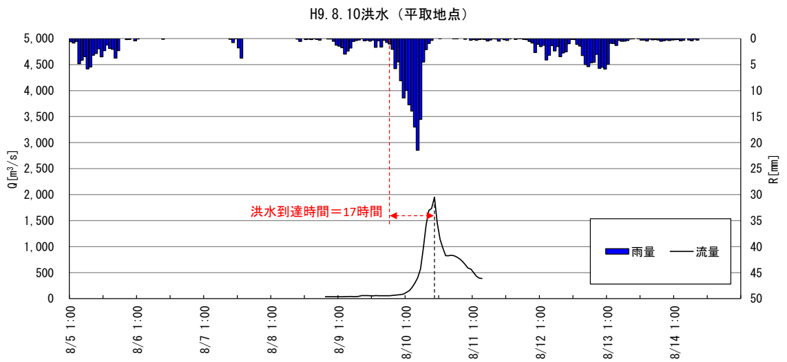
図 1-16(4) Kinematic Wave 法による洪水到達時間（平成 9 年 8 月洪水）
