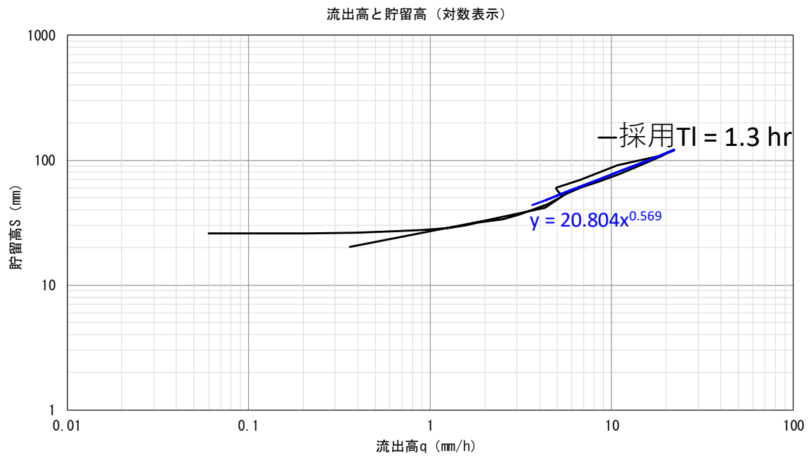
図 1-9(4) 貯留高-流出高関係図 (貫気別地点：平成 15 年 8 月洪水)
