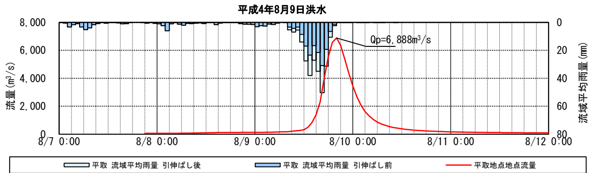
図 1-24(1) 基本高水ハイドログラフ (基準地点平取)
