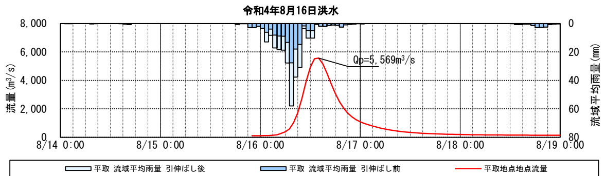
図 1-24(6) 基本高水ハイドログラフ (基準地点平取)
