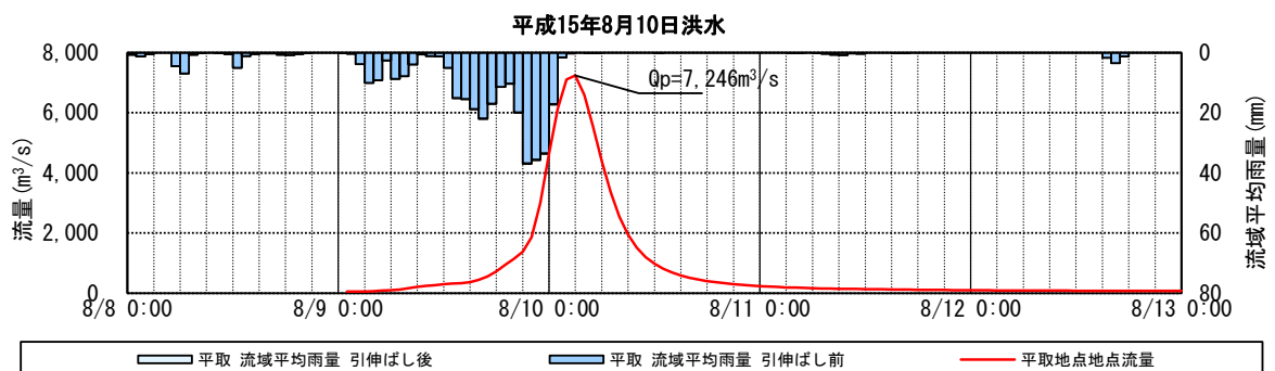
図 1-24(4) 基本高水ハイドログラフ (基準地点平取)
