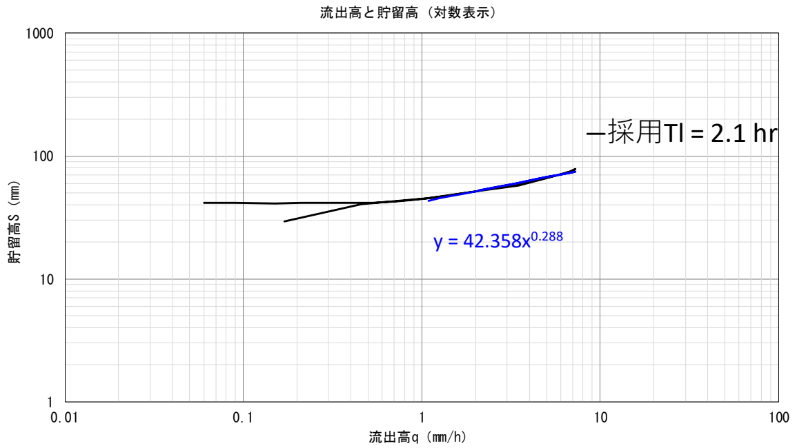
図 1-9(3) 貯留高-流出高関係図 (貫気別地点：平成9年8月洪水)
