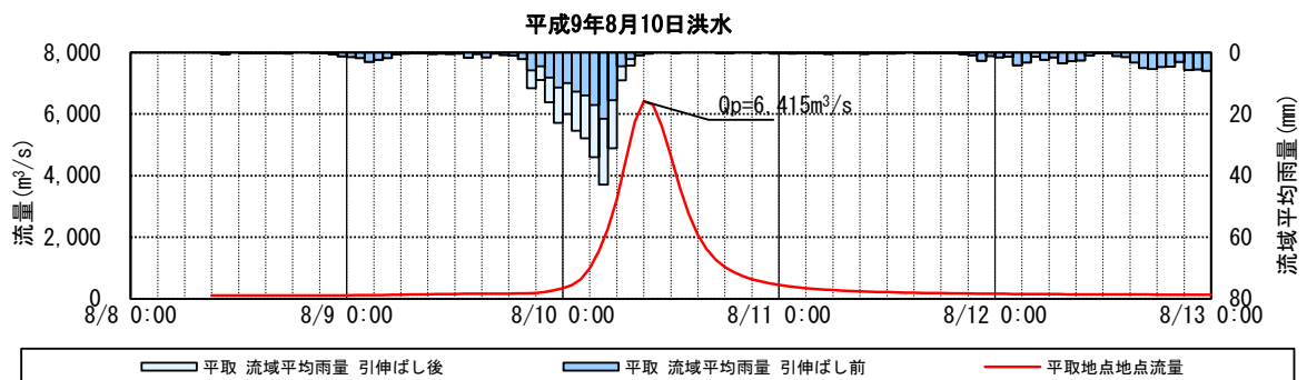
図 1-24(2) 基本高水ハイドログラフ (基準地点平取)
