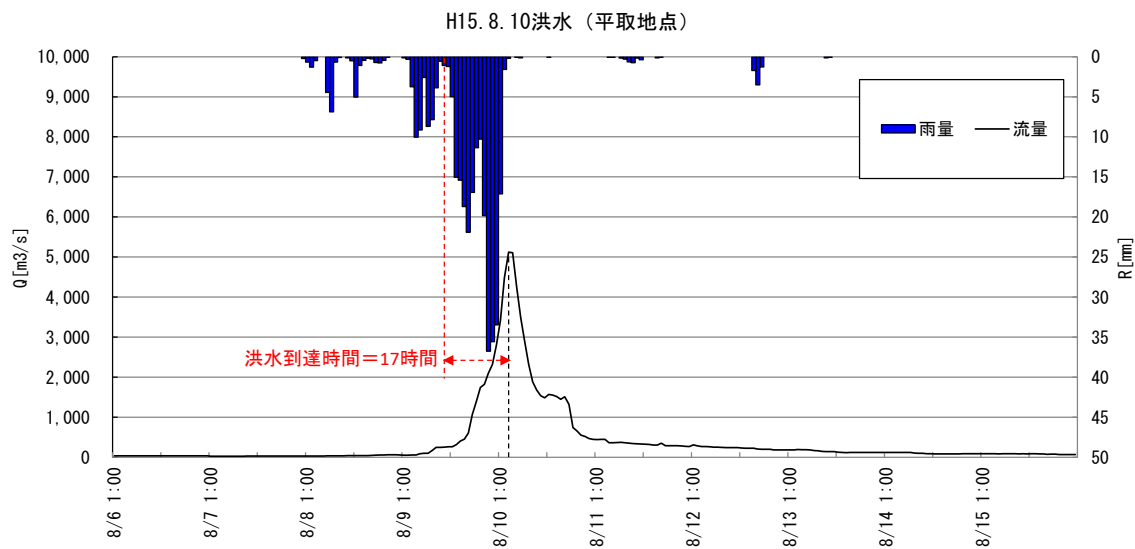
図 1-16(6) Kinematic Wave 法による洪水到達時間（平成 15 年 8 月洪水）
