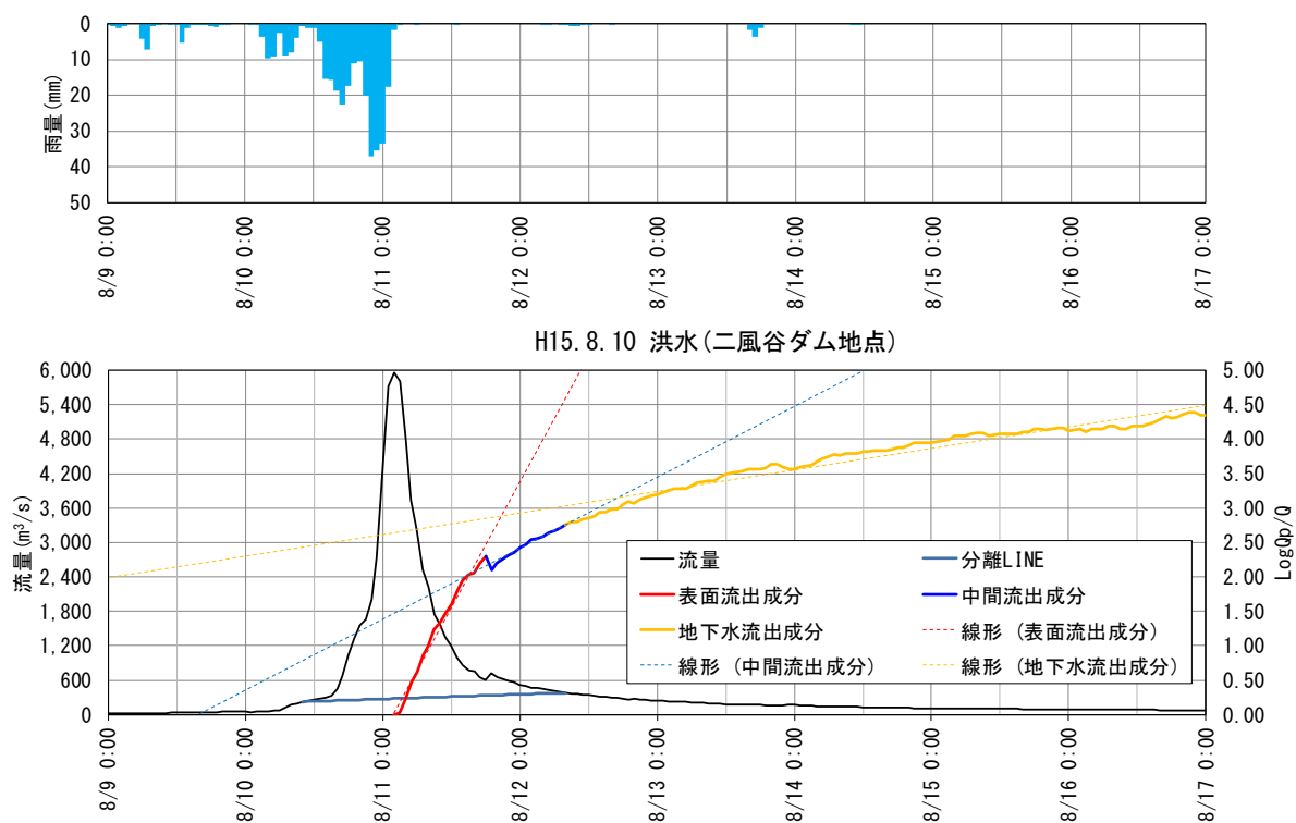
図 1-5 成分分離の事例 (H15. 8 洪水)
