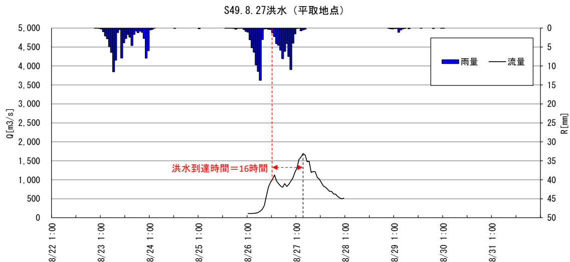
図 1-16(1) Kinematic Wave 法による洪水到達時間（昭和 49 年 8 月洪水）
