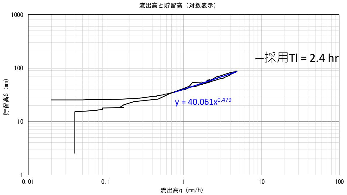
図 1-7(3) 貯留高-流出高関係図 (二風谷ダム地点：平成 22 年 8 月洪水)
