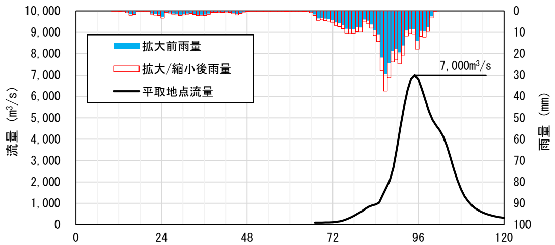
図 1-26(8) 抽出した予測降雨波形のハイドログラフ (基準地点平取)
