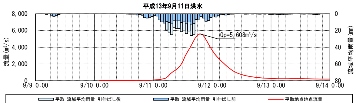
図 1-24(3) 基本高水ハイドログラフ (基準地点平取)
