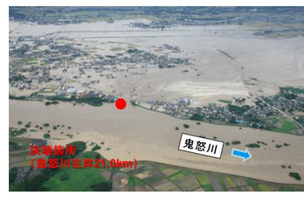
鬼怒川 常総市上三坂地先 決壊状況
