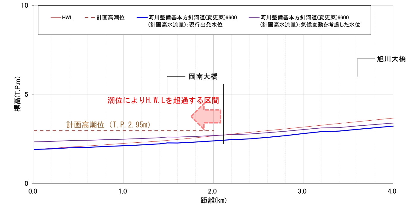
気候変動による海面水位上昇の影響を踏まえた水位縦断面図
