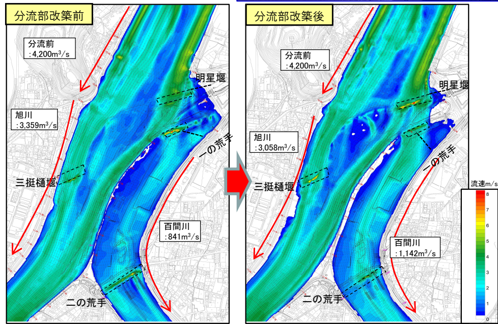
シミュレーション結果：平成30年7月豪雨実績による分流部(改築前後)の流速状況
