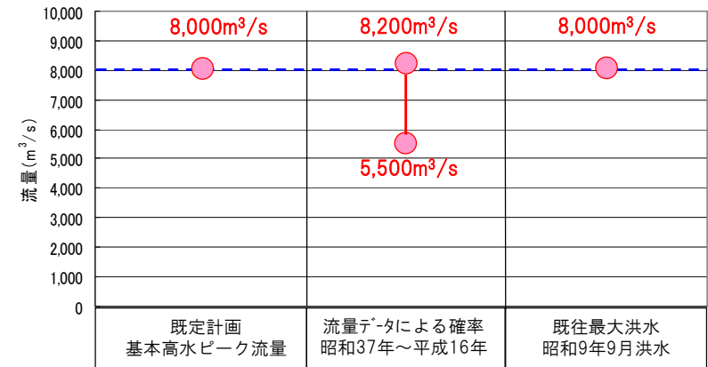
基本高水ピーク流量の検証
