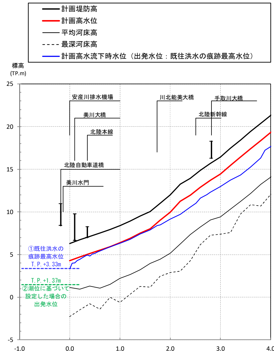
手取川水位縦断面図
