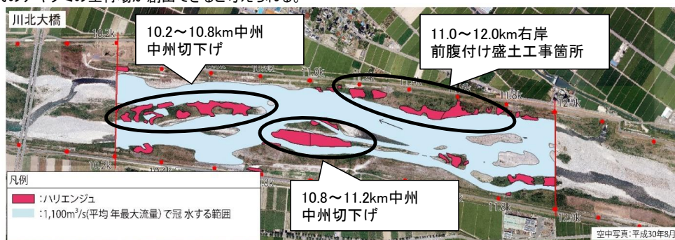
図 1,100m³/s(平均年最大流量)で冠水する範囲とハリエンジュの分布
