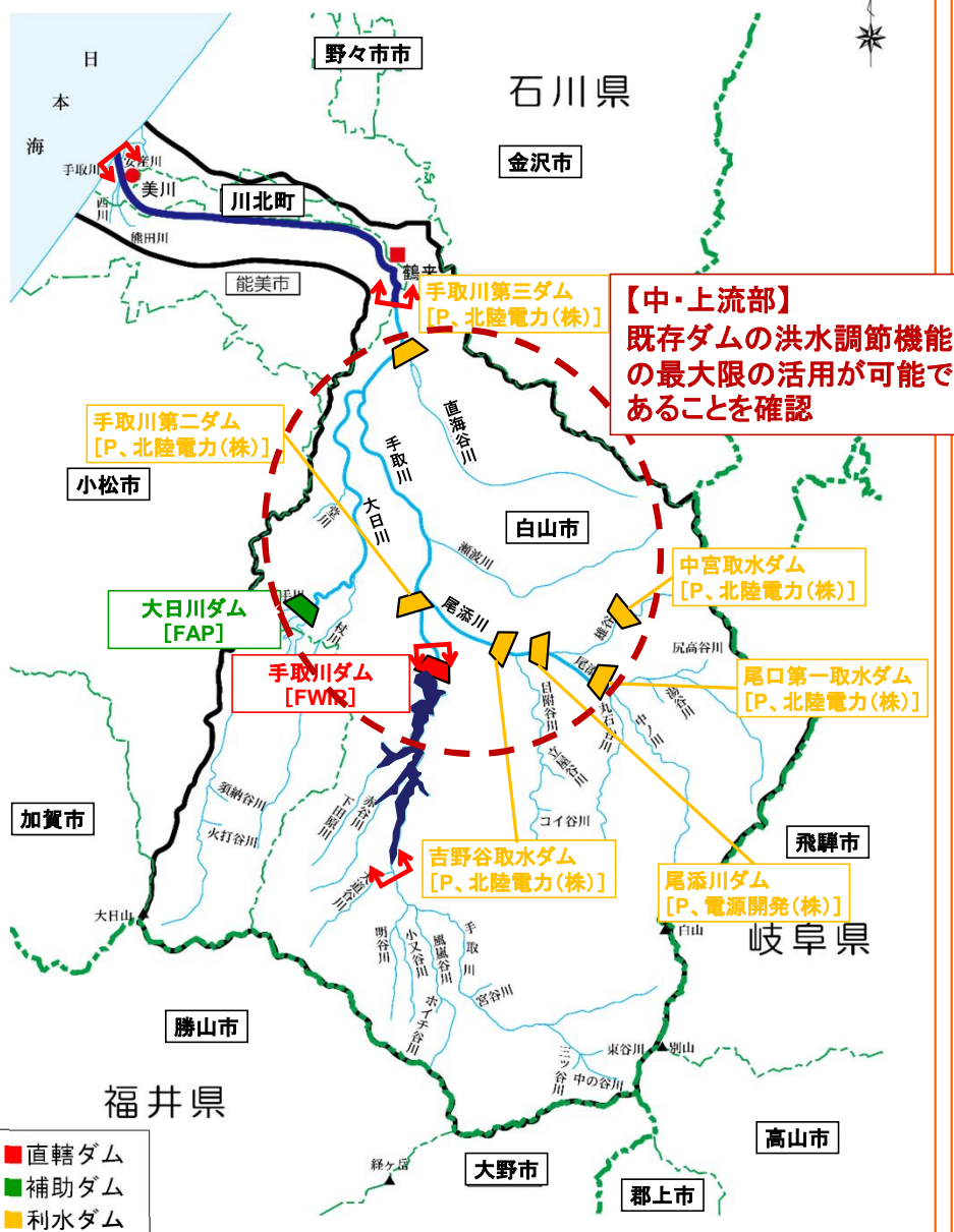
手取川流域のダム位置図
