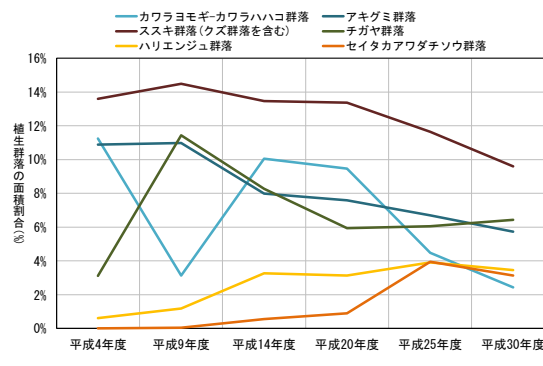
図 主な在来植物・外来植物群落の経年変化(手取川)
