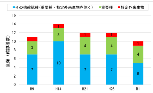
図 魚類の確認種数の経年変化(手取川ダム)
