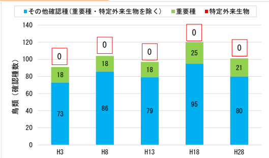
図 鳥類の確認種数の経年変化(手取川)
