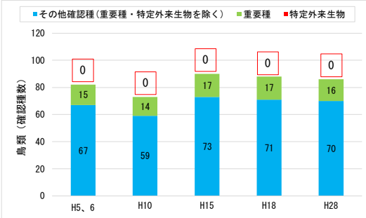
図 鳥類の確認種数の経年変化(手取川ダム)
