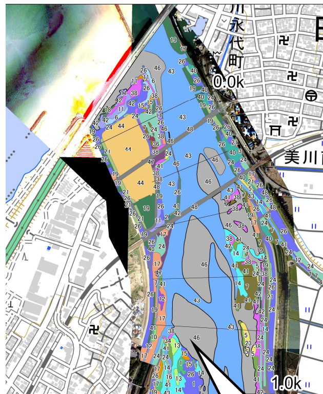
図 河口域の植生
