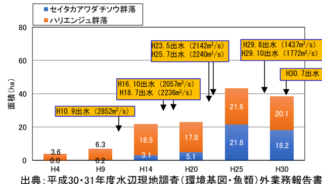
図 外来植物群落の経年変化(手取川)
