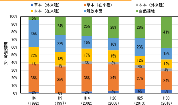
図 陸域の植生群落の経年変化(手取川)
