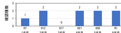
図 魚類(外来種)の経年変化(手取川)
