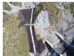
【山腹工】
