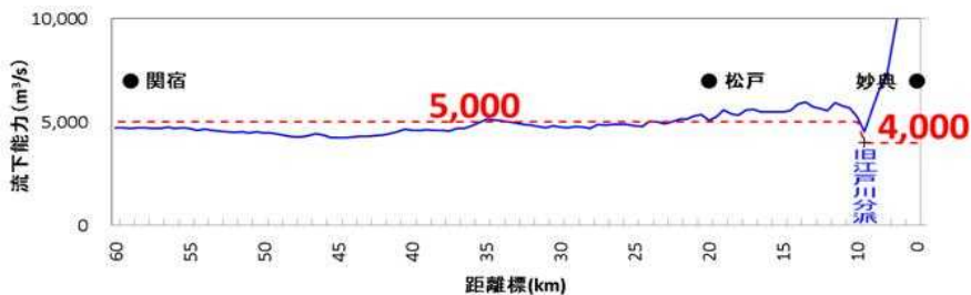
江戸川 流下能力図
