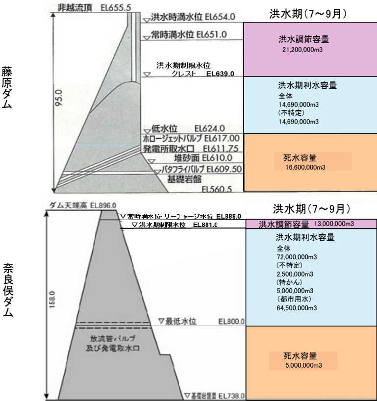
貯水池容量配分図（現行）
