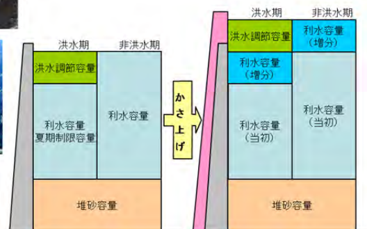
図 4.3-21 かさ上げイメージ図
