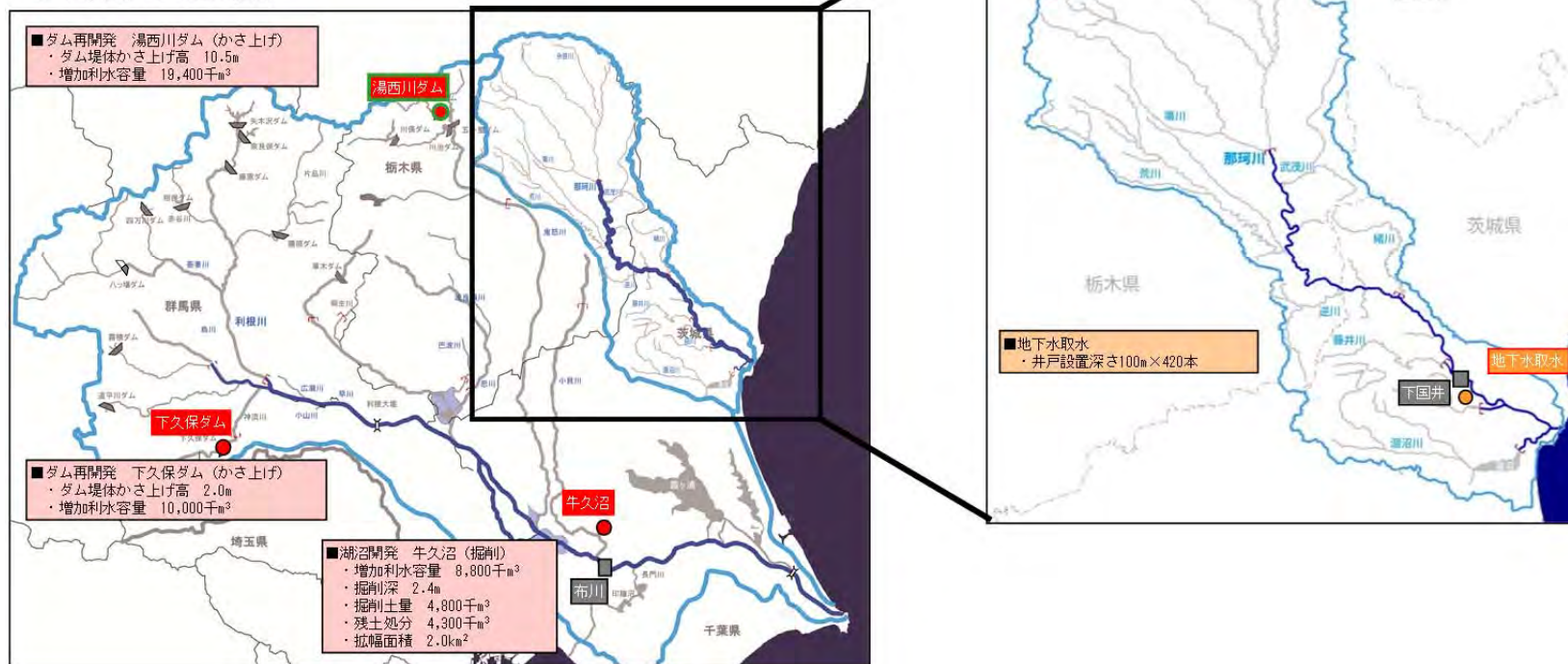
図 4.3-66 新規利水対策案の概要 ケース 5-2 那珂川における開発量を地下水取水により確保する新規利水対策案
