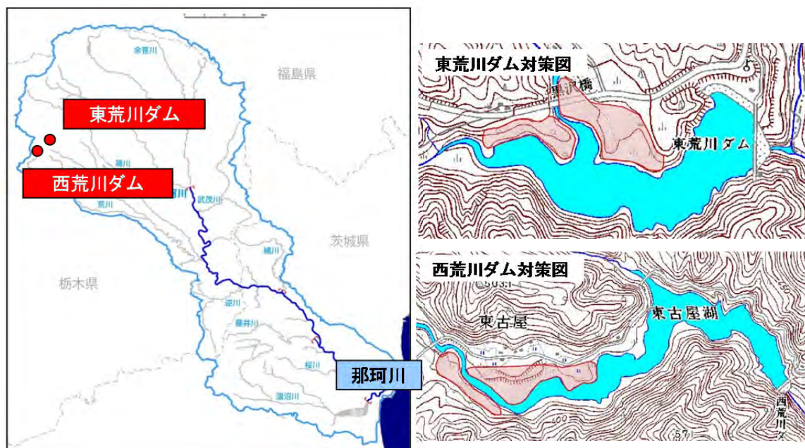
図 4.3-46 対象施設位置図等
