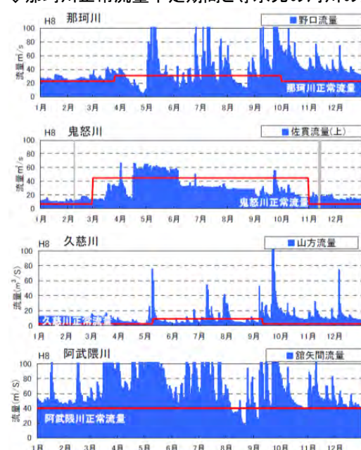
◇那珂川正常流量不足期間と導水元の河川の流況
