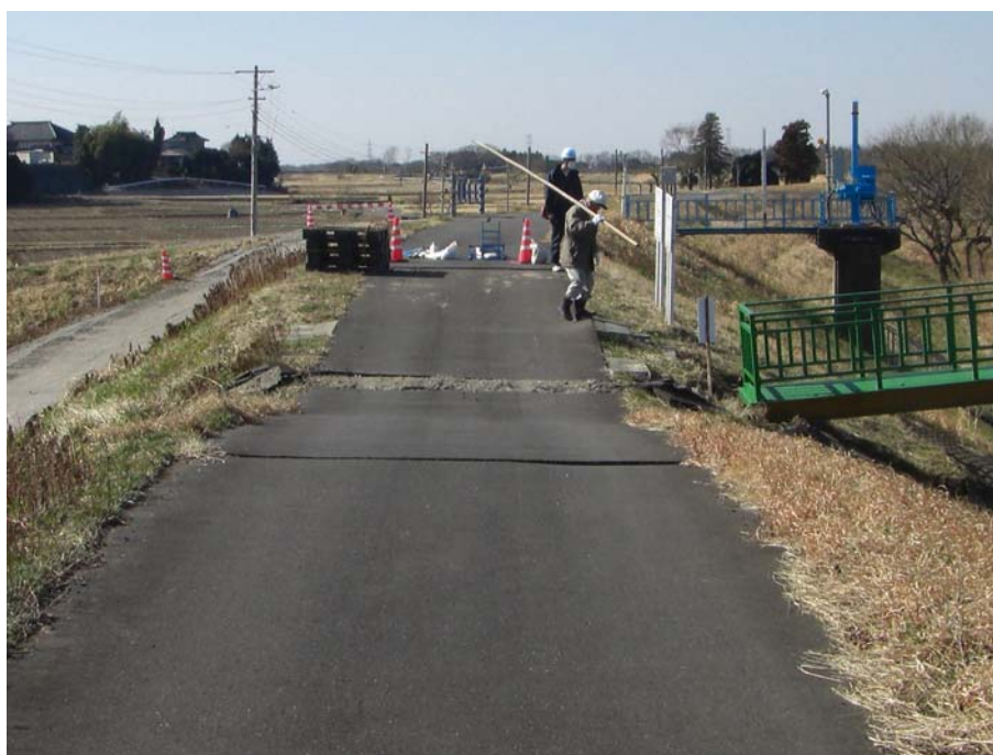
写真-24 天端の沈下と管理橋の落座
