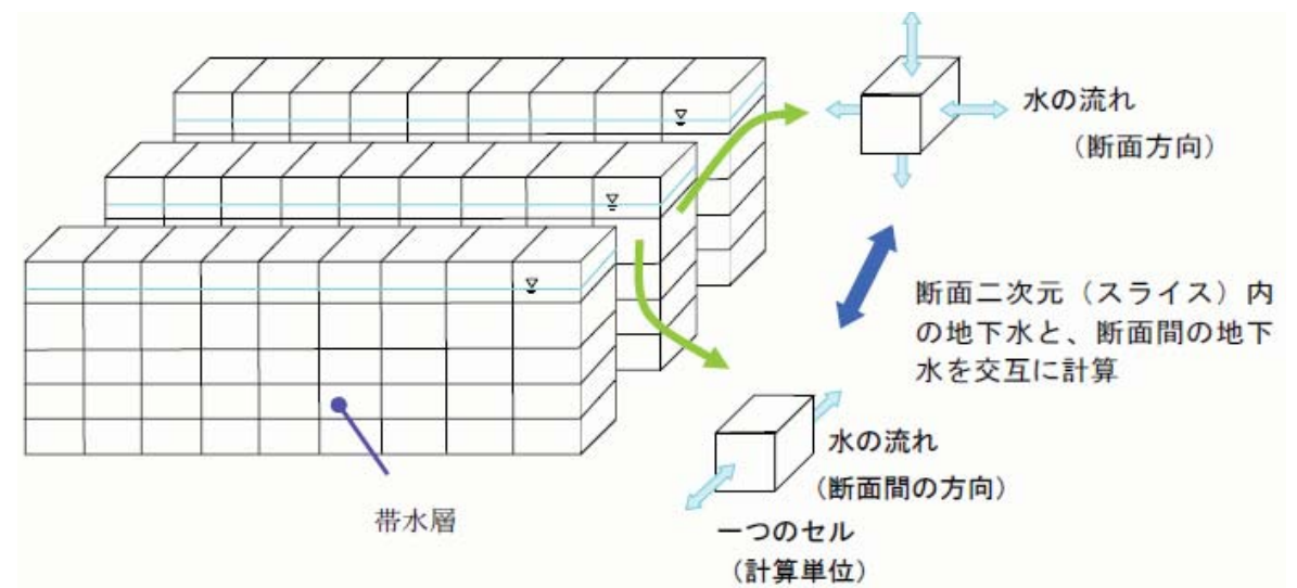
d 準三次元モデル③
