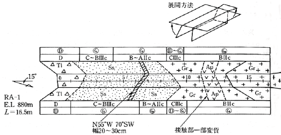
図 15-4-3 調査横坑展開図の例
