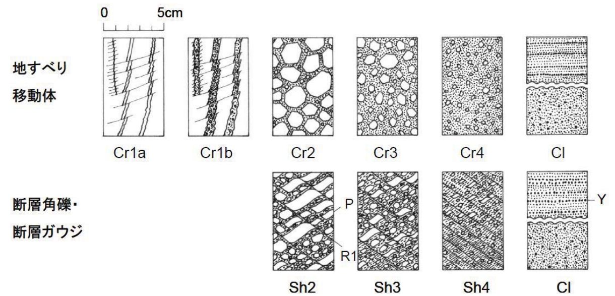
図15-4-4 地すべり移動体及び断層岩類の破碎度区分の例（脇坂・上妻・綿谷・豊口, 2012）
