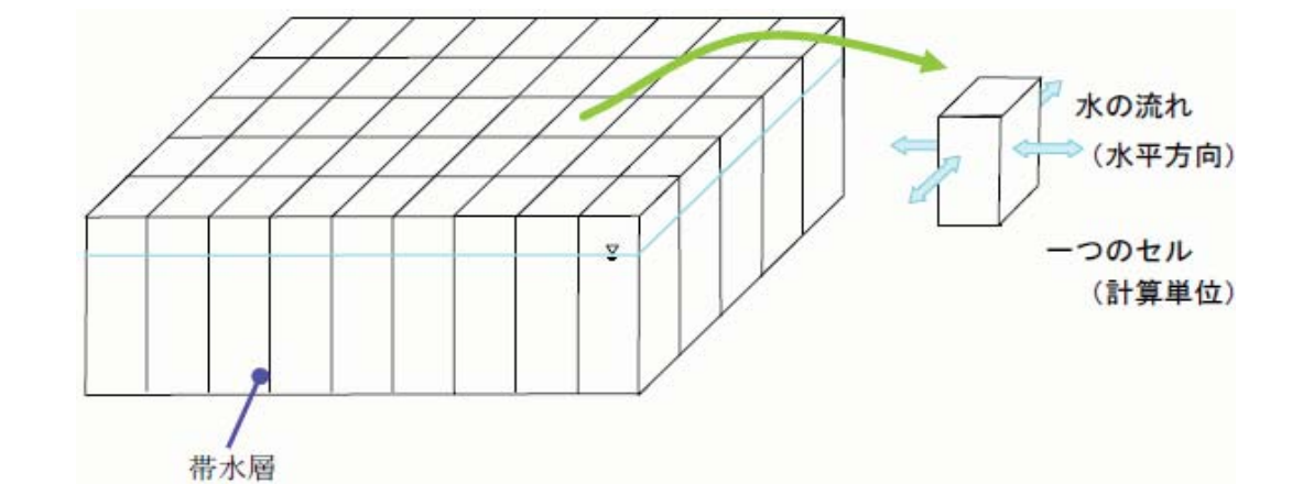
f 平面二次元モデル
