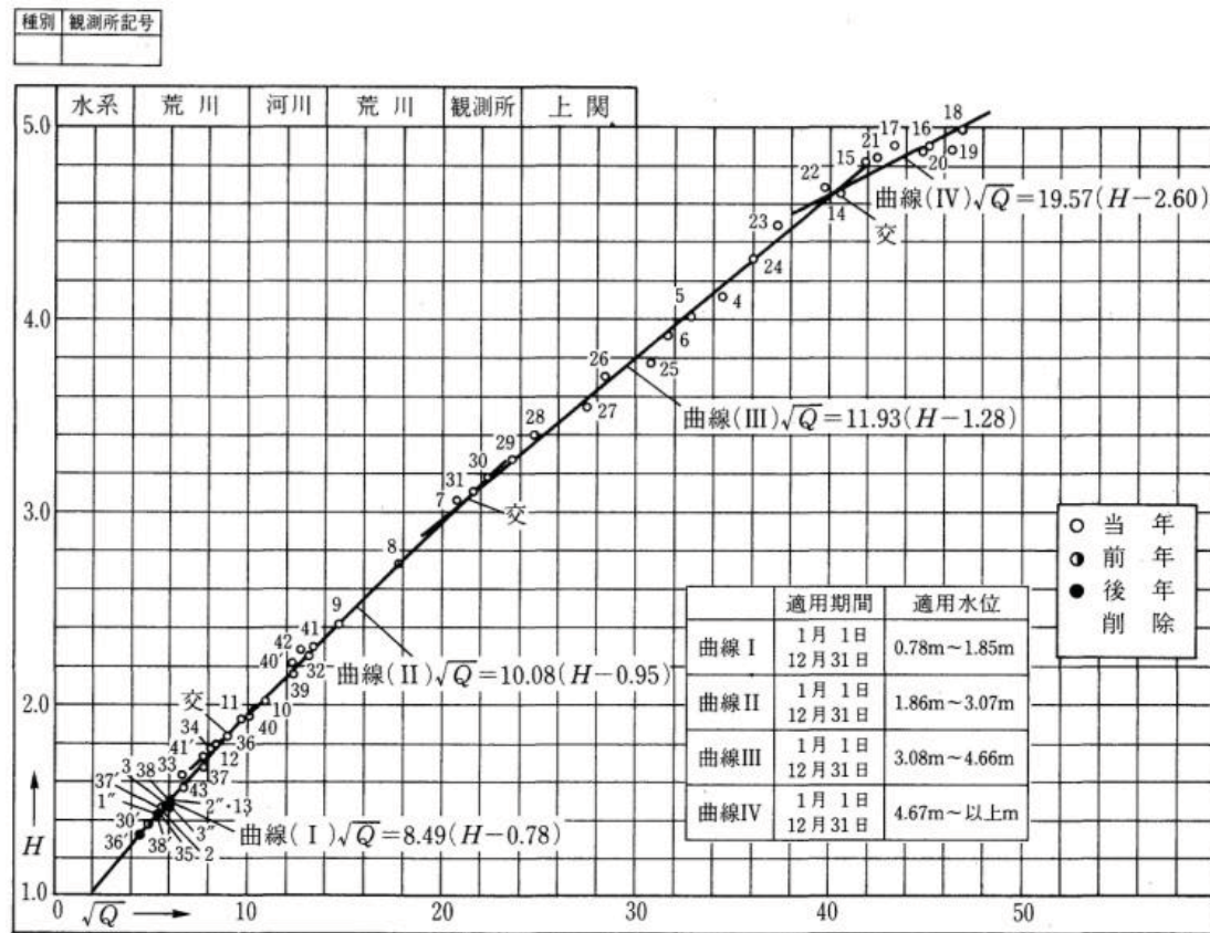
図 2-5-4 観測水位流量図 (H-√Q 図)
