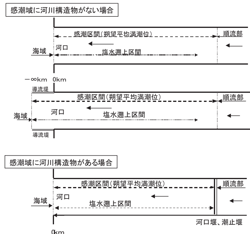
図 14-1-2 感潮区間及び塩水遡上区間
