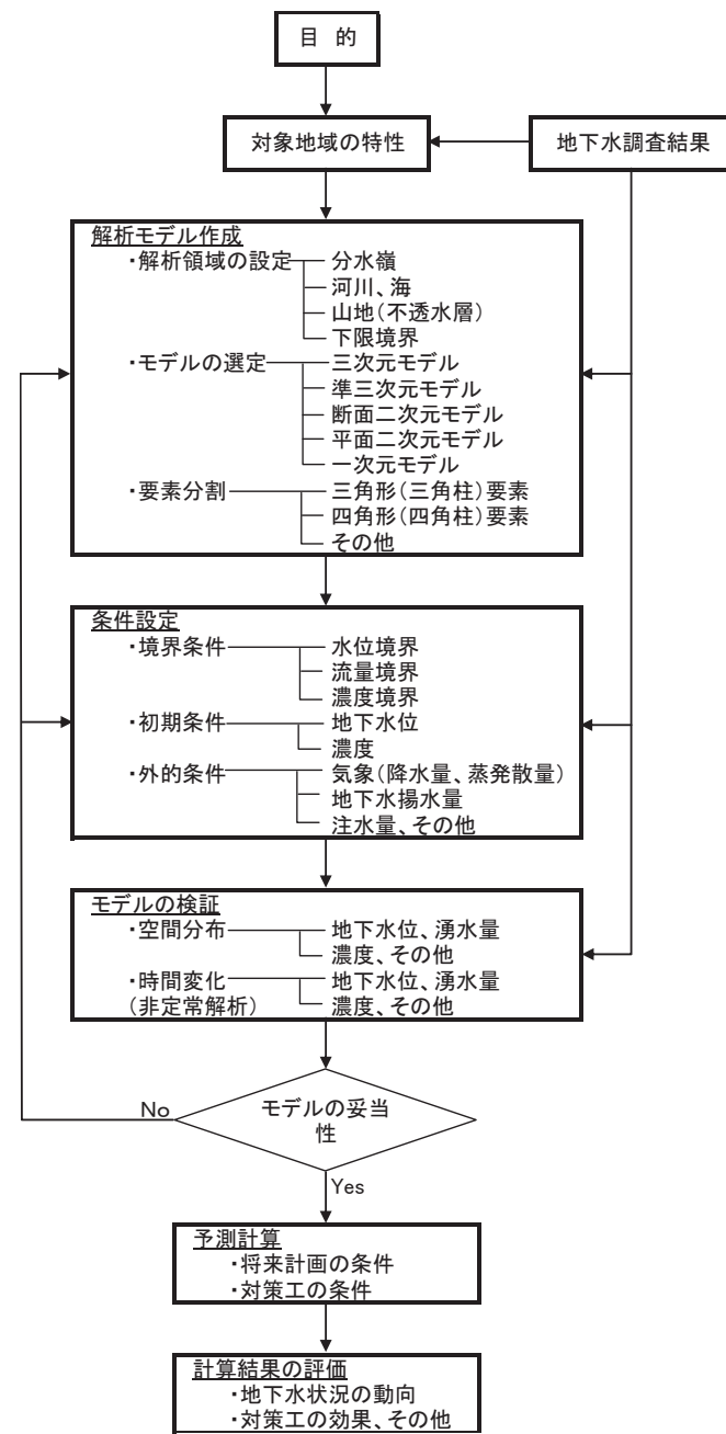
図 3-3-2 地下水流動解析の流れ (「地下水調査及び観測指針(案)」に加筆)
