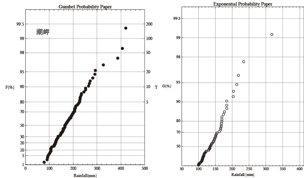
図 3-1-1 Gumbel 確率紙の事例 (極値資料)
