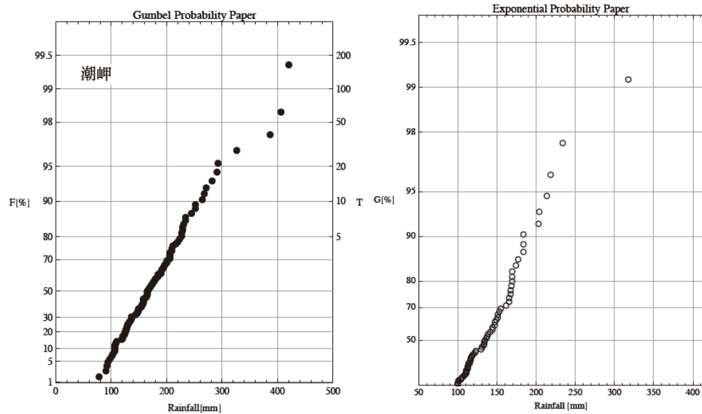
図 3-1-1 Gumbel 確率紙の事例 (極値資料)
