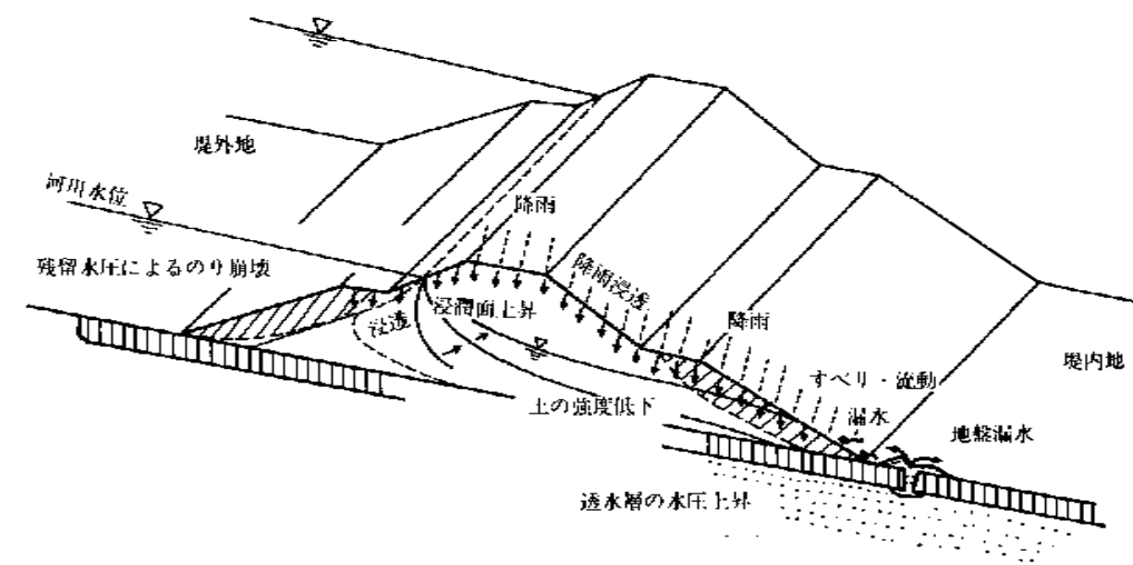
図 15-2-3 堤防への降雨、河川水の浸透と漏水
