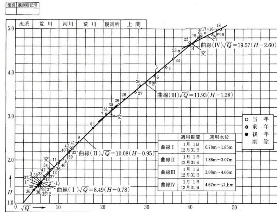
図 2-5-4 観測水位流量図 (H-√Q 図)
