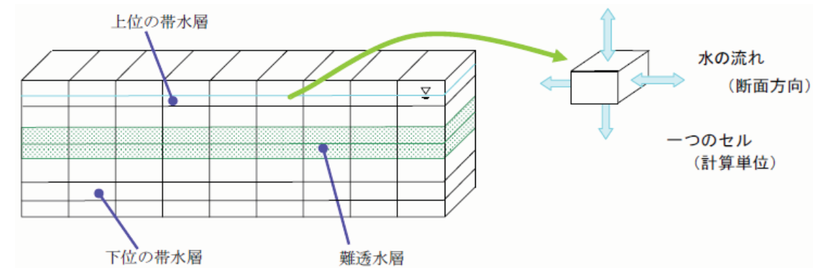
e 断面二次元モデル
