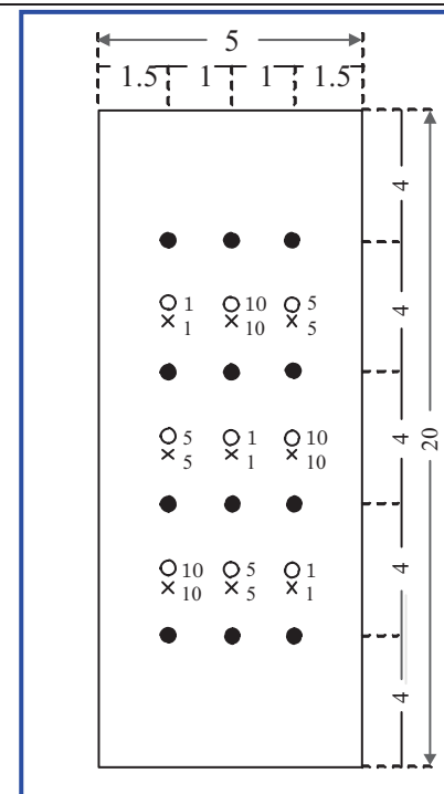
図 15-2-2 試験施工の測定項目と測点位配置の一例
