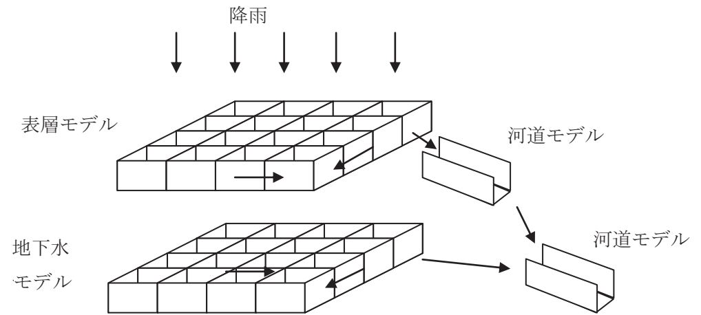
図 3-2-3 土研分布モデル Ver. 2 の構成図
