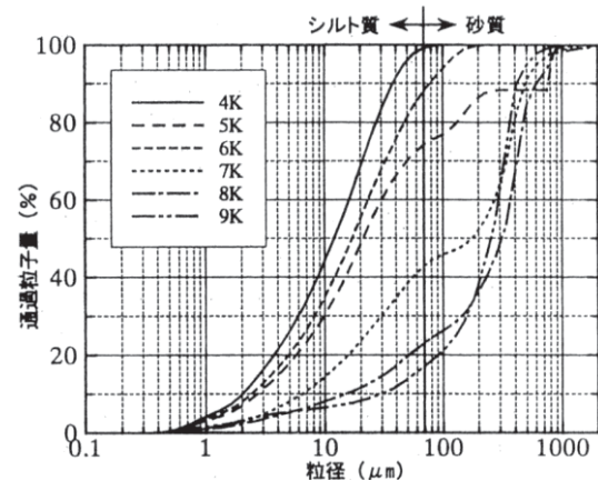
図14-2-3 粒度分布分析結果（4k～9k）
