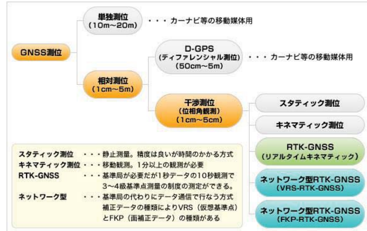
図 22-3-6 GNSS 測量/計測の方式の種類
