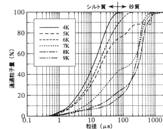
図14-2-3 粒度分布分析結果（4k～9k）
