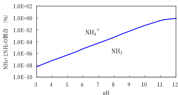
図 5.15 pH 値による \text{NH}_4^+ と \text{NH}_3 の割合変化 (25℃の場合)
