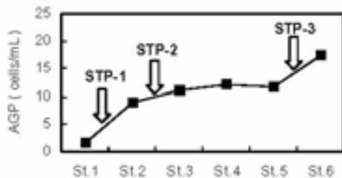
図 5.25 多摩川における AGP の変化
