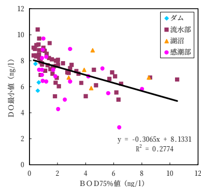
図 5.11 BOD(75%値)と D0(最小値)の関係
