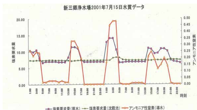
図 5.21 中江戸導水路運転時の新三郷浄水場における原水水質の状況
