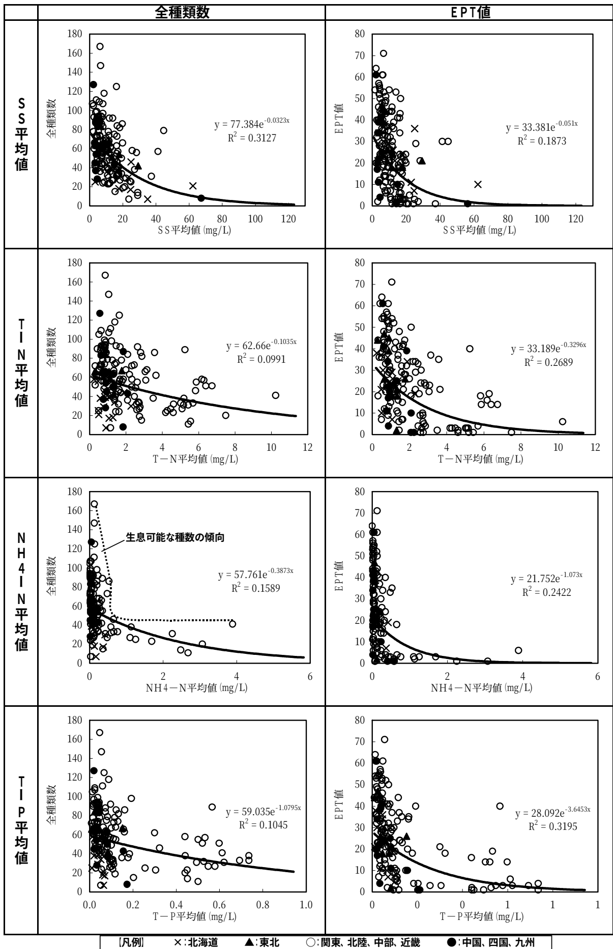
図 5.18 (2) 底生生物（全種数・EPT 値）と水質の関係
