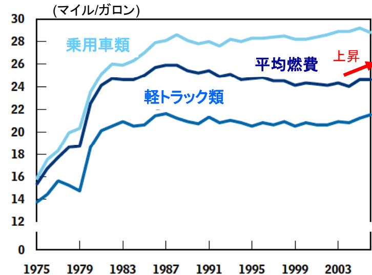
平均燃費効率の推移
