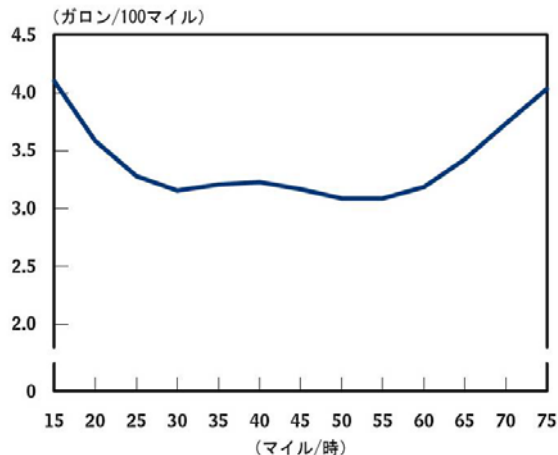
旅行速度と燃費の関係
