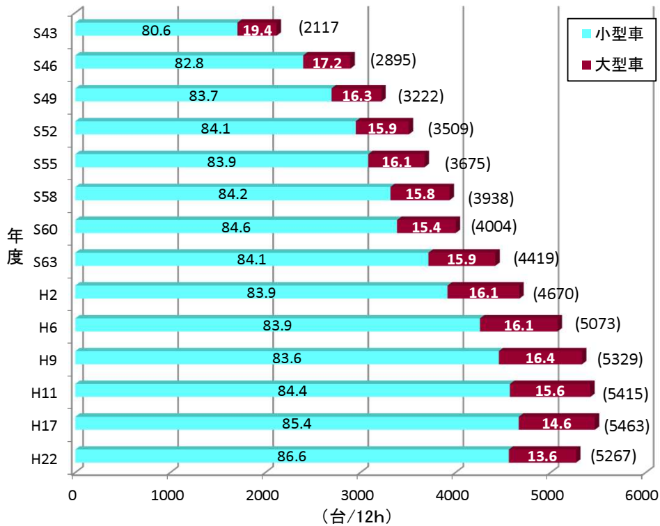
図1-1 車種別12時間平均交通量の推移〔一般道路計〕
