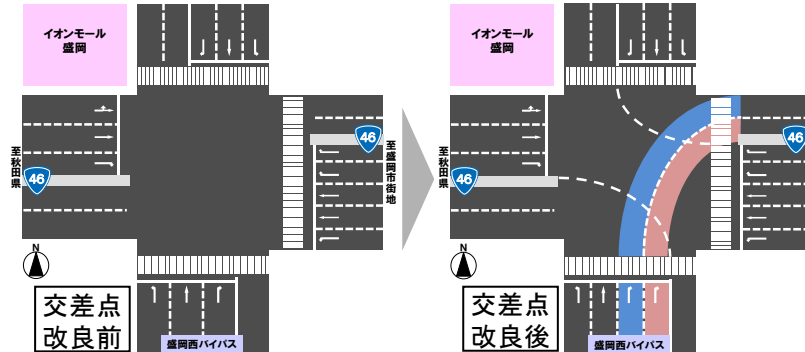
一般国道46号 前潟交差点
