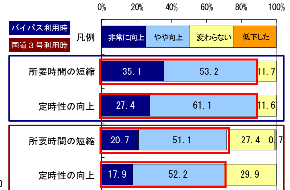
▲交通円滑化の実感(住民アンケートより)
