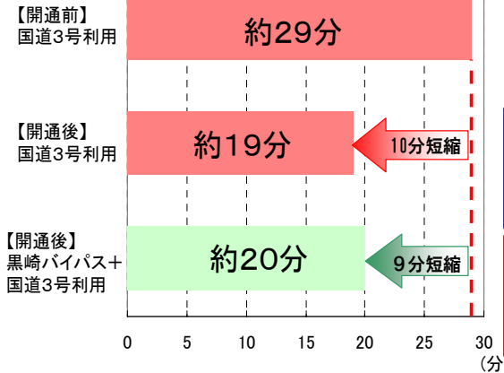
▲樋口町～西本町1丁目交差点 所要時間の変化
