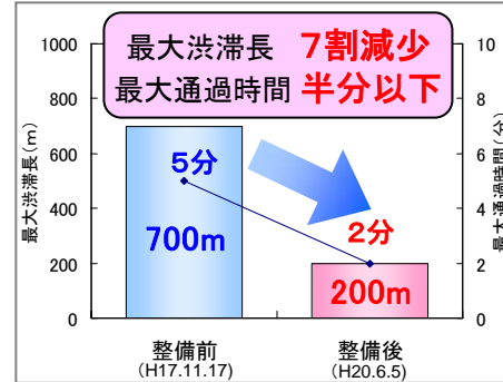
▲最大渋滞長、通過時間の変化 (渋滞調査結果)
