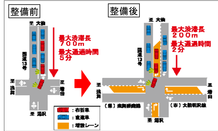
▼大橋交差点の渋滞状況の変化
