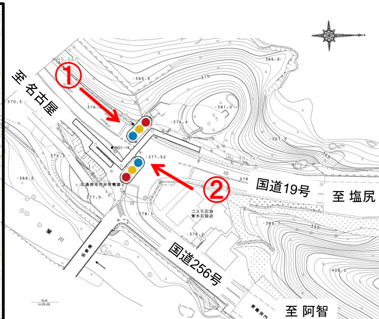
平面図
