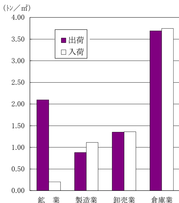
図 3 - 1 - 20 産業別事業所敷地面積 1 m 2 当たり年間出入荷量
