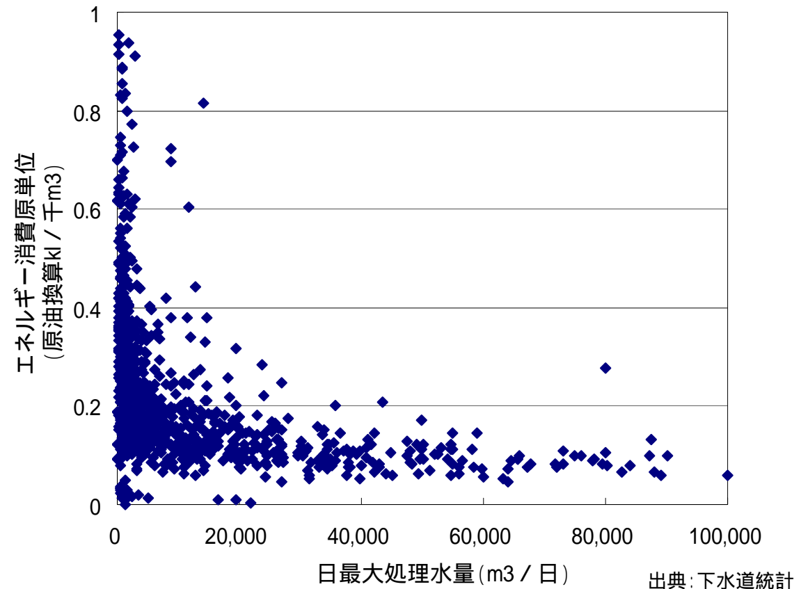
下水処理場のエネルギー消費原単位
