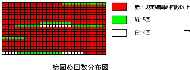
締固め回数分布図
