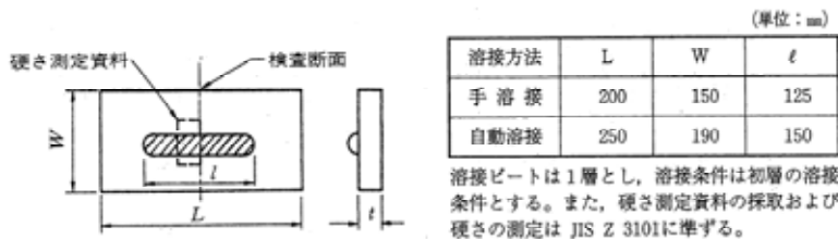
図3 - 4 最高硬さ試験, 試験体形状および試験片採取位置
