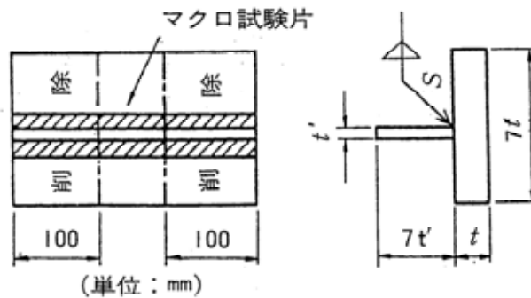
図3 - 3 すみ肉溶接試験, 試験体形状および試験片採取位置
