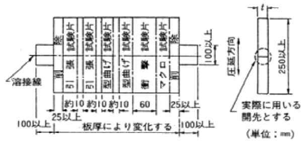
図3 - 1 突合せ溶接試験, 試験体形状および試験片採取位置
