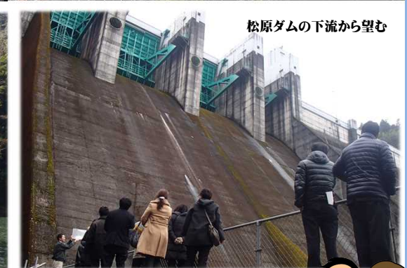
松原ダム
