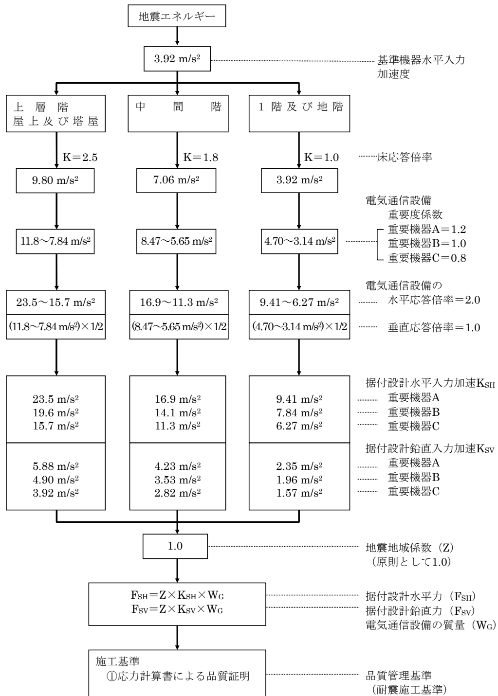
図3-3-1 電気通信設備の耐震据付設計基準の考え方
