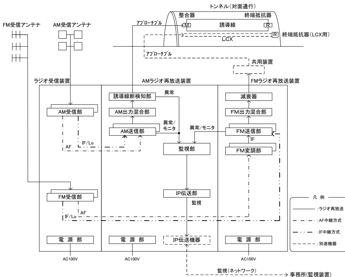
トンネル内ラジオ再放送設備 概念図
