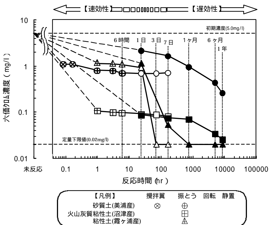
図-4.5 六価クロム濃度の変化
