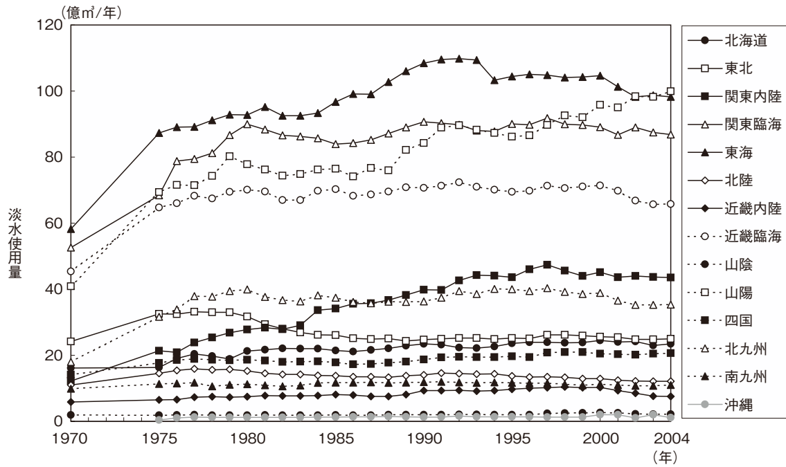
図4-1-3 地域別工業用水淡水使用量の推移
