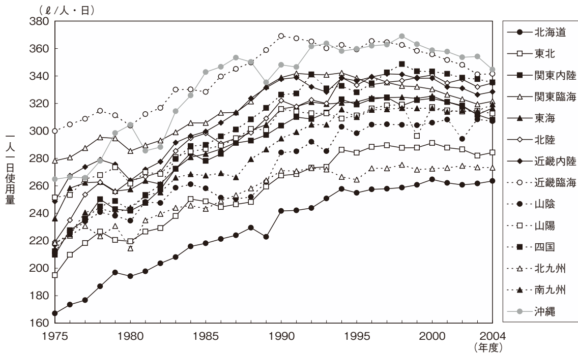
図4-1-2 生活水の一人一日使用量の推移（地域別）（有効水量ベース）
