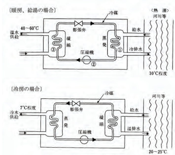
図 ヒートポンプによる熱利用の例
