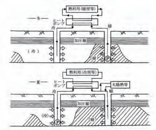
図2 地下水の熱利用システムの例
