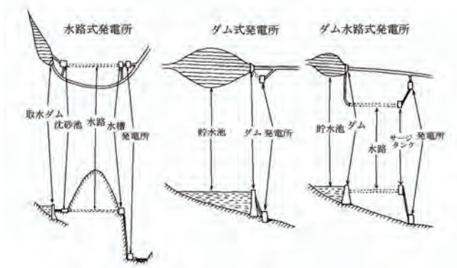
図 一般水力発電所の構造
