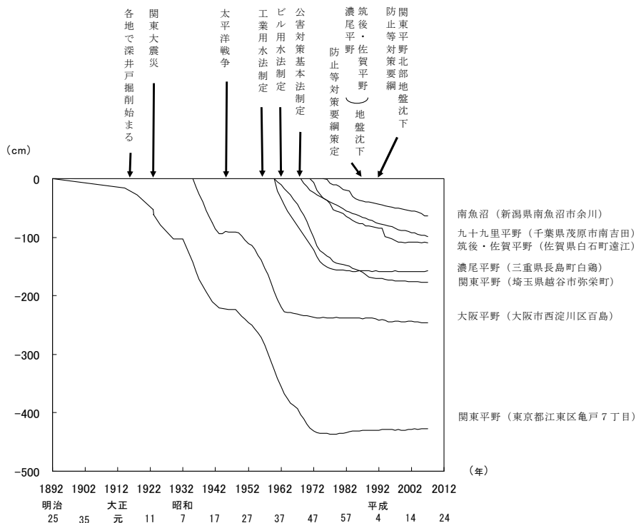
図7-1-1 代表的地域の地盤沈下の経年変化
