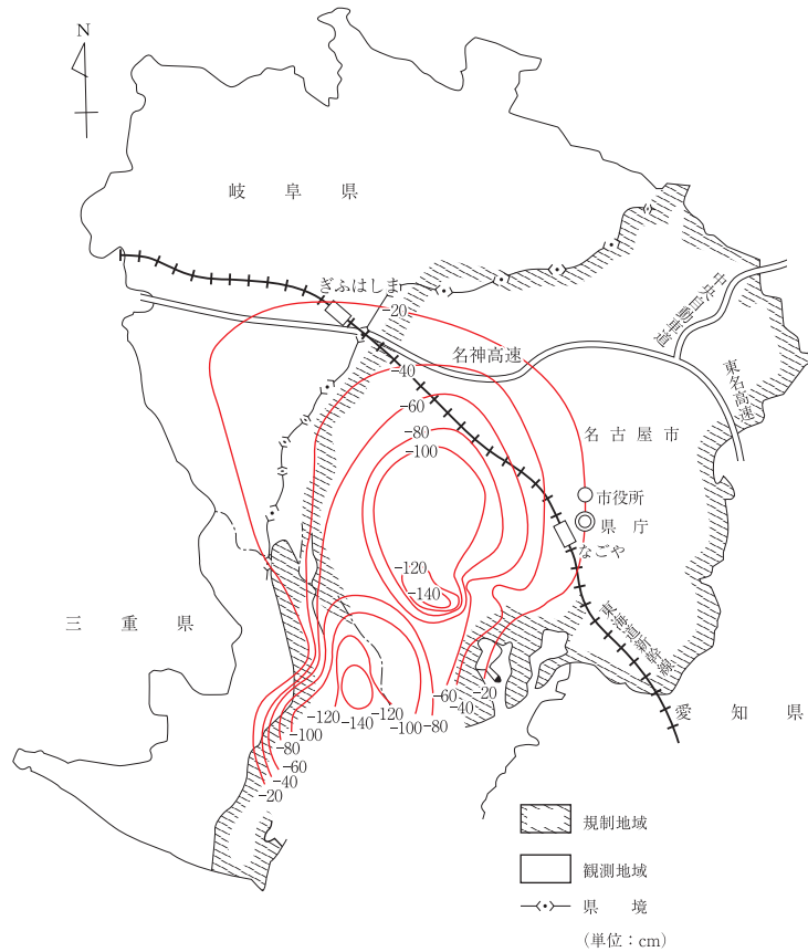
図7-2-1 濃尾平野地盤沈下防止等対策要綱対象地域及び累積沈下量 (昭和36年2月～平成19年11月)
