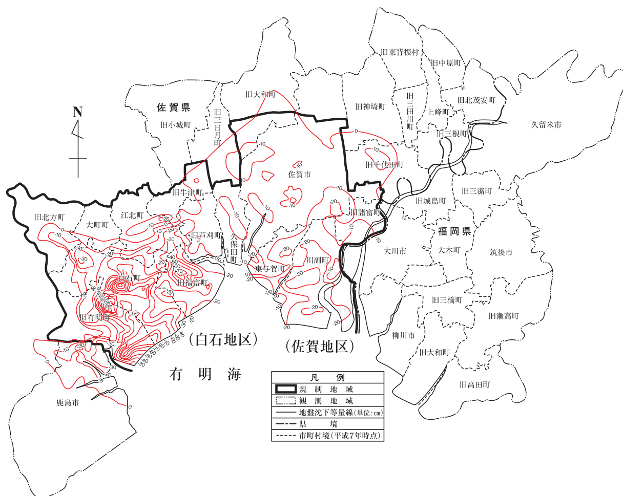
図7-2-3 筑後・佐賀平野地盤沈下防止等対策要綱対象地域及び累積沈下量 (昭和47年2月～平成20年2月)
