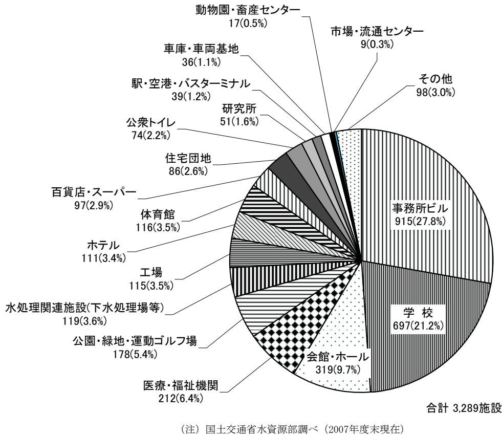
図8-1-4 建物用途別 雨水・再生水利用施設数
