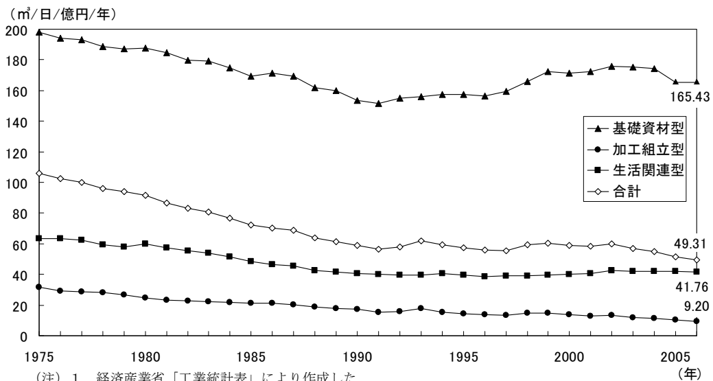
図 8-1-6 工業用使用水量原単位の推移
