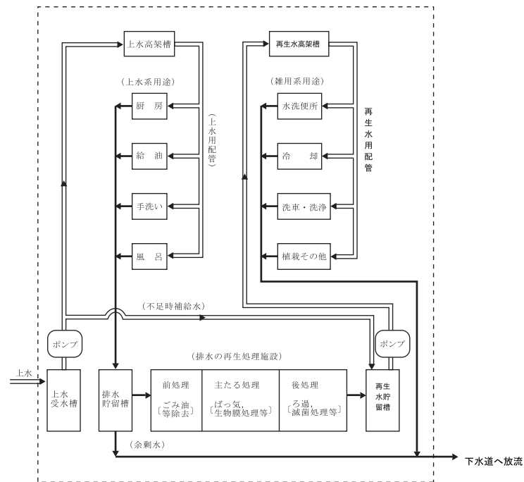
図8-1-2 再生水利用のシステム例
