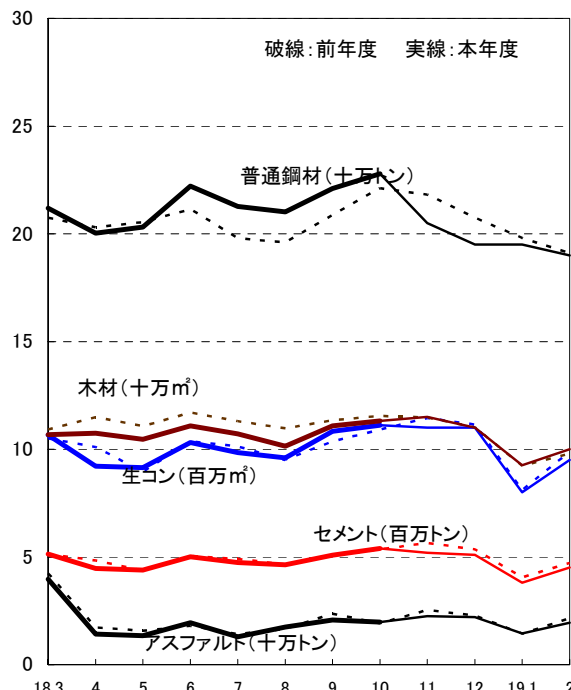
主要建設資材需要量の推移
