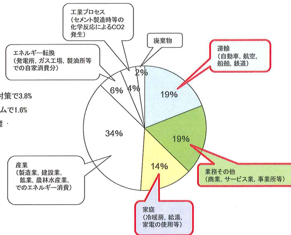
二酸化炭素排出量の部門別内訳
