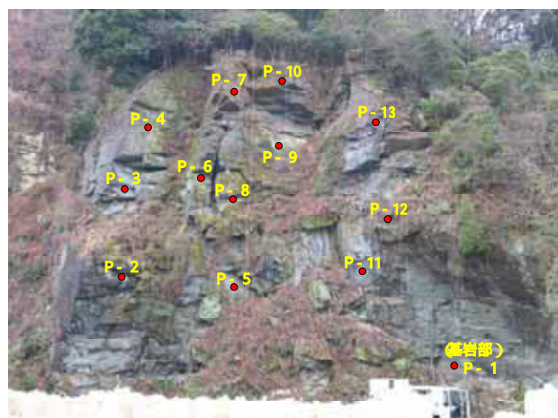
図 - 4 計測対象斜面及び計測点配置
