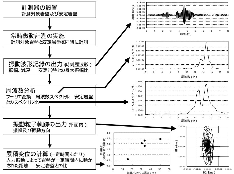
図 - 3 解析処理の流れ
