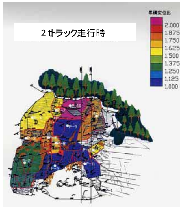
図 - 6 累積変位比分布図
