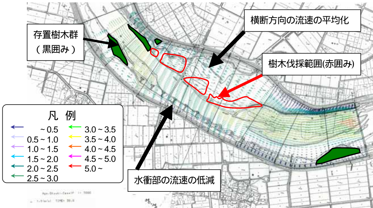
図 4 . 1 . 3 樹木伐採後の平面流況 (阿賀野川水系阿賀川)
