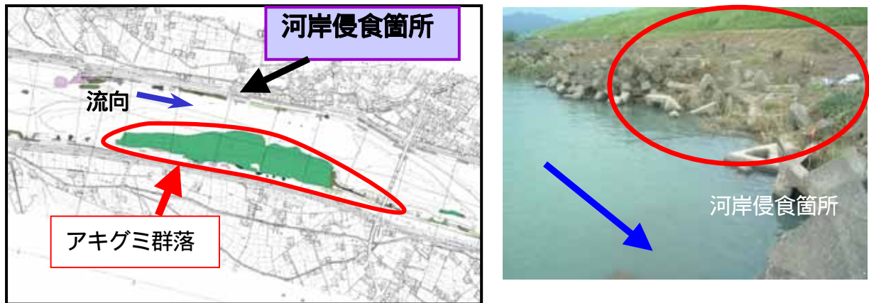
図4.2.2 河道内樹木群による河岸侵食の誘発（那賀川水系那賀川）
