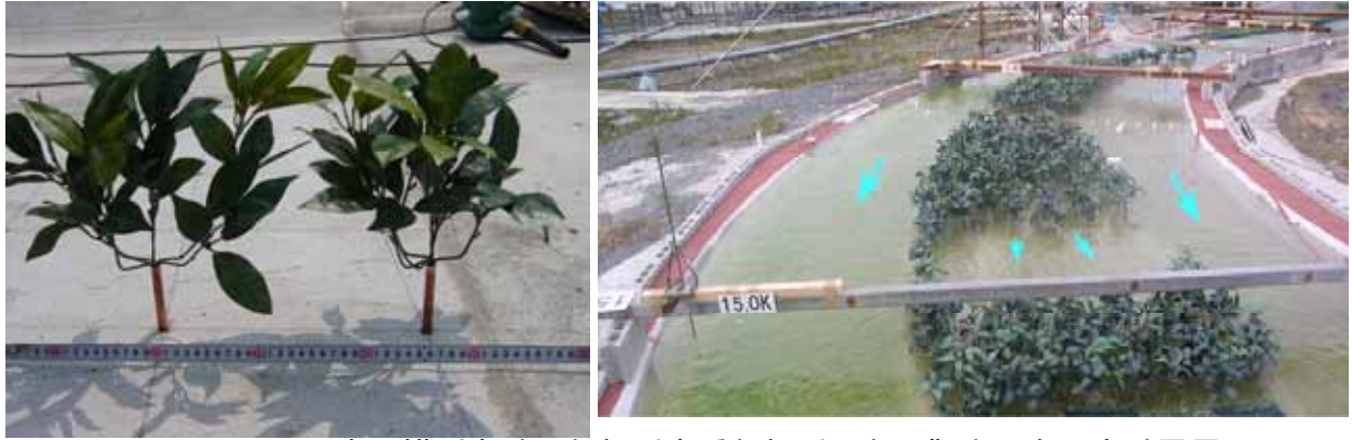
図4.1.5 水理模型実験（矢部川水系矢部川 左：擬木 右：実験風景）
