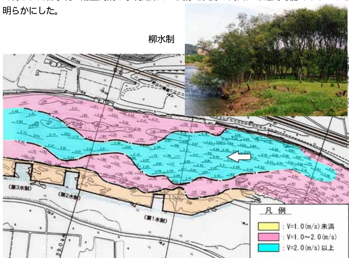
図4.1.2 出水時の空撮による流速ベクトル解析図と柳水制(米代川水系米代川)
