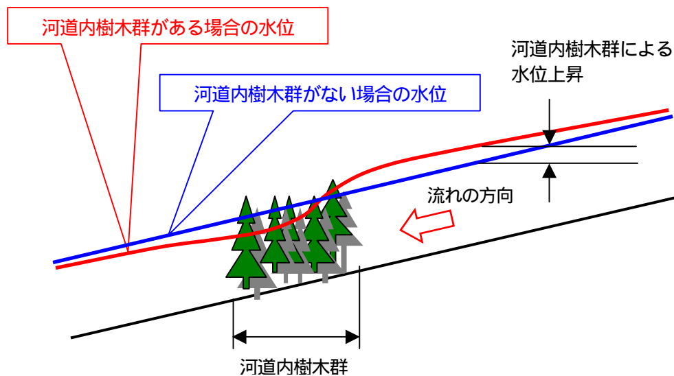
図 4 . 1 . 4 樹木群の水位への影響の概念図 (江の川水系江の川)
