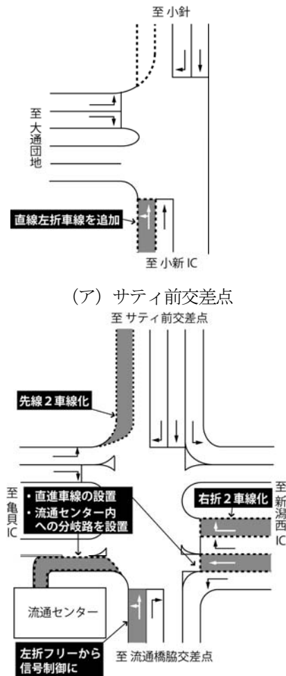
（イ）小新IC交差点 図－6 改良計画（イメージ）
