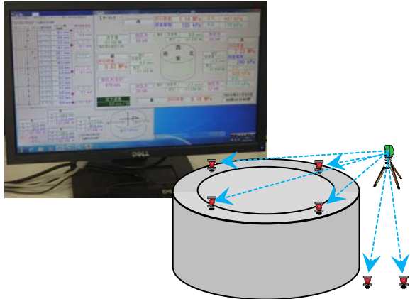
図-2 ケーソン沈下管理システム（ICT）
