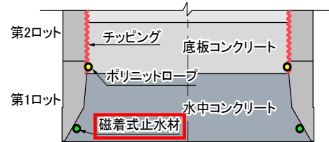
図-4 磁着式止水材
