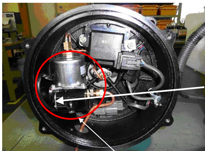
燃料ポンプ
