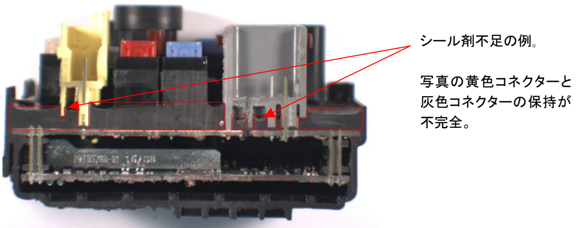
拡大断面図
