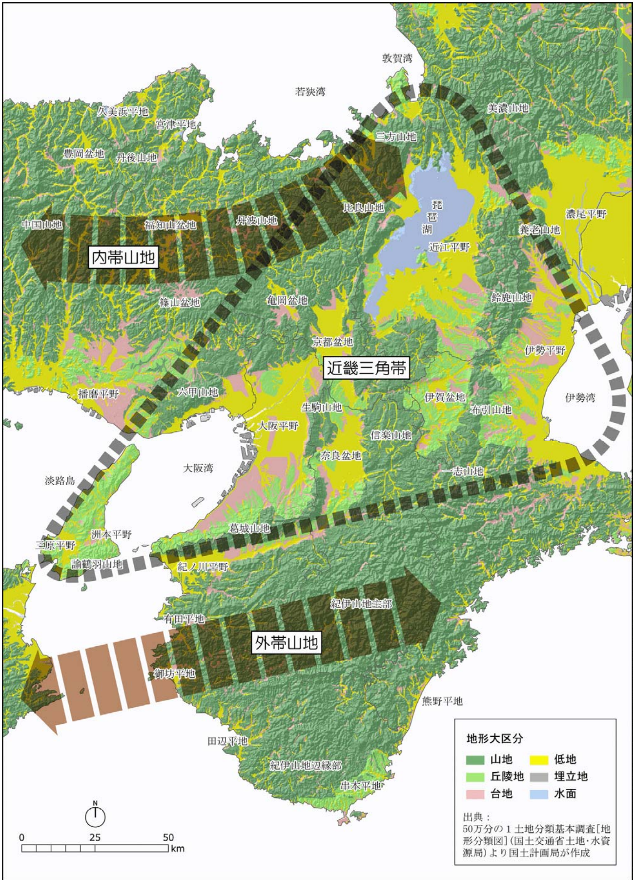
図エラー！ 指定したスタイルは使われていません。-1：地形大区分
