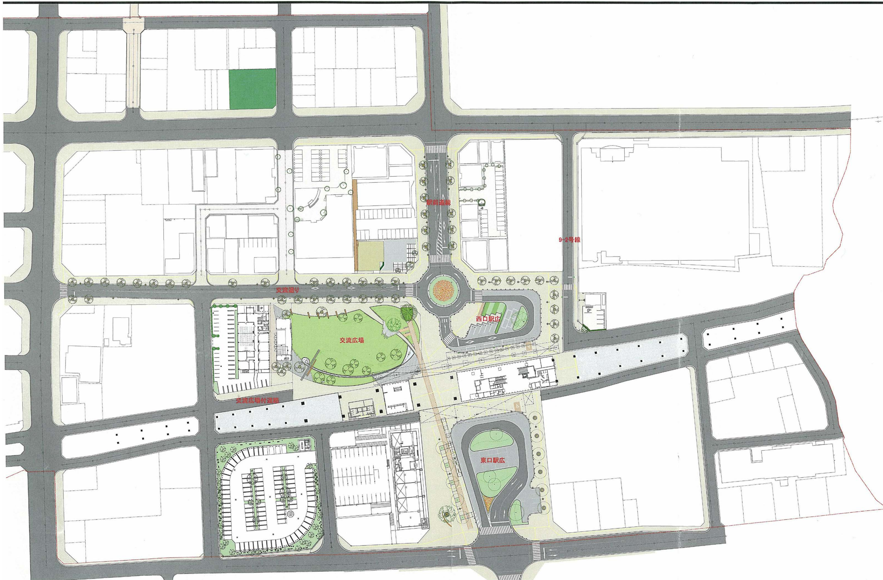
図 駅前広場及び広場計画平面図
