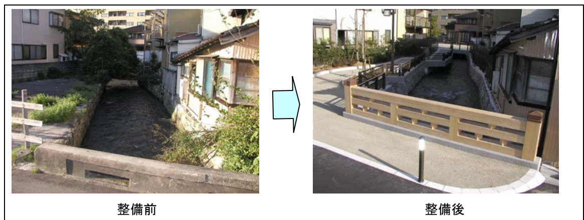
写－４５ 歴史的なまちなみにあわせた橋および歩道の整備
