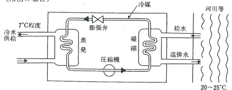
図 ヒートポンプによる熱利用の例
