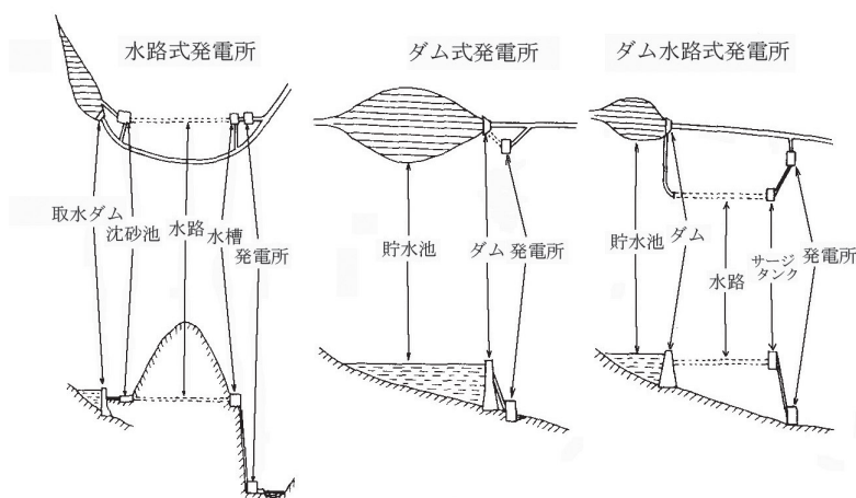
図 一般水力発電所の構造
