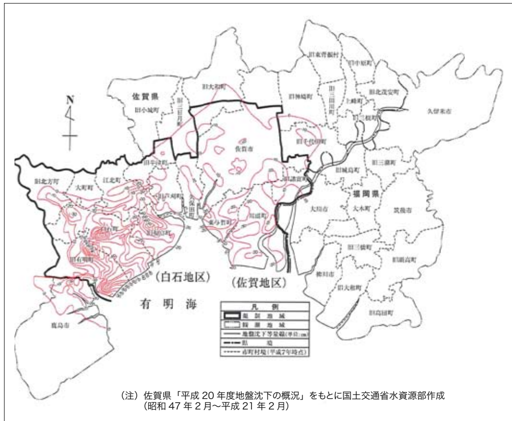
図4-2-3 筑後・佐賀平野地盤沈下防止等対策要綱対象地域及び累積沈下量
