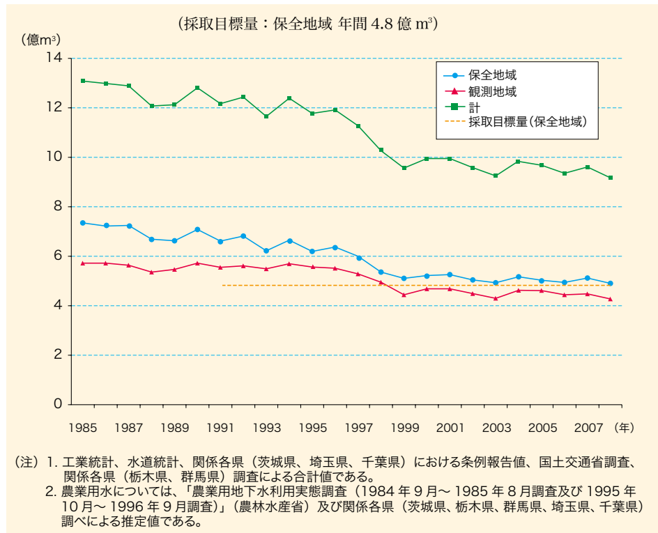
図4-2-6 関東平野北部地下水採取量の推移
