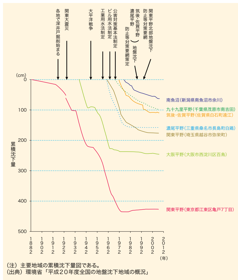
図4-1-1 代表的地域の地盤沈下の経年変化
