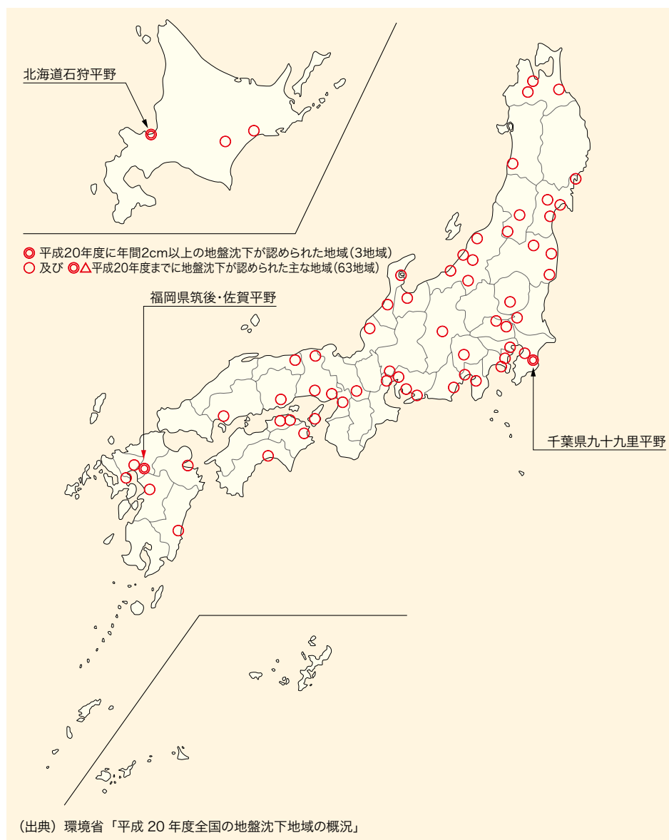
図4-1-2 平成 20 年度の全国の地盤沈下の状況
