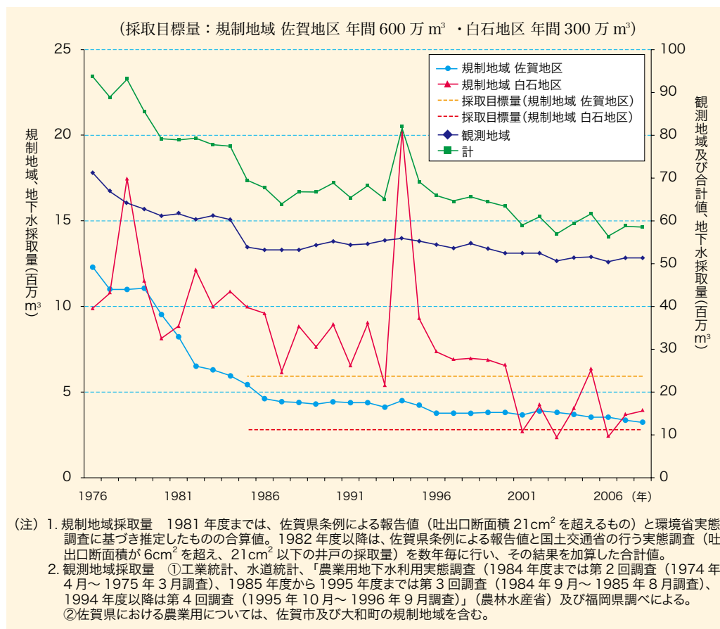
図4-2-4 筑後・佐賀平野地下水採取量の推移
