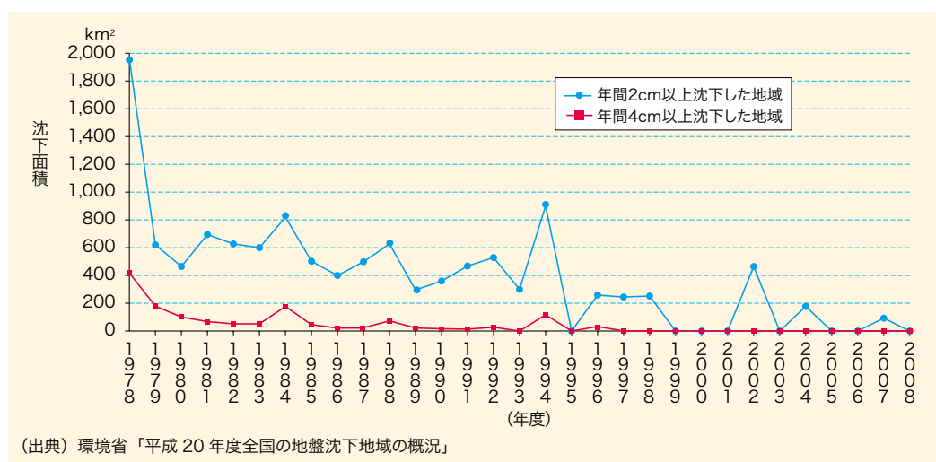
図4-1-3 全国の地盤沈下面積（年度別推移）
