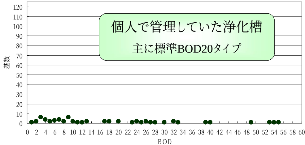
市管理浄化槽【寄付】の検査結果分布
