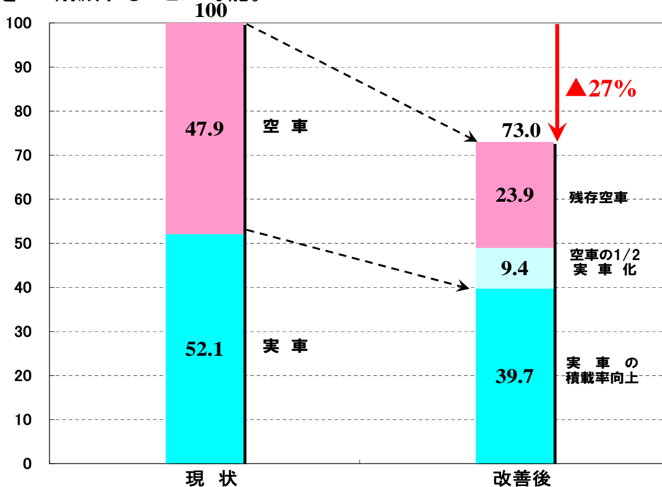
図 ロードファクター改善前後のエネルギー消費量の比較(現状=100)
